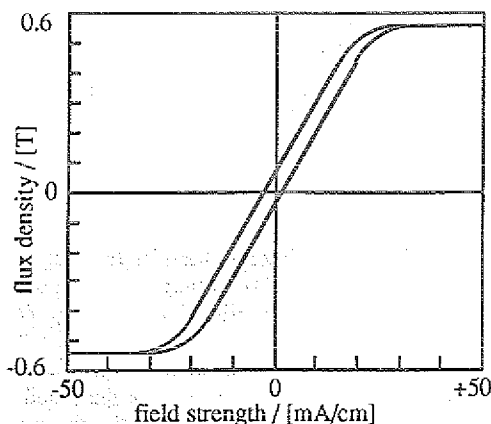
Fig. 6: VitroVac 6025F hysteresis
