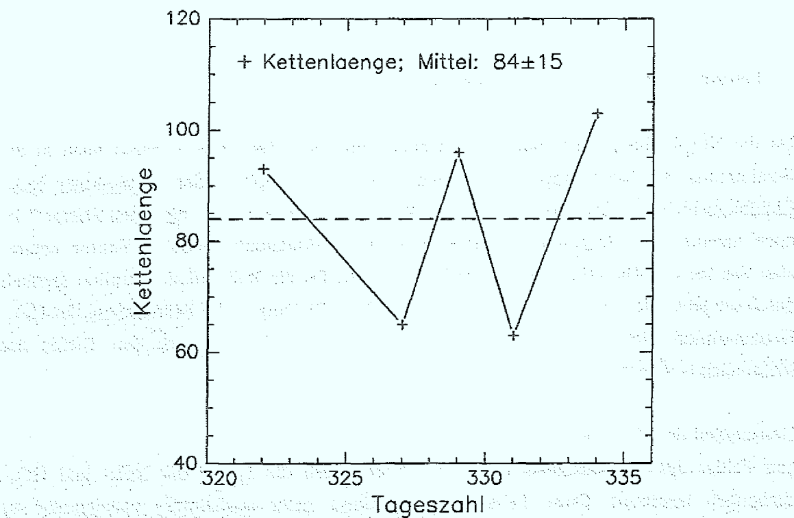
Abb. 5.4: Darstellung der Kettenlänge im Verlauf der Meßkampagne.
