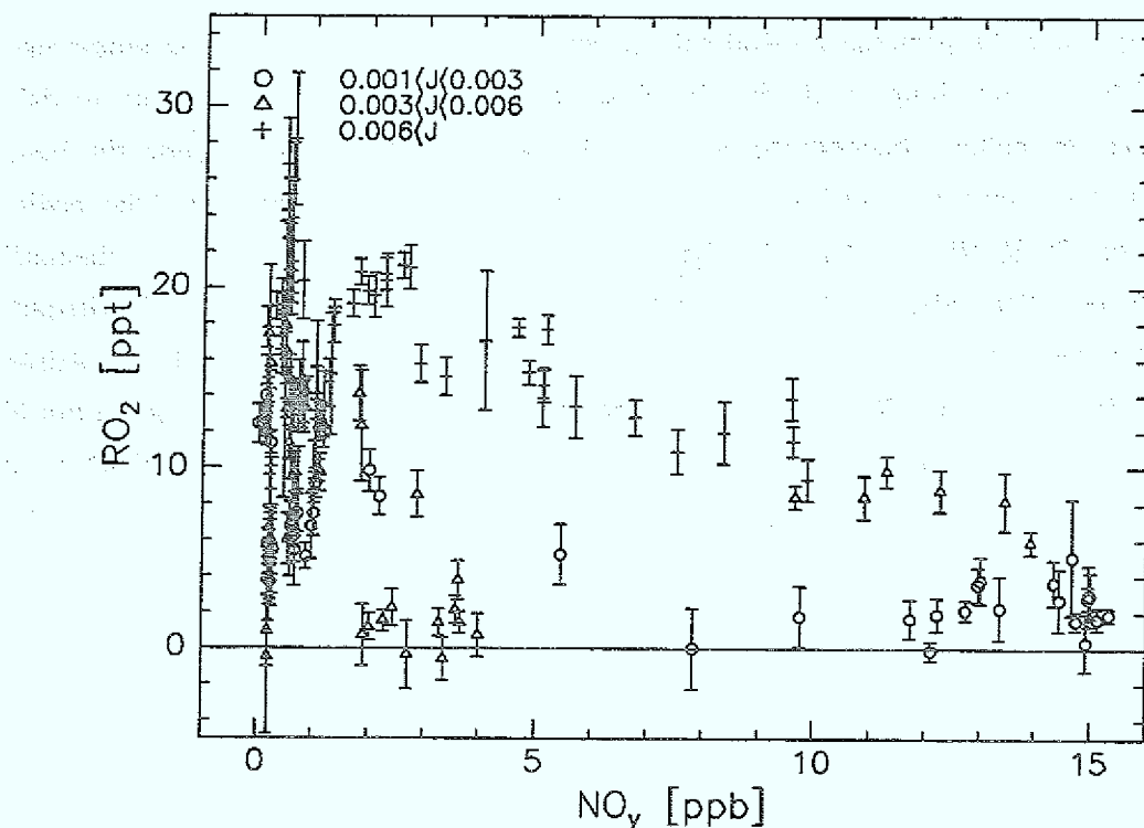
Abb. 6.4: Auftragung von RO_2 gegen NO_y^* . Bei starker Strahlung scheinen die Werte zunächst ein Maximum zu durchlaufen, um aber oberhalb von ca. 5 ppb NO_y^* unabhängig von der NO_y^* -Konzentration zu sein.
