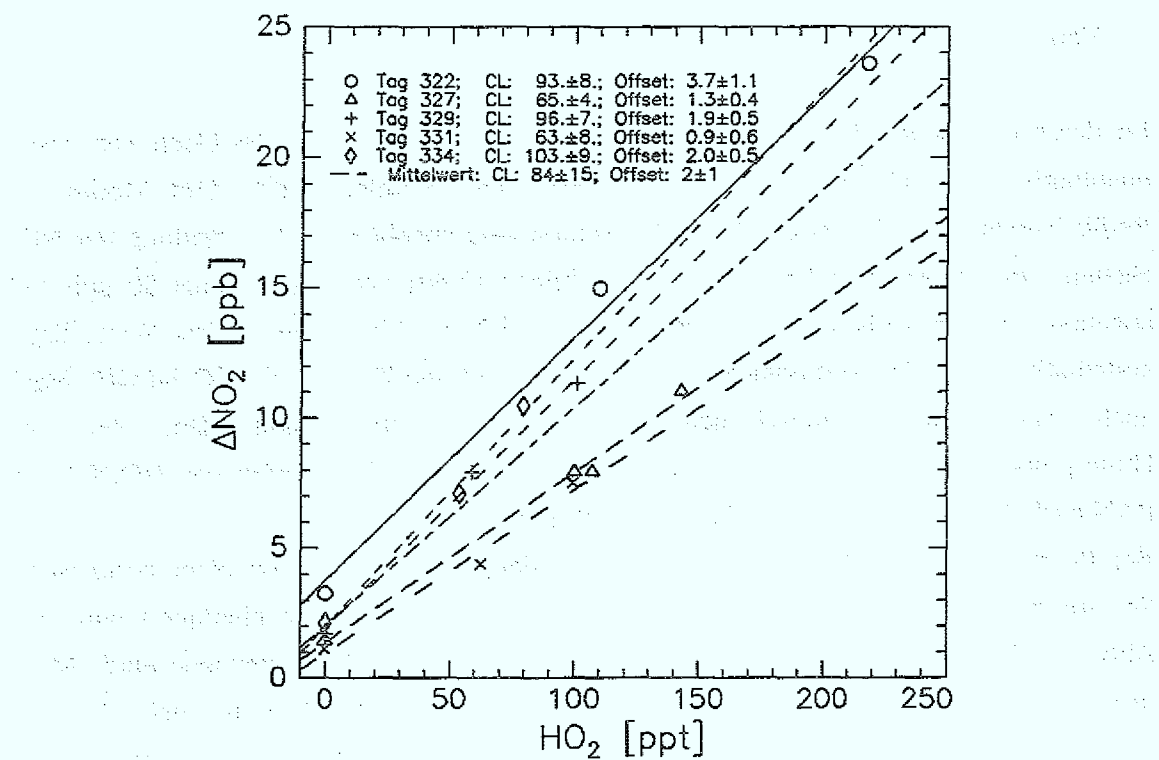
Abb. 5.3: Darstellung der Eichpunkte der Radikaleichungen auf dem Schauinsland. Die theoretisch berechneten Werte wurden entsprechend der Vergleichsmessung mit MIESR korrigiert (vgl. Kap. 4.5.2).
