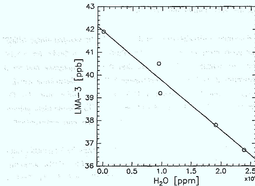
Abb. 4.6: Einfluß von Feuchte auf den NO 2 -Nachweis. Die Empfindlichkeit des Gerätes nimmt mit steigender Feuchte ab.
