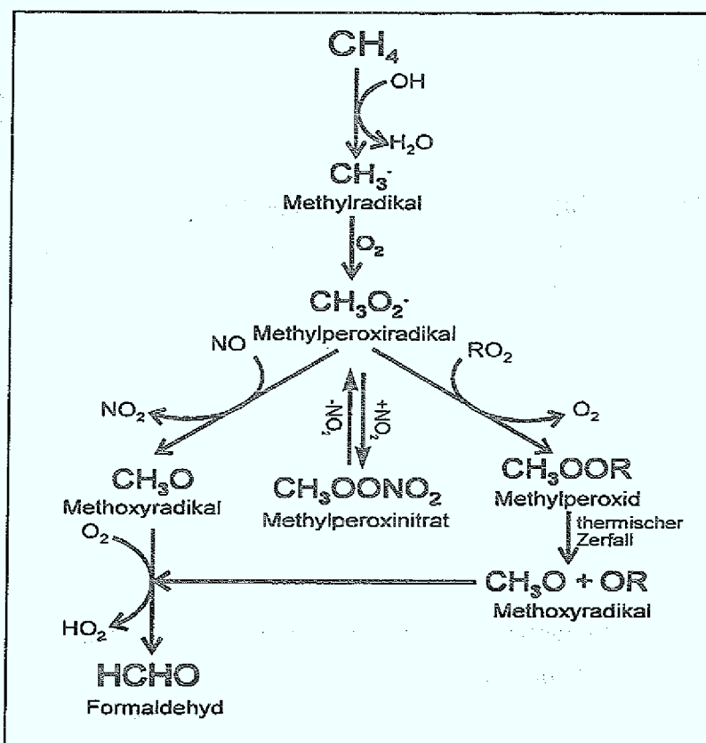
Abb. 2.2: Abbauwege von Methan initiiert durch das Hydroxylradikal.
