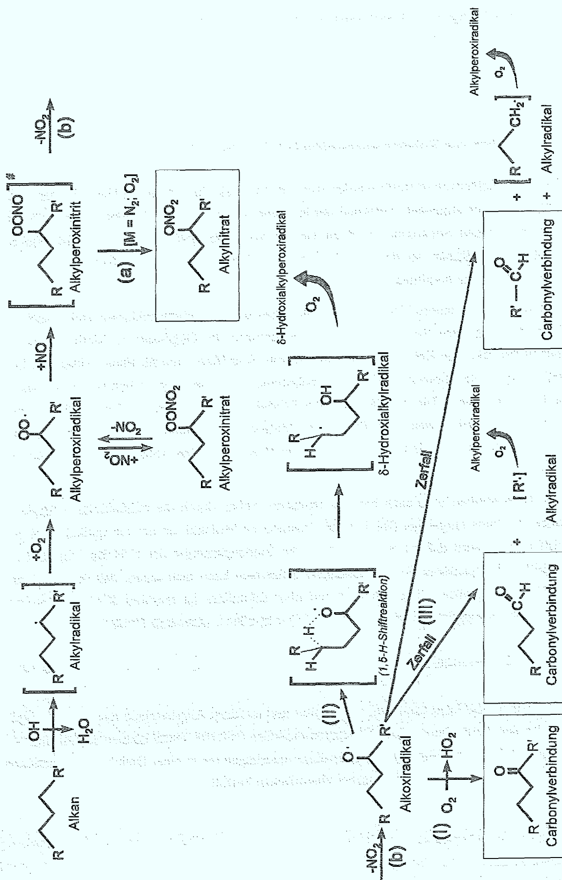
Abb. 2.3: OH-initiiertes, oxidatives Abbau von höheren Alkanen in der Atmosphäre.
