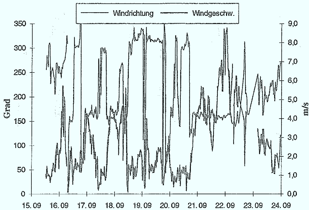
Abb. 4.34: Wie 4.32, jedoch für Windgeschwindigkeit und Windrichtung.
