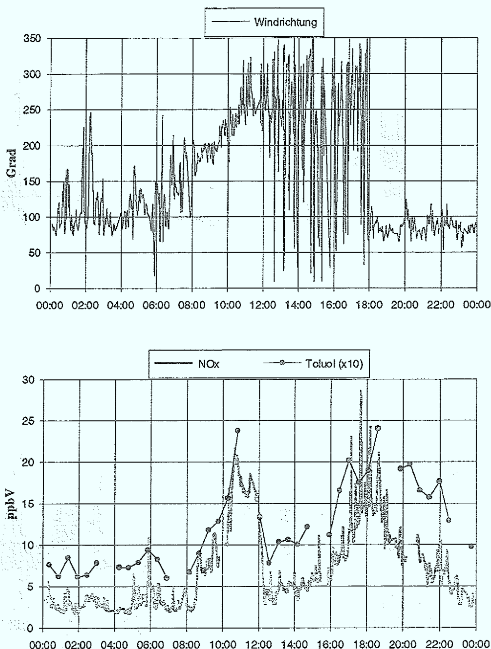
Abb. 4.36: Windrichtungsabhängigkeit der Schadstoffkonzentrationen in Kappel am Sonntag, den 20.9. Die NO x -Konzentrationen und Windrichtungsangaben sind Minutenmittelwerte. Die Toluolkonzentrationen (Halbstundenmittelwerte) wurden mit 10 multipliziert.
