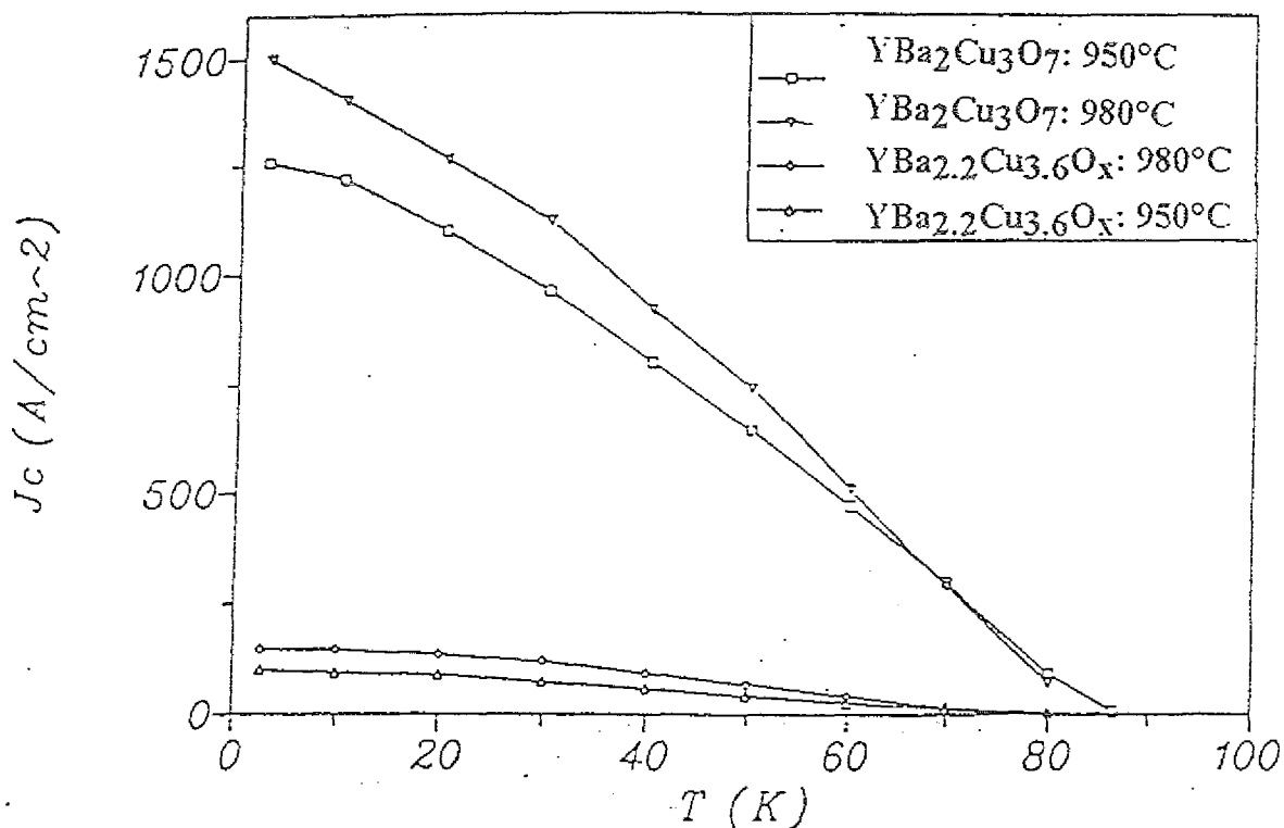
Abb. 38: Die kritische Stromdichte in Abhängigkeit von der Sintertemperatur für mit stöchiometrischem 1-2-3 und überstöchiometrischem, mehrphasigen 1-2,2-3,6 Pulver hergestellten LPPS Schichten.
