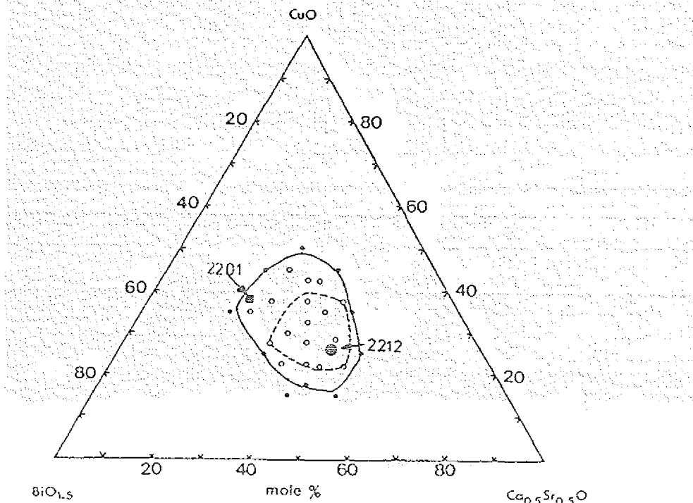
Abb. 69: Der glasformende Bereich im System \text{BiO}_{1.5}\text{-CuO-Sr}_{0.5}\text{Ca}_{0.5}\text{O} : teilweise kristallisiertes Glas, o: Glas /Zhe89/.
