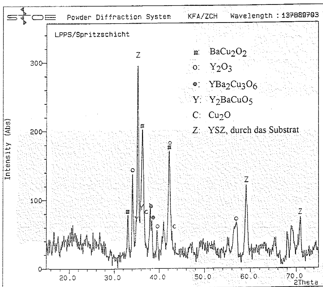
Abb. 28: Röntgenbeugungsdiagramm der aus dem 123-Pulver bei 60 mbar und 26 kW Leistung in einer Argonatmosphäre gespritzten Schicht.
