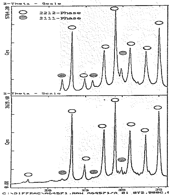
Abb. 81: Röntgenbeugungsdiagramm einer mit 10^\circ\text{C/h} von 900^\circ\text{C} auf 850^\circ\text{C} abgekühlten und bei 850^\circ\text{C}/10\text{h} gehaltenen Probe. Oberes Diagramm 32 kW, unteres Diagramm 40 kW Plasmaspritzleistung.
