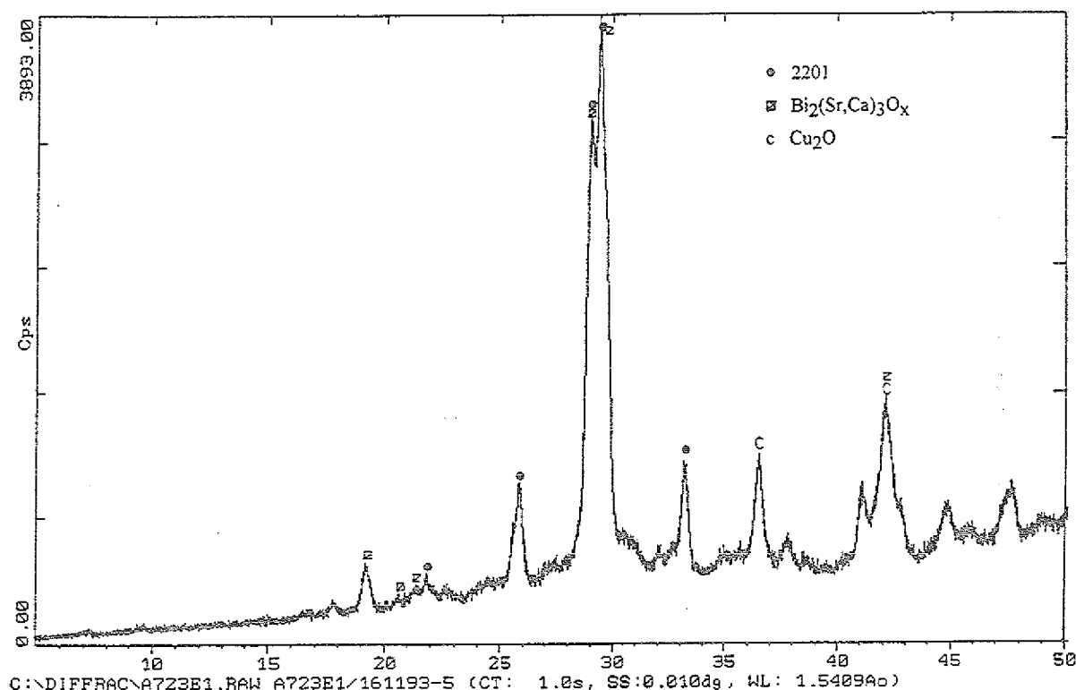
Abb. 67: Röntgenbeugungsdiagramm der mit 40 kW gespritzten 3212-Schicht. CuK \alpha -Strahlung.
