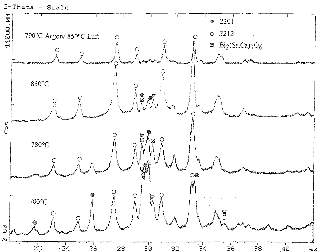
Abb. 74: Röntgenbeugungsdiagramm der aus dem 2212-Pulver hergestellten Spritzschichten für unterschiedliche (10 stündige) Nachbehandlungstemperaturen. CuK \alpha -Strahlung.
