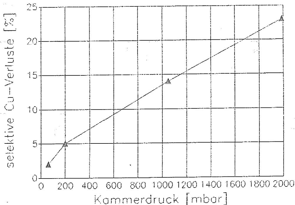
Abb. 27: Einfluß des Kammerdrucks bei 26 kW Leistung auf die selektiven Cu-Verluste.
