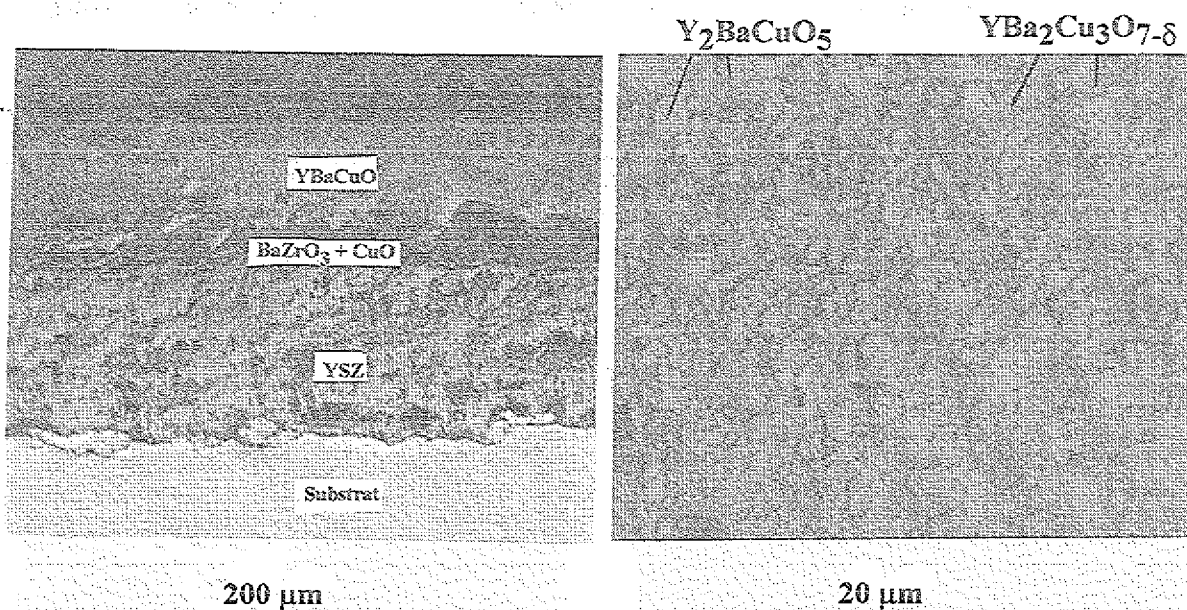
Abb. 56: Querschliff einer an 211-Phase angereicherten, schmelztexturierten Probe. Links 100 fach, mit Substrat, YSZ und YBaCuO-Schicht. Rechts 1000 fach Detail aus der YBaCuO-Schicht. LM.
