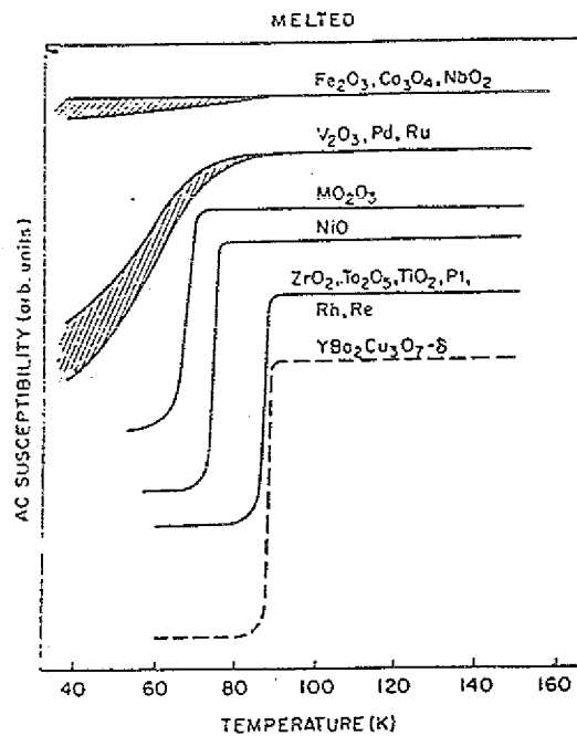
Abb.44: Suszeptibilitätsverlauf von schmelztexturisiertem \text{YBa}_2\text{Cu}_3\text{O}_7 , mit Zusätzen von 10 Gew. % unterschiedlicher Übergangsmetalle oder Metalloxide [Kam90].
