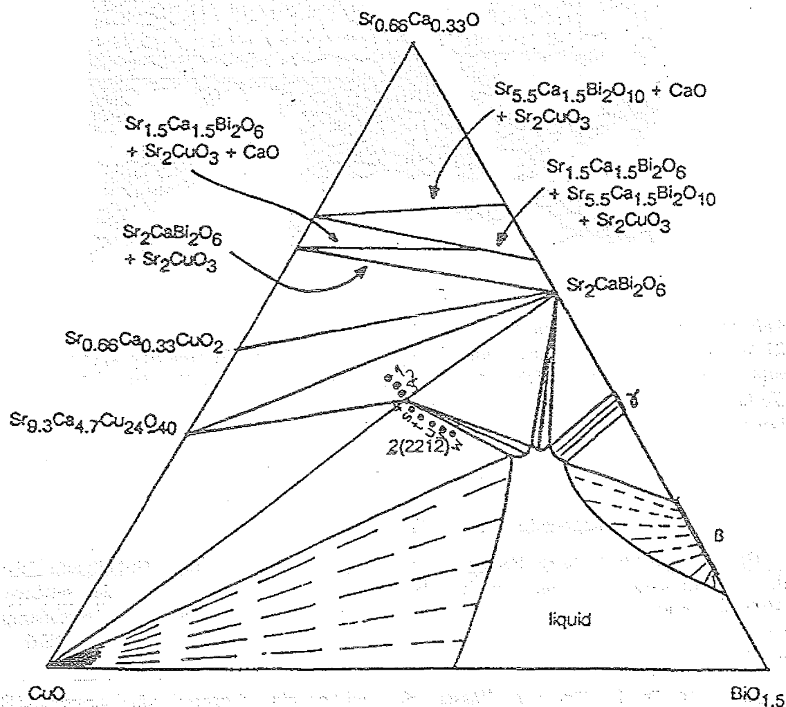
Abb. 64: Lage der verwendeten Spritzpulver und der Spritzschichten in Abhängigkeit von der Spritzleistung im Phasendiagramm (nach [Sch90]) bei 850°C.
