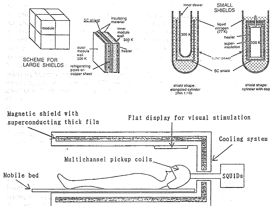
Abb. 102: Oben: Technisches Design möglicher HTSL Schirmungskörper unter Berücksichtigung einer Arbeitstemperatur von 300 K. Links: Modulbauweise zur Herstellung großer Flächen. Rechts: Zylindrische Körper, anwendbar bei kleinen Flächen [Pav92]. Unten: Möglicher Aufbau zur Messung der magnetischen Felder des menschlichen Gehirns [Yos93].
