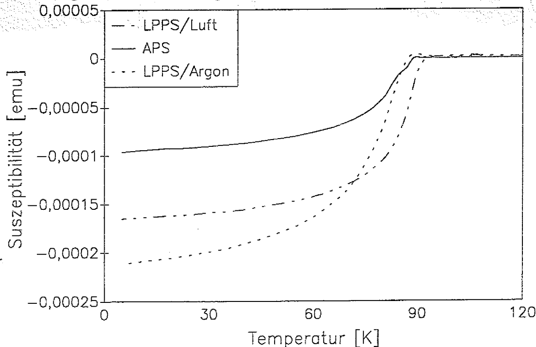
Abb. 40: AC-Suszeptibilität über APS, LPPS (Luft) und LPPS (Argon) hergestellter und bei 950°C/O 2 nachbehandelter Schichten.
