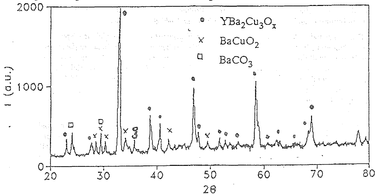
Abb. 37: Röntgenbeugungsdiagramm einer mit 1-2,2-3,6 Pulver hergestellten und bei 950°C nachbehandelten VPS Schicht, CuK \alpha -Strahlung.
