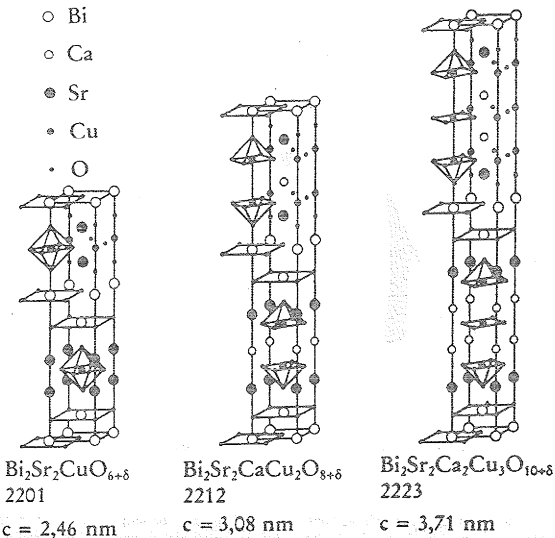
Abb. 11: Struktur von \text{Bi}_2\text{Sr}_2\text{CuO}_6 , \text{Bi}_2\text{Sr}_2\text{CaCu}_2\text{O}_8 und \text{Bi}_2\text{Sr}_2\text{Ca}_2\text{Cu}_3\text{O}_{10} aus /Hoe91/.
