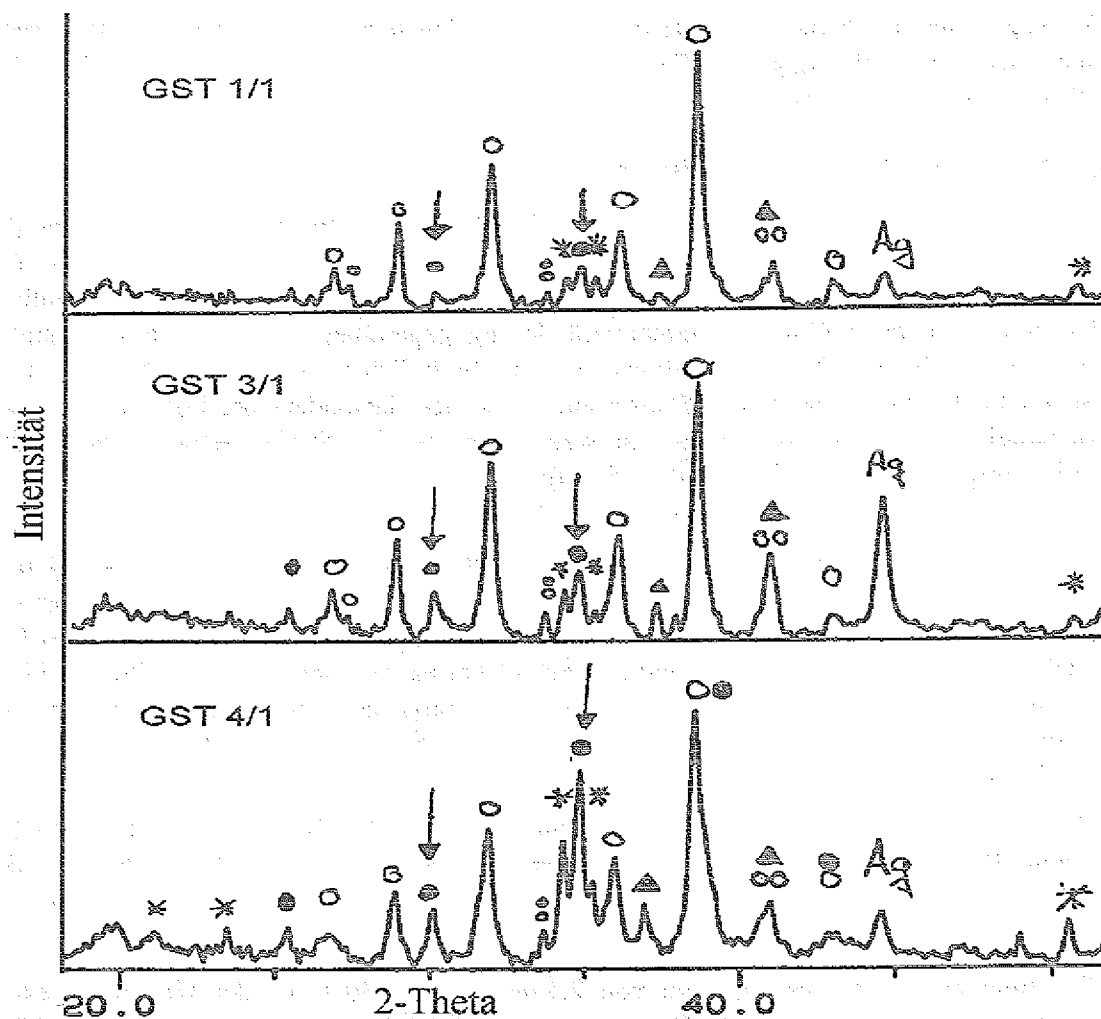
Abb. 76: Röntgenbeugungsdiagramm ( \text{CoK}_\alpha -Strahlung) der bei unterschiedlichen Ziehgeschwindigkeiten und 900^\circ\text{C} maximaler Temperatur schmelztexturierten Schichten. Die mit einem Dreieck gekennzeichneten Peaks sind der (\text{Ca,Sr})_2\text{CuO}_3 -Phase, die mit einem Stern markierten Peaks der \text{Bi}_2(\text{Sr,Ca})_3\text{O}_x -Phase zuzuordnen. Der durch Silber hervorgerufene Reflex ist mit Ag kenntlich gemacht.
