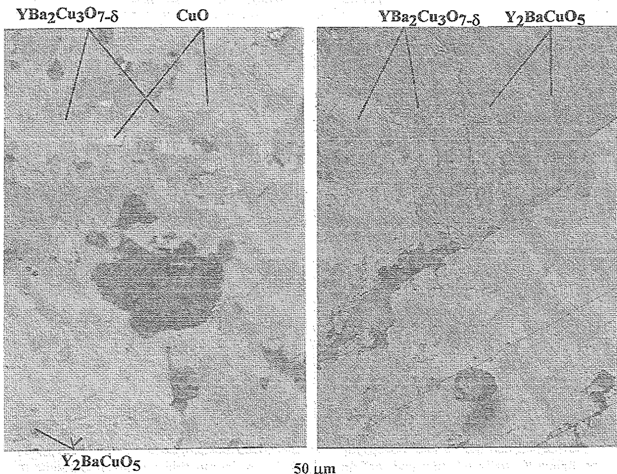
Abb.49: Querschliffe der mit dem Parameter MT 1 (links) und MT 2 (rechts) schmelztexturierten \text{YBa}_2\text{Cu}_3\text{O}_7 -Proben. LM 500.
