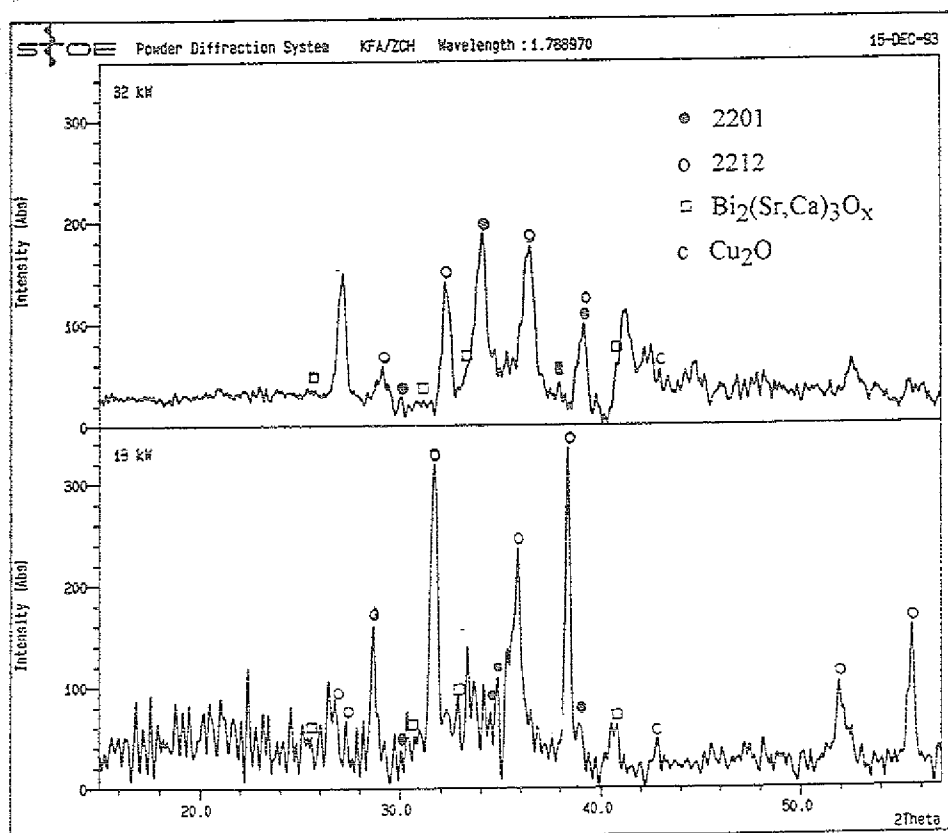
Abb. 63: Röntgenbeugungsanalyse der 2212-Spritzschicht bei 60 mbar und 18 kW (unten), sowie 200 mbar und 32 kW Leistung (oben) CoK α -Strahlung.
