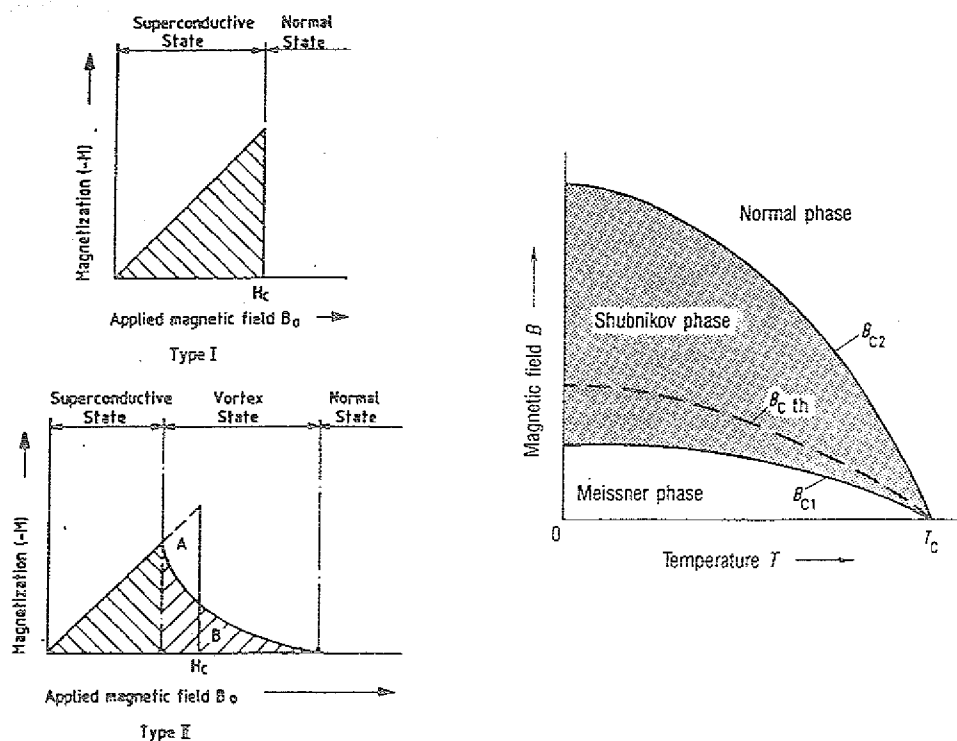
Abb. 1: Links: Verhalten von Supraleitern 1. Art (oben) und 2. Art (unten) im Magnetfeld. Rechts: B-T Zustandsdiagramm eines Supraleiters 2. Art [Buc91].
