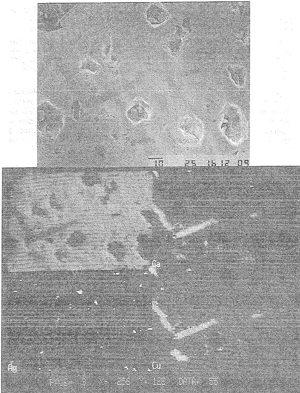
Abb. 83: Querschliff einer mit 250 C/h Abkühlgeschwindigkeit schmelztexturierten Probe mit Elementverteilungsbild. REM
