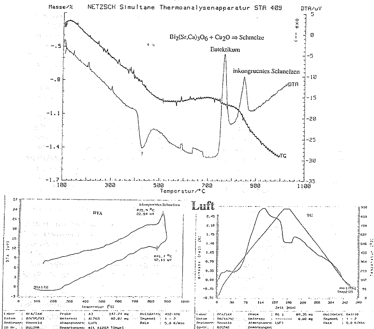
Abb. 70: DTA/TG der aufgemahlenen 3212-Spritzschichten in Stickstoff und in Luft.
