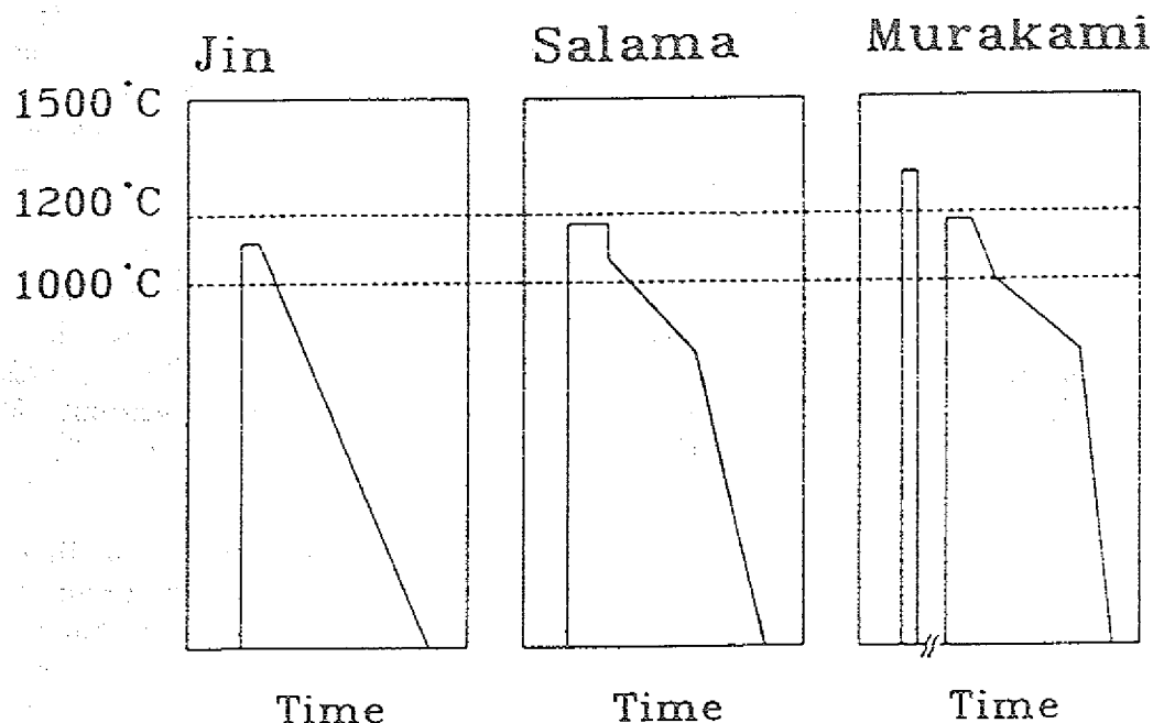
Abb. 10: Schematische Darstellung des Temperatur-Zeit Verlaufes der MTG- /Jin88/, modifizierten MTG- /Sal89/ und QMG (MPMG)- /Mur91/ Prozesse.
