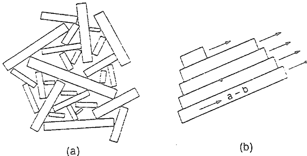
Abb. 9: Schematische Mikrostruktur der 123-Phase nach der Schmelzbehandlung: verursacht durch zu schnelle Abkühlraten (a) und bei \leq 1\text{-}2^\circ\text{C/h} Abkühlgeschwindigkeit (b) nach [Jin92].
