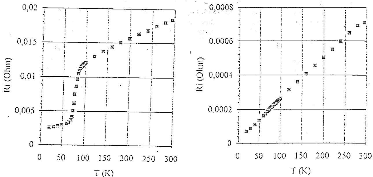
Abb. 86: Widerstand zwischen den Stromkontakten in Abhängigkeit von der Temperatur. Links für eine Probe mit 120 \mu\text{m} Schichtdicke, rechts für eine Probe mit 30 \mu\text{m} Schichtdicke. Der lineare Widerstandsverlauf wird durch das Silbersubstrat verursacht, da durch die geringe Schichtdicke und die Oberflächenrauigkeit keine geschlossene BiSrCaCuO-Schicht vorhanden ist.
