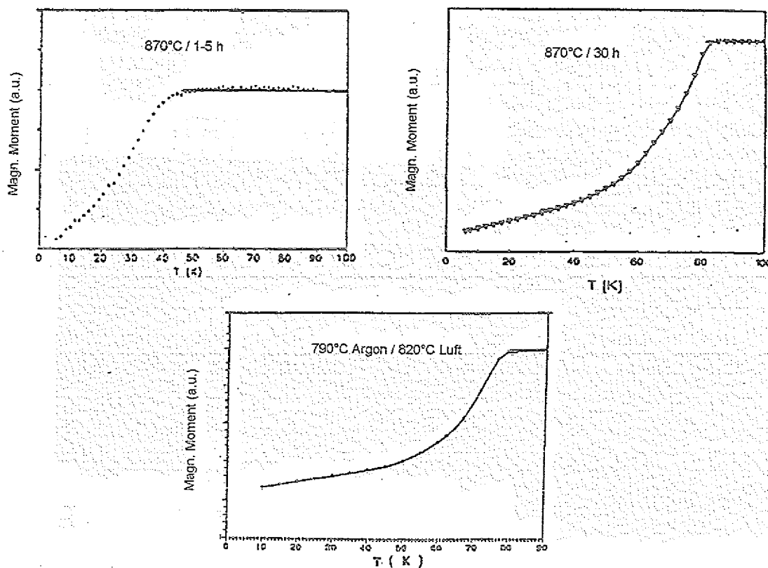
Abb. 75: AC-Suszeptibilität der unterhalb des Schmelzpunktes nachbehandelten 3212-Schichten: links 1h 870°C, rechts 30h 870°C, unten 790°C Argon/820°C Luft.
