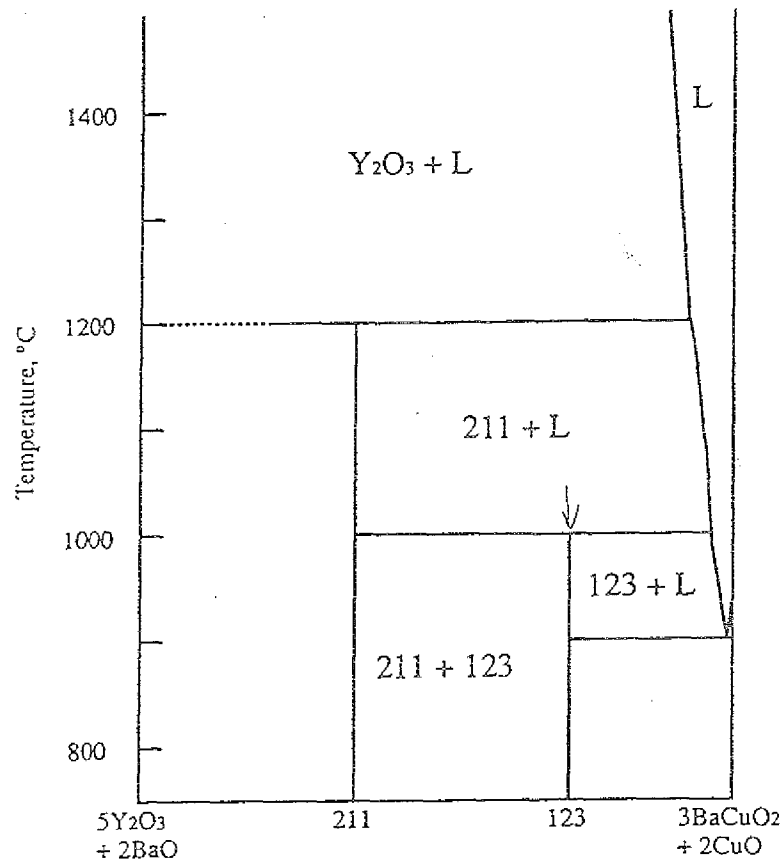
Abb. 7: Phasendiagramm entlang der Konode \text{Y}_2\text{BaCuO}_5\text{-YBa}_2\text{Cu}_3\text{O}_7 nach /Rot88/.
