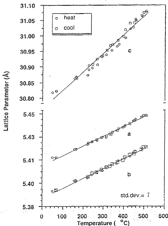
Abb. 15: Temperaturabhängigkeit der Gitterparameter der 2212-Phase nach /Are91/.
