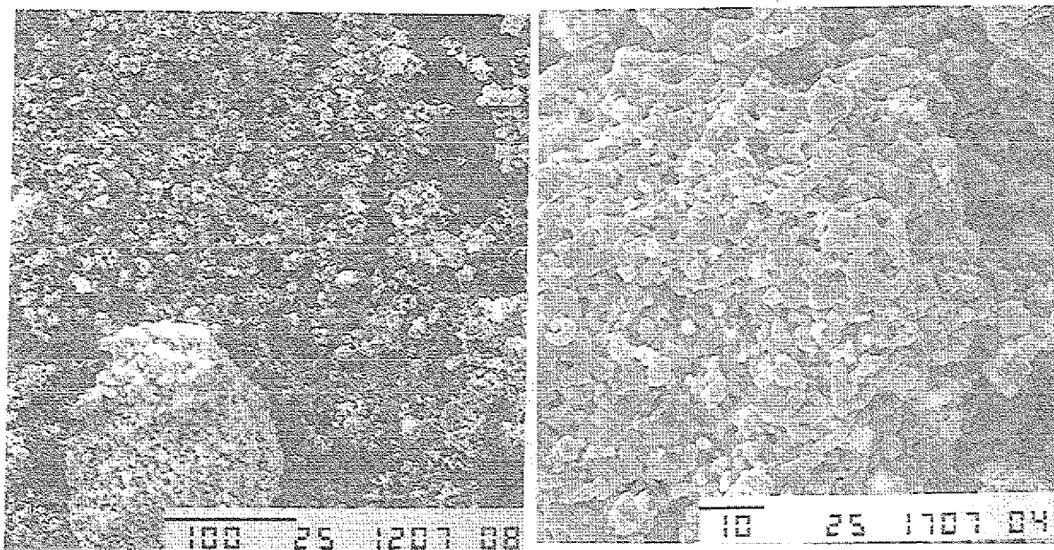
Abb. 20: Sprühgetrocknetes \text{YBa}_2\text{Cu}_3\text{O}_7 -Pulver (DORNIER), REM-Aufnahme.
