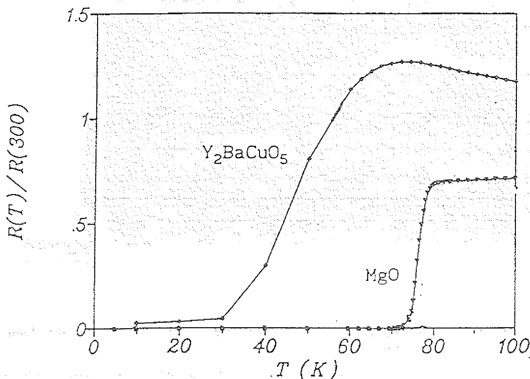
Abb. 48: Widerstandsverlauf schmelztexturierter \text{YBa}_2\text{Cu}_3\text{O}_{7-x} -Proben auf Ni 200 Substrat mit \text{Y}_2\text{BaCuO}_5 - und MgO-Zwischenschichten.
