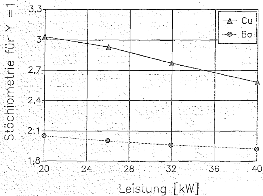
Abb. 26: Zusammenhang zwischen Spritzleistung und selektivem Abdampfen bei 200 mbar Kammerdruck. Ergebnisse der ICP/OES Analyse, normiert auf Y=1 .
