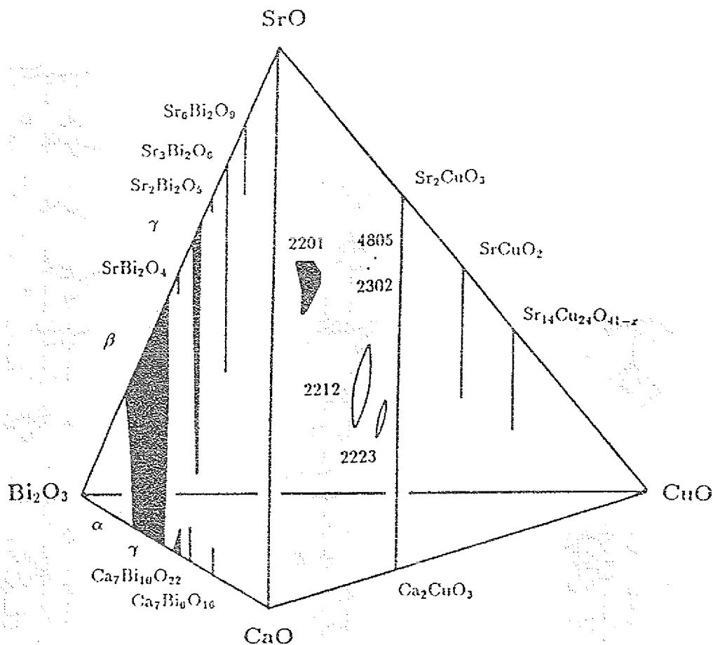
Abb. 12: Komponenten im quaternären System \text{Bi}_2\text{O}_3\text{-SrO-CaO-CuO} bei 850^\circ\text{C} in Luft [Sch90].
