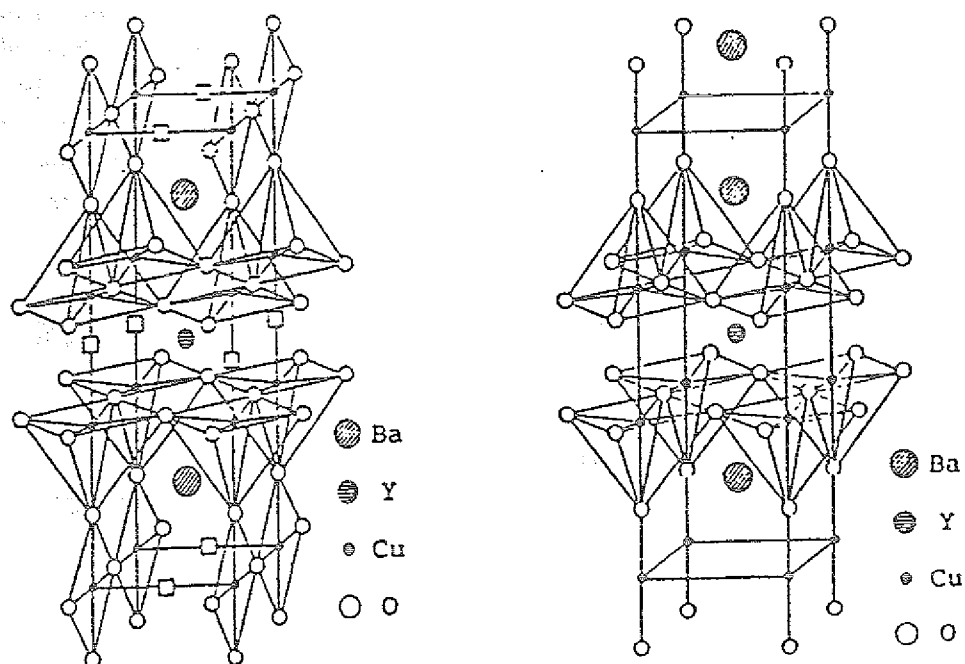
Abb. 3: Struktur der orthorhombischen und tetragonalen \text{YBa}_2\text{Cu}_3\text{O}_{7-\delta} -Phase nach /Fue89/.
