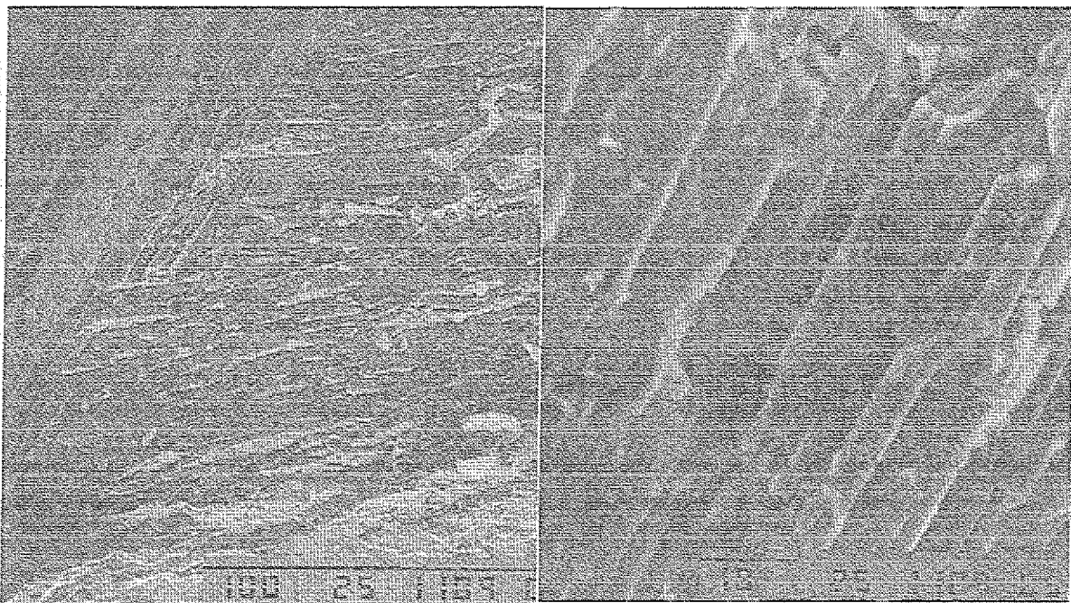
Abb. 50: Bruchfläche einer mit 5 mm/h durch einen Gradienten bewegten, schmelztexturierten Probe. REM 500 (links), 1500 (rechts).
