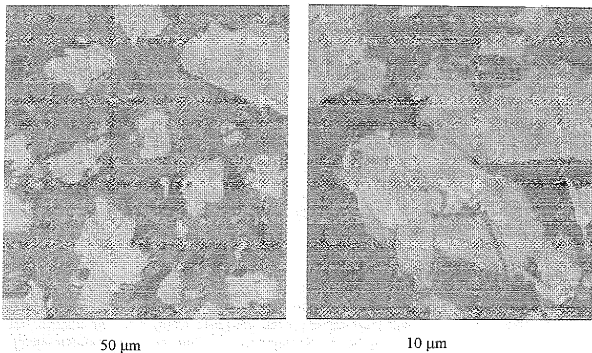
Abb. 20: Sprühgetrocknetes \text{YBa}_2\text{Cu}_3\text{O}_7 -Pulver (DORNIER), REM-Aufnahme.
