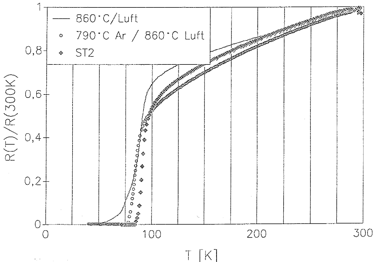
Abb. 90: R(T) Verlauf der mit ST 2 schmelzbehandelten Schicht nach einer Argonnachbehandlung bei 500°C, im Vergleich zu den zweistufig und konventionell gesinterten Schichten. Die Schichten wurden vor der Messung vom Substrat gelöst.
