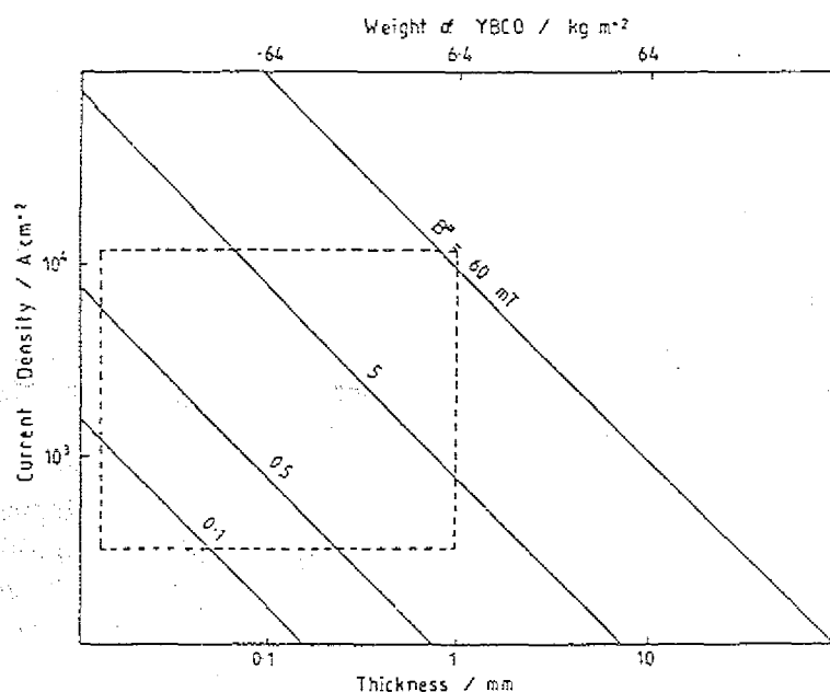
Abb. 93: Abhängigkeit der abschirmbaren Felder von der kritischen Stromdichte und der Schichtdicke der verwendeten HTSL mit Angabe des Gewichtes für die 123-Phase /Tan92/.
