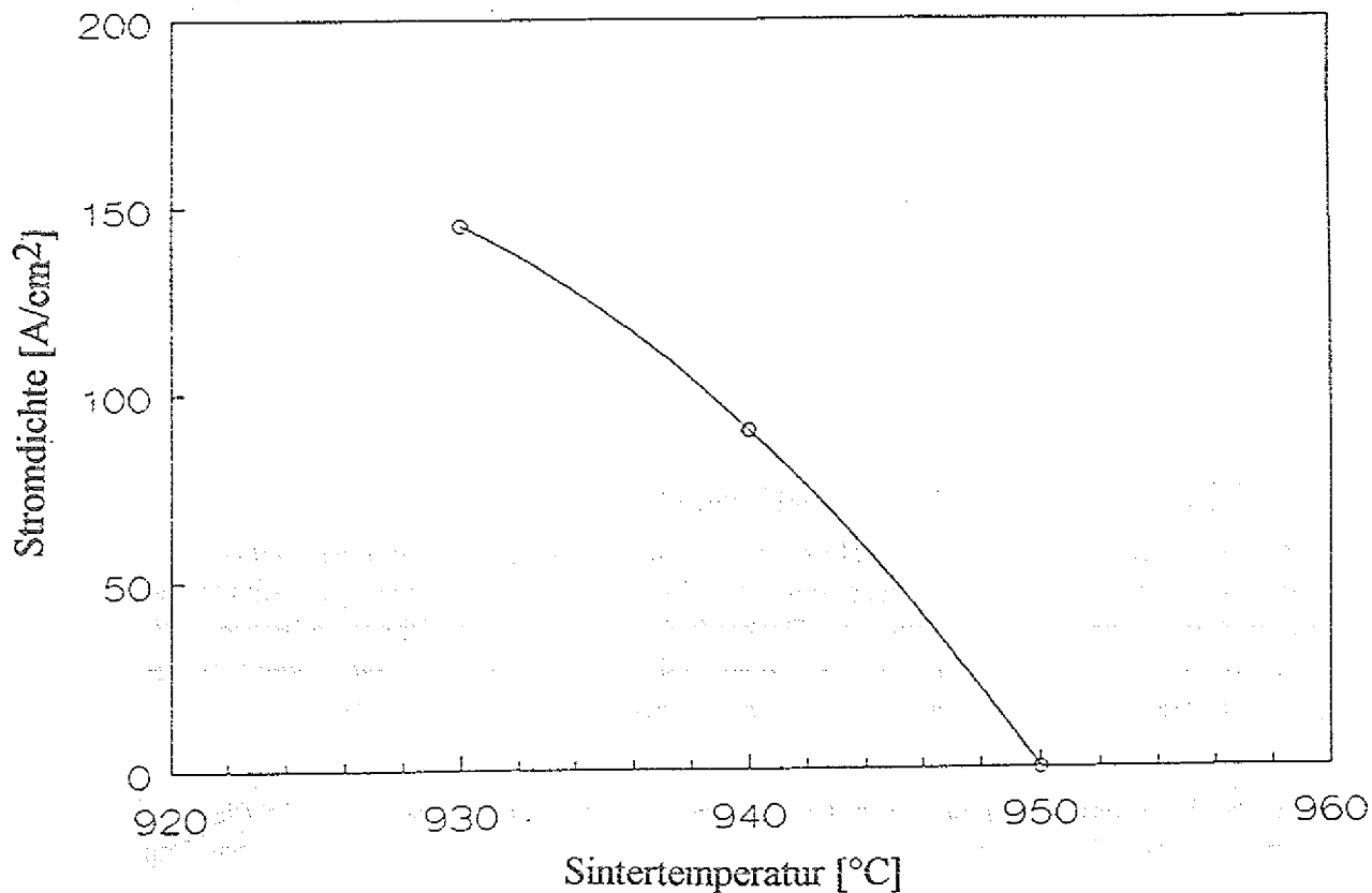
Abb. 31: Stromdichte bei 77 K in Abhängigkeit von der Sintertemperatur (in Luft) für den in Mol mit APS hergestellten Schichtverbund Stahl-NiCrAlY-YBa 2 Cu 3 O 7 / Mol93/.
