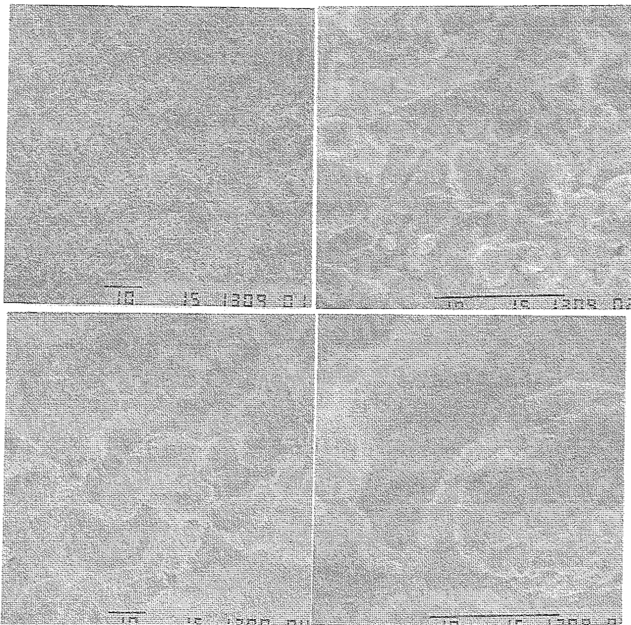
Abb. 24 : Oberfläche einer niederdruckplasmagespritzten Schicht für optimierte Leistung und Substrattemperatur, bei Verwendung eines Haftgrundes (unten). Oben zum Vergleich die Oberfläche einer APS-Spritzschicht.
