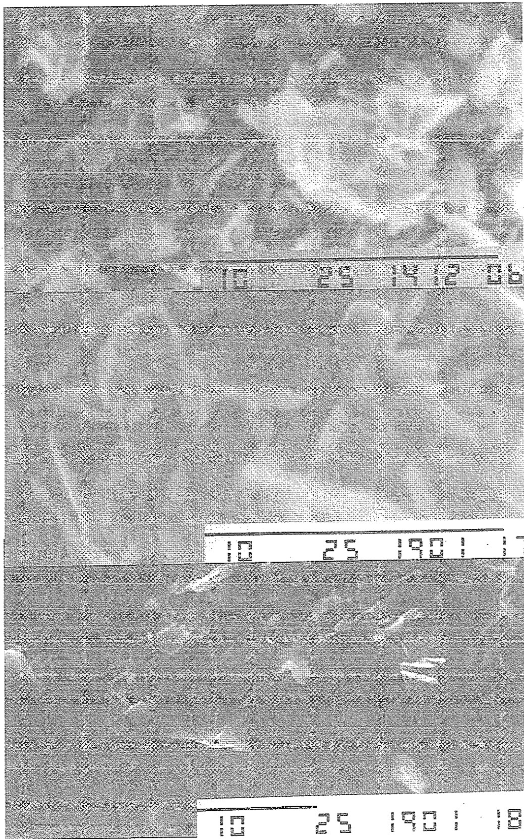
Abb. 76: Oberfläche einer an Luft bei 870°C / 1h (oben), 30h (mitte) und einer zweistufig nachbehandelten Spritzschicht (unten).
