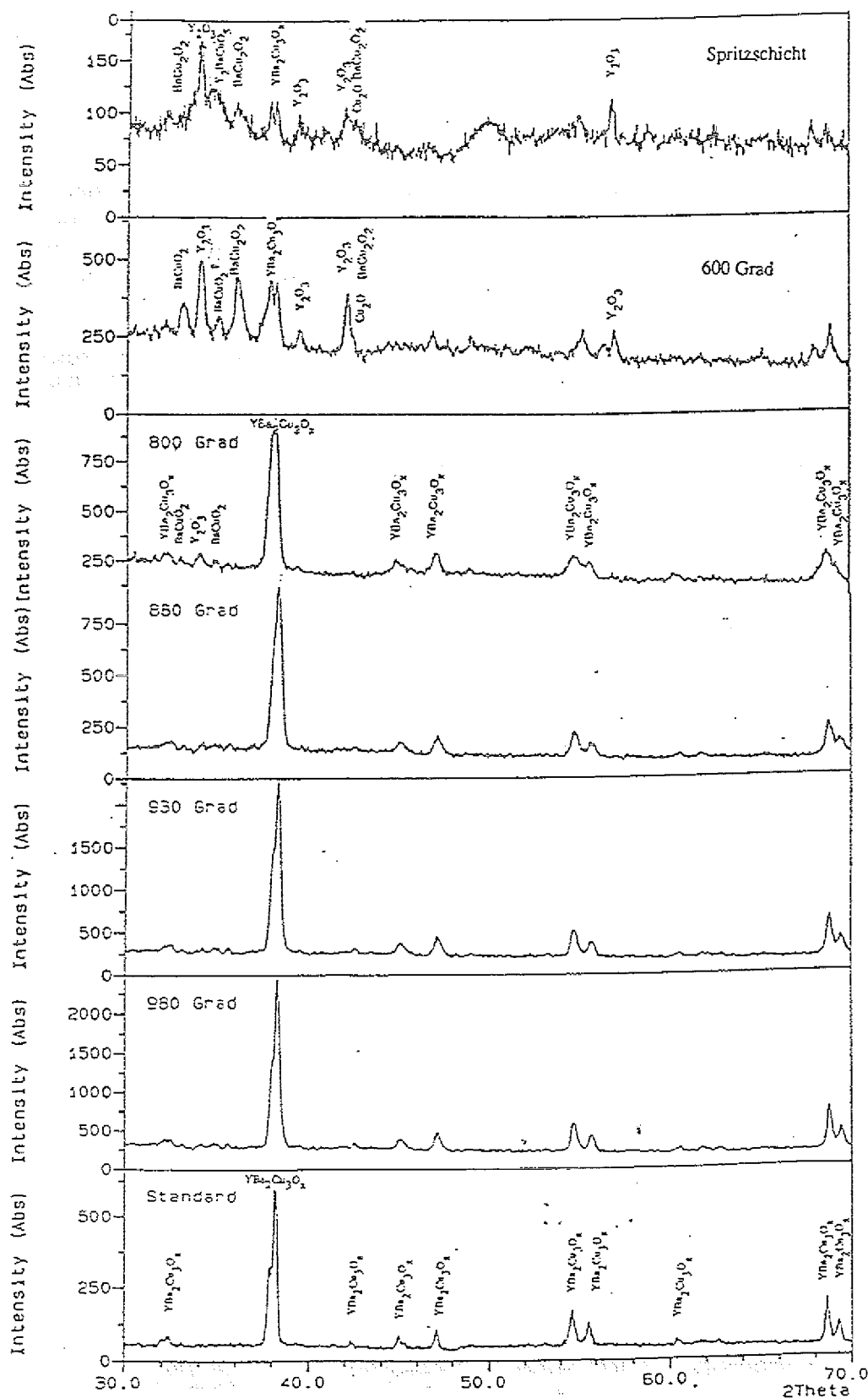
Abb. 32: RBA der bei unterschiedlichen Temperaturen 10 Stunden nachbehandelten YBaCuO-Spritzschichten, CoKa-Strahlung. Als Standard dient das Spritzpulver.
