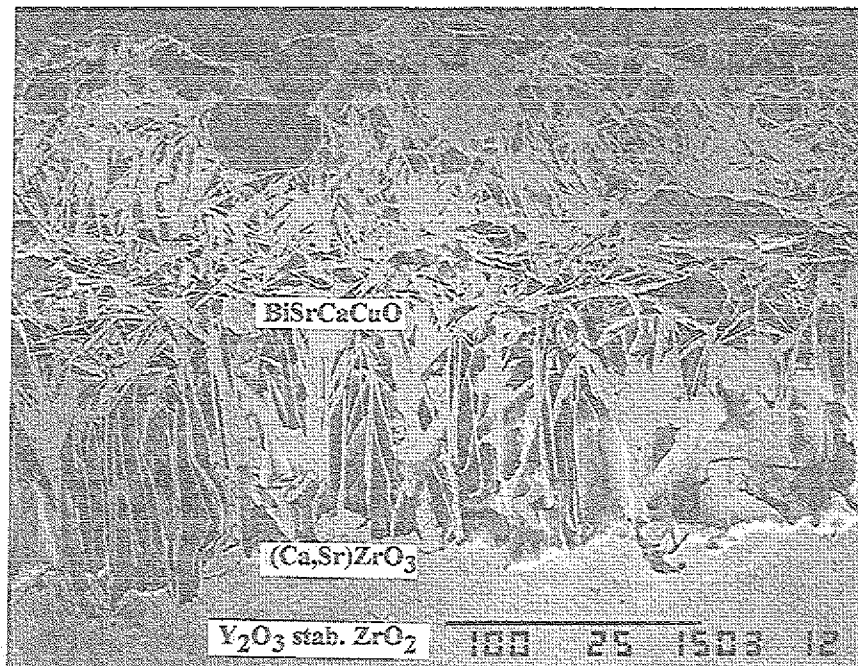
Abb. 85: Querschliff der mit ST2 nachbehandelten Schicht auf einem Stahlsubstrat mit YSZ Zwischenschicht. An der Grenzfläche ist eine deutliche Reaktionszone aus (Sr,Ca)ZrO 3 erkennbar. Die Schicht ist im Vergleich zu den auf Silber texturierten Schichten hoch porös. Vermutlich aufgrund dieser Reaktion sind die 2212-Kristallite im Grenzflächenbereich mit der a,b -Achse senkrecht zum Substrat ausgerichtet.
