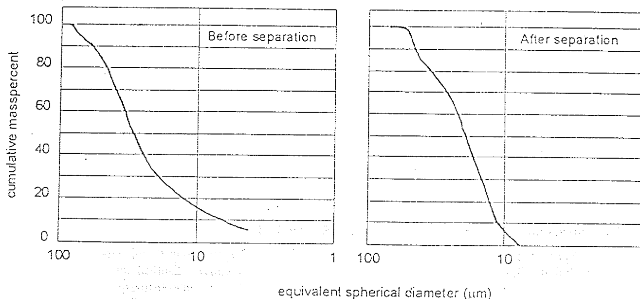
Abb. 22: Korngrößenverteilung des 123-Pulvers vor (links) und des Grobkornes nach der Fraktionierung (rechts).
