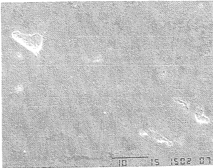
Abb. 65: Querschliff der mit dem 2212-Pulver hergestellten, optimierten Spritzschicht. REM-Aufnahme. Die dunkelen, lamellar auftretenden Bereiche sind Bi-frei (teilweise sind nur Cu und O nachweisbar, teilweise Cu, Sr, Ca und O). Die Bereiche erhöhter Helligkeit sind sehr Bi-reich und Cu-arm oder Cu-frei. Typisch sind die oft auch lamellar auftretenden Poren. Oben links ist die Einbettung nicht vollständig aufgeschmolzener Körner ersichtlich.
