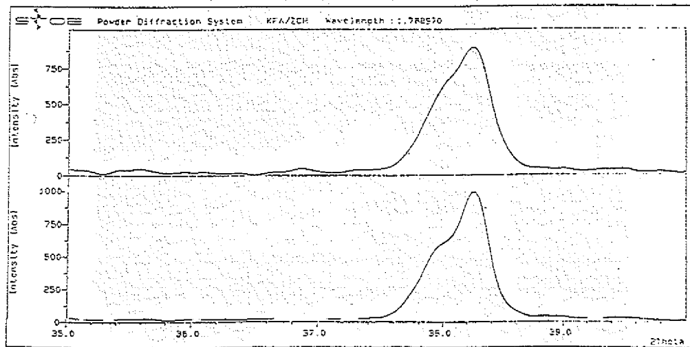
Abb. 96: Röntgenbeugungsdiagramm für YBaCuO auf Stahl/NiCoCrAlY bei einer Nachbehandlungstemperatur von 920°C (oben) und 930°C (unten). 103 und 110 Peak, Co-K \alpha -Strahlung.
