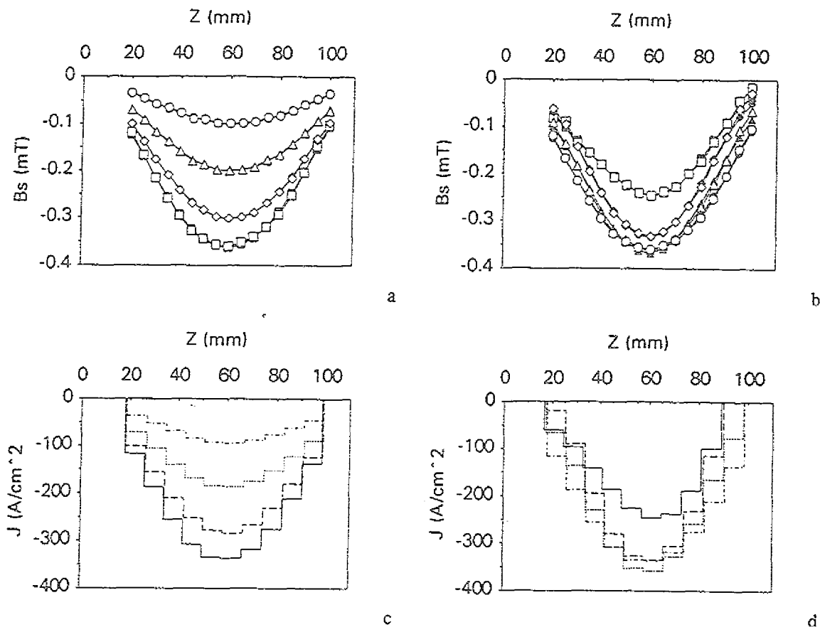
Abb. 99: Schirmungsfeldprofile und davon abgeleitete Stromdichtenprofile für das APS-Rohr, gemessen bei 77 K. (a,c) O, strichpunktiert: 0,1 mT; \Delta , punktiert: 0,2 mT; \diamond , gestrichelt: 0,3 mT; \square , durchgezogen: 0,4 mT. (b,d) \Delta , punktiert: 0,5 mT; \diamond , gestrichelt: 0,7 mT; \square , durchgezogen: 1,0 mT. Offene Symbole sind gemessen, geschlossene berechnet.
