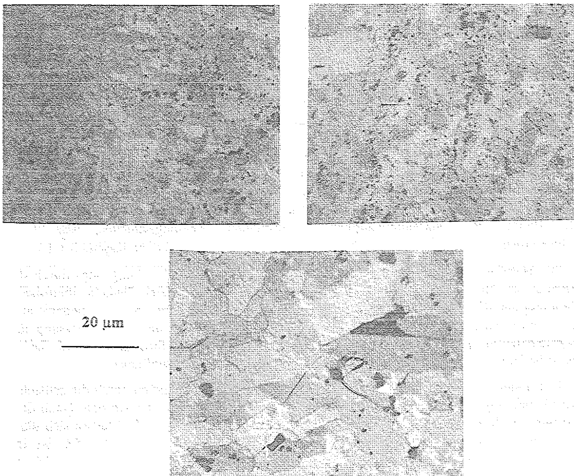
Abb. 34: Querschliff der bei 930°C, 950°C und 980°C nachbehandelten YBa 2 Cu 3 O 7-8 Spritzschichten. LM.
