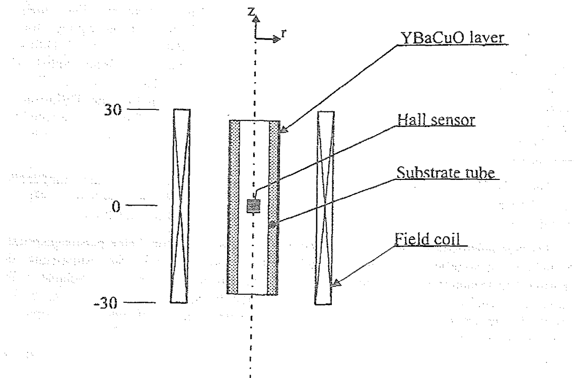
Abb. 19: Experimenteller Aufbau zur Messung der magnetischen Schirmung der supraleitenden Rohre. Der Hall-Sensor kann entlang der Zylinderachse bewegt werden.
