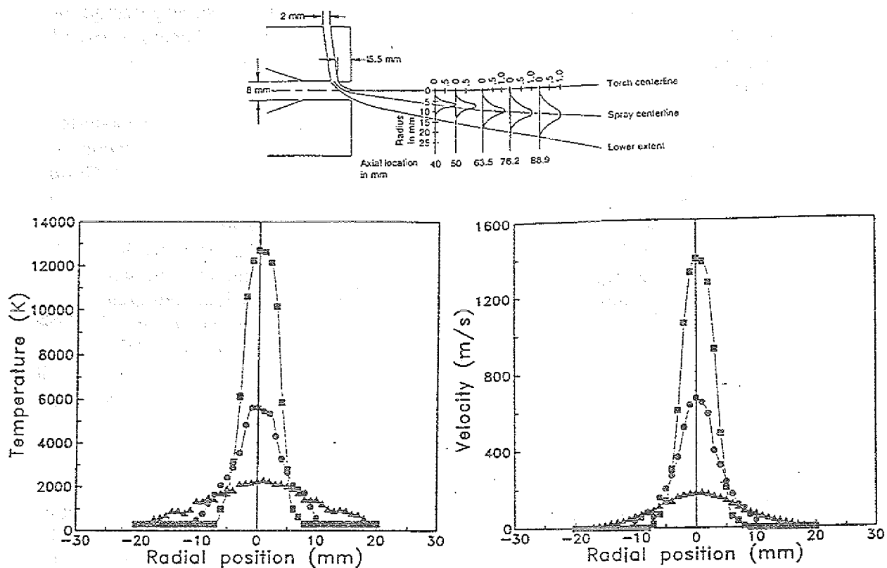
Abb. 17: Radiales Profil der Temperatur (a) und der Gasgeschwindigkeit (b) bei axialen Positionen von 5 ( \diamond ), 30 ( \circ ) und 76,2 ( \triangle ) mm, gemessen von der Stirnseite der Düse in einem Ar/He Plasma [Swa93].
