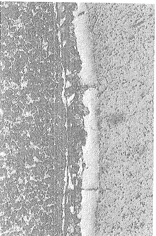
Abb. 100: Querschnitt der auf CaSZ mit QMG 2 schmelztexturierten YBaCuO-Schicht.
