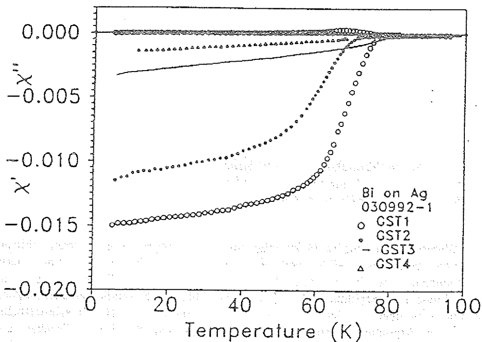
Abb. 87: AC-Suszeptibilität der bei mit 2,5, 12,5, 50 und 250 mm/h bei 900°C maximaler Temperatur durch einen Gradienten gezogenen Proben ohne Nachbehandlung bei 850°C.
