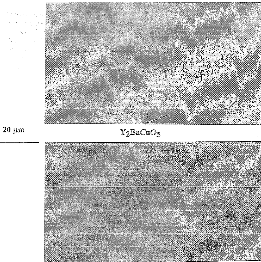
Abb. 54: Lichtmikroskopische Aufnahmen der Querschliffe mit QMG 4 schmelztexturierter Plasmaspritzschichten (oben) und isostatisch gepresster, mit 1^\circ\text{C/h} im Gradienten von 3^\circ\text{C/mm} nach dem MTG-Verfahren schmelztexturierter Presslinge (3 mm dick, 2 cm \varnothing ). Die Presslinge weisen eine über den gesamten Probenbereich reichende Textur auf. Die mittlere Korngröße der 211-Phase ist bei den plasmagespritzten QMG-Proben deutlich geringer.
