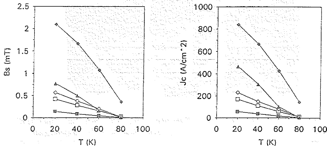
Abb. 97: Temperaturabhängigkeit der Schirmungsfelder und die davon abgeleiteten kritischen Stromdichten.
