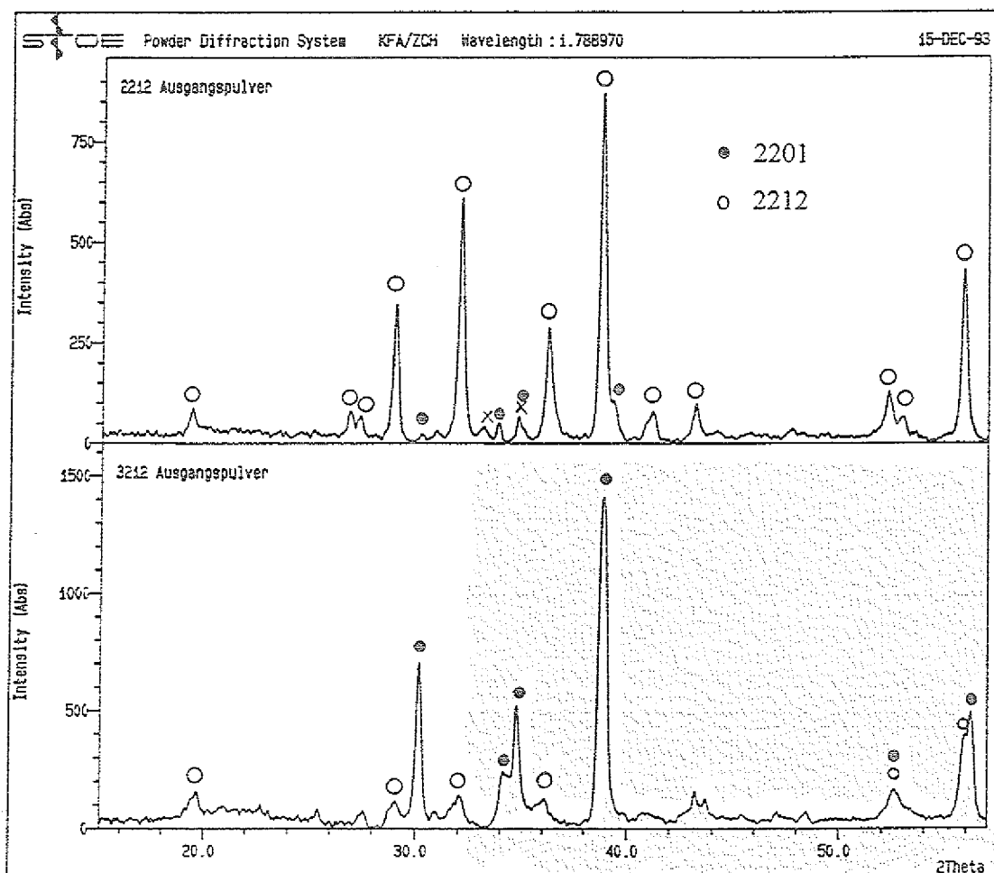
Abb. 59: Röntgenbeugungsdiagramm des 2212 und 3212-Pulvers.
