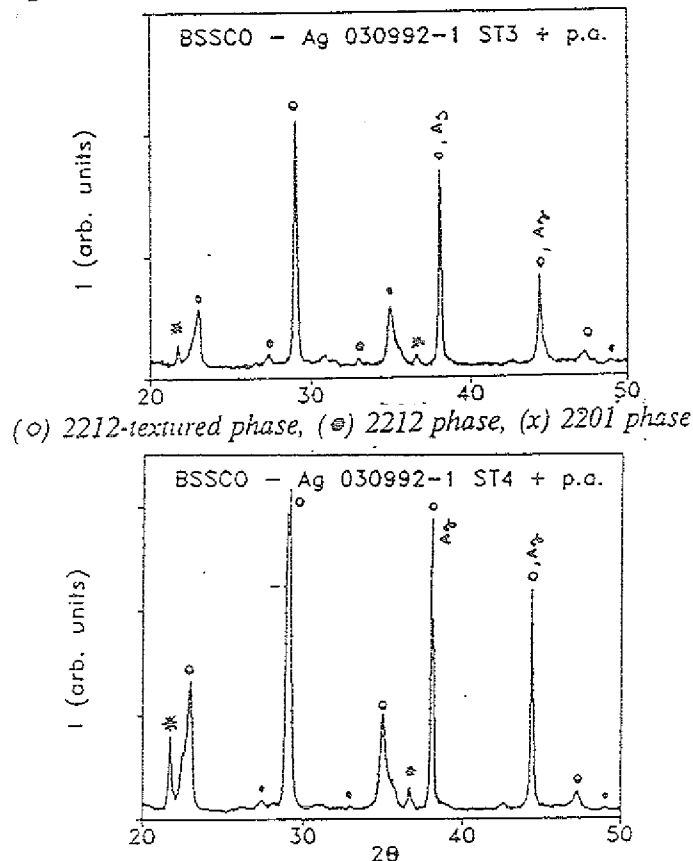
Abb. 89: Röntgenbeugungsanalyse der mit den Parametern ST3 und ST4 hergestellten Schichten nach einer Nachbehandlung bei 850^\circ\text{C}/10\text{h} .
