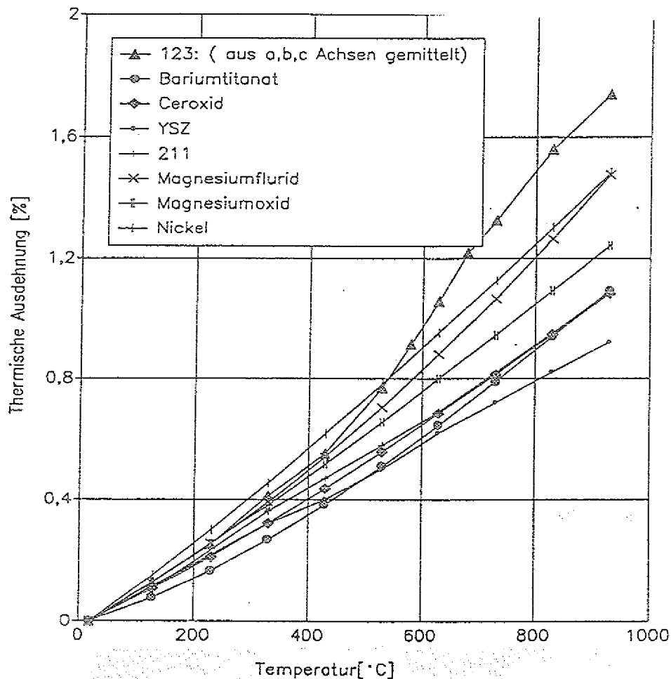
Abb. 43 : Thermische Dehnung untersuchter Substratwerkstoffe und Diffusionsbarrieren nach [The12, Yos88] im Vergleich zur 123-Phase nach [Jor87].
