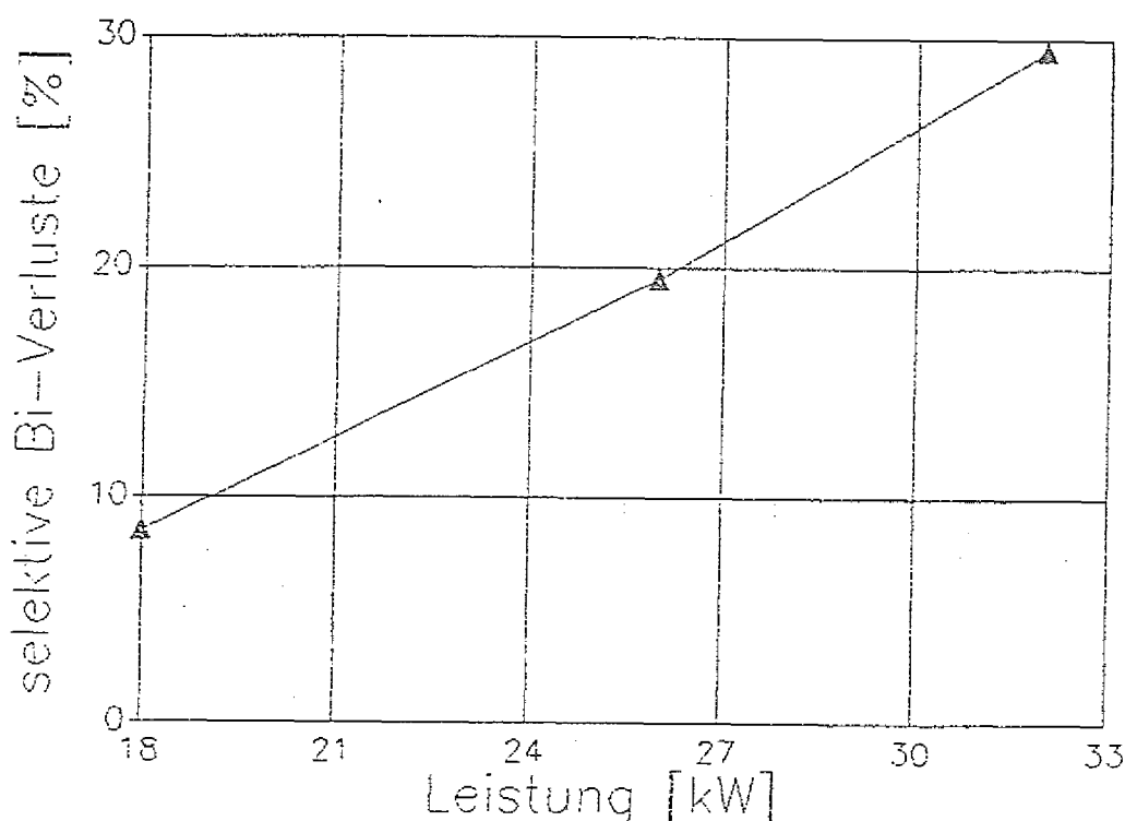
Abb. 62: Bi-Abdampfverluste normiert auf Ca = 1 in Abhängigkeit von der Leistung bei 200 mbar Kammerdruck und einem Spritzabstand von 300 mm. Ar-He Plasma.
