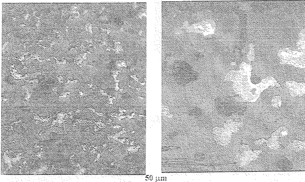
Abb. 57: Querschliff von YBaCuO-Schichten mit 15 Gew.% Silberzusatz nach einer Temperaturbehandlung bei 980°C/10h (links) und nach der Schmelzbehandlung mit Parameter MT2/C (rechts). LM 500.
