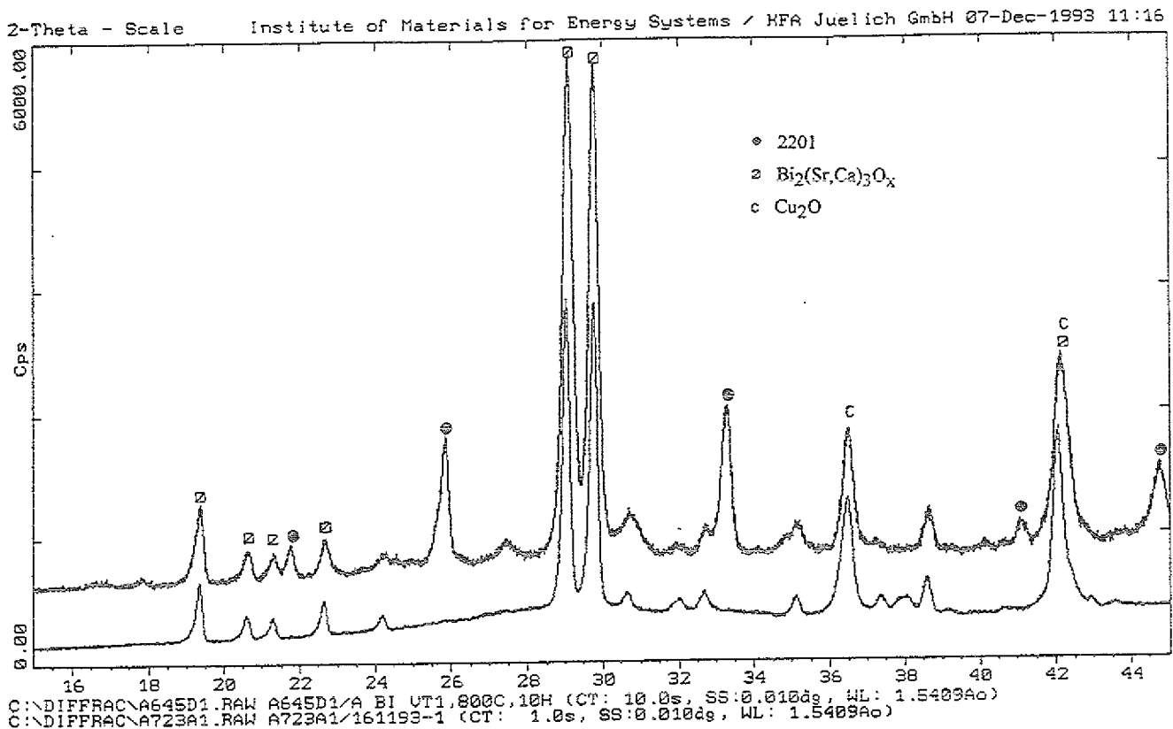
Abb. 72: Röntgenbeugungsanalyse der bei 730°C unterhalb des Eutektikums und bei 800°C oberhalb des Eutektikums in Argon nachbehandelten Spritzschicht. Oberhalb der Eutektikumstemperatur verschwindet die 2201-Phase. CuK \alpha -Strahlung.
