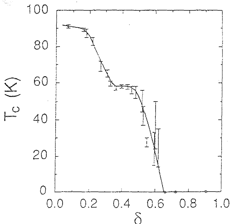
Abb. 4: Zusammenhang zwischen Sprungtemperatur und Sauerstoffgehalt bei \text{YBa}_2\text{Cu}_3\text{O}_{7-\delta} nach /Jor90/.
