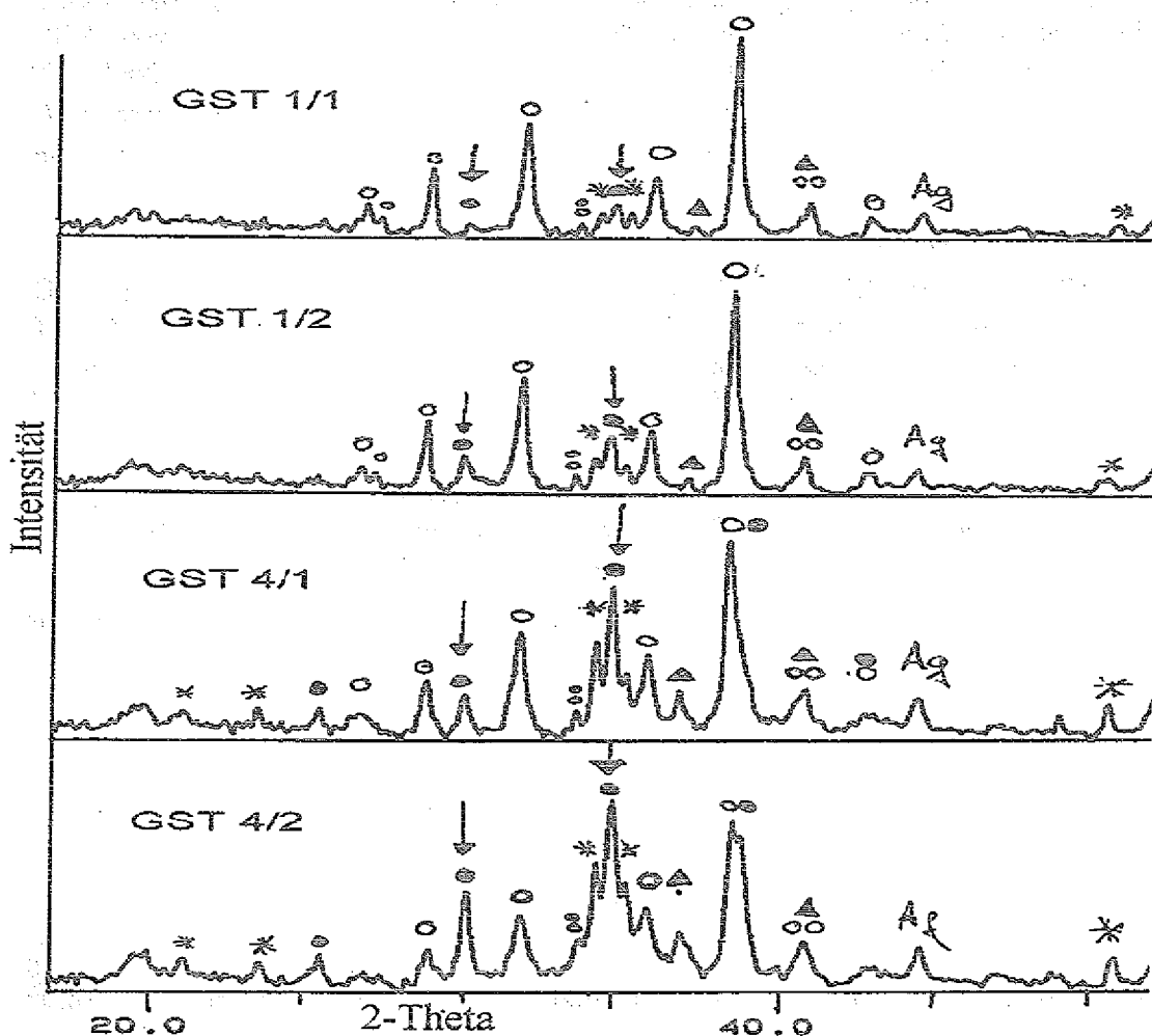
Abb. 77: Röntgenbeugungsdiagramm ( \text{CoK}\alpha -Strahlung) der bei Ziehgeschwindigkeiten von 2,5 und 250 mm/h und Temperaturen von jeweils 900 und 930°C schmelztexturierten Schichten. Phasenzuordnungen wie bei Abb. 76.
