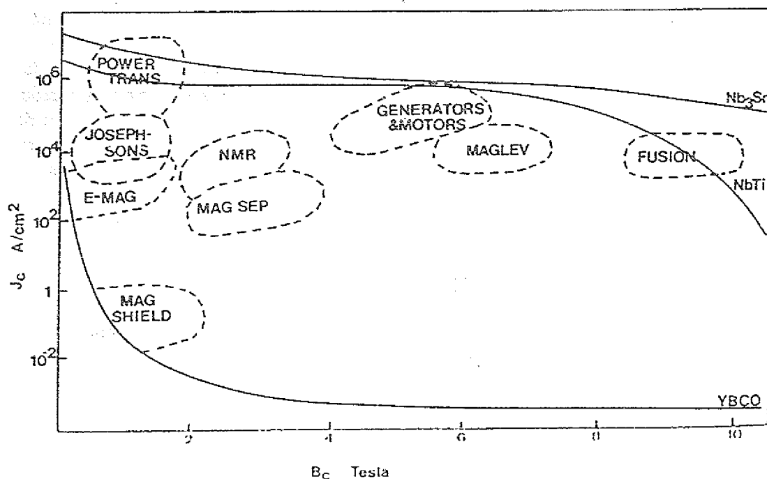
Abb. 92: Potentielle Anwendungsmöglichkeiten der HTSL, basierend auf deren J_c - B_c -Eigenschaften [Cha88].
