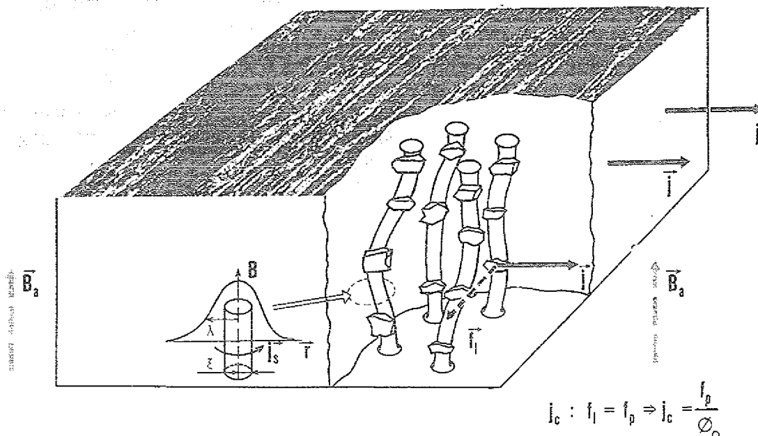
Abb. 2: Einwirkung des Transportstromes auf die Flußschläuche im Supraleiter 2. Art. Die Flußschläuche sind parallel zum angelegten Feld B_a ausgerichtet. Übersteigt die Lorentzkraftdichte f_l die Verankerungskraftdichte f_p , so wandern die Flußfäden in Richtung der Lorentzkraft. Bei f_p = f_l ist die Grenze des verlustlosen Stromtransportes erreicht [Agf91].
