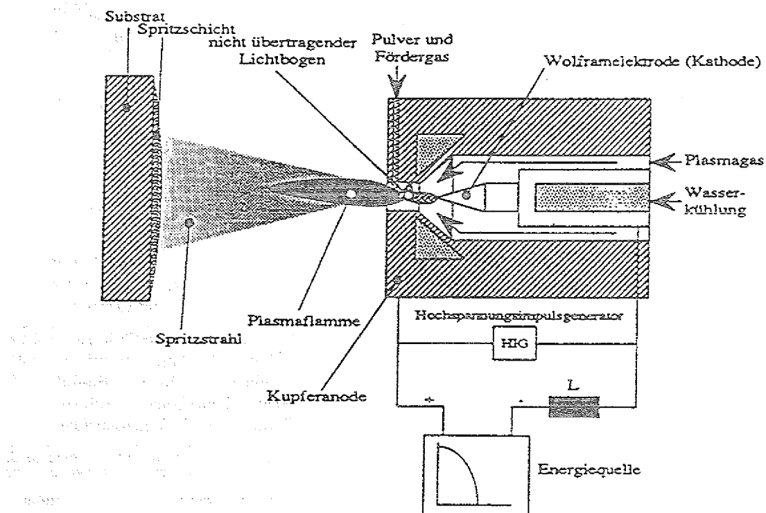
Abb. 18: Schematische Darstellung des Plasmaspritzens [Lug93].
