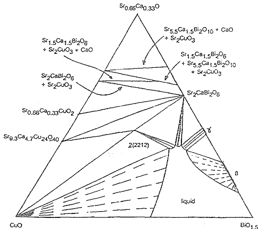
Abb. 13: Schnitt durch den Tetraeder \text{Bi}_2\text{O}_3\text{-SrO-CaO-CuO} , mit 2\text{SrO/CaO-CuO-Bi}_2\text{O}_3 bei T=850^\circ\text{C} in Luft [Sch90].
