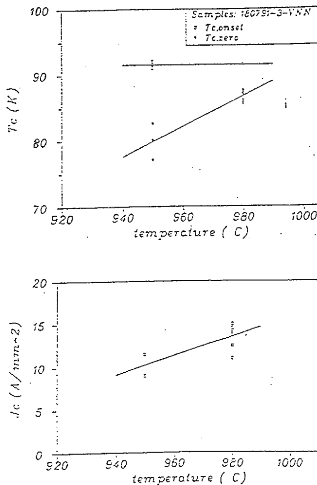
Abb. 33: Sprungtemperatur (a) und kritische Stromdichte bei 4,2 K (b) für unterschiedliche Sintertemperaturen auf Ni 200 Substraten mit Ni-Haftgrund.
