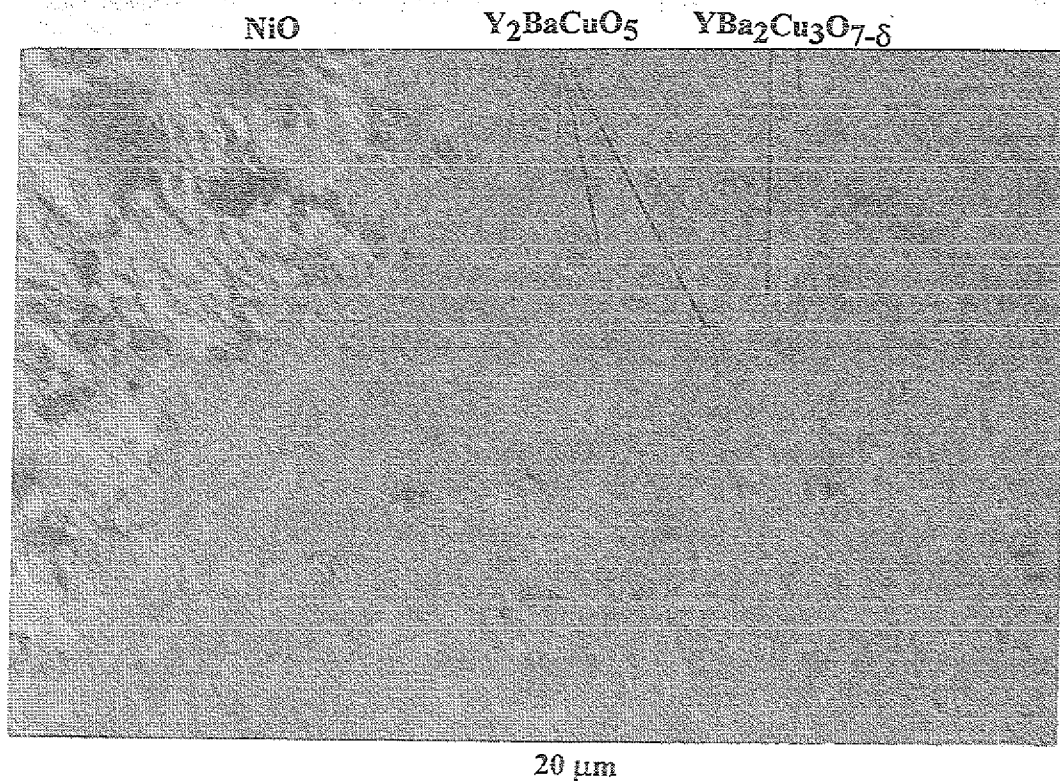
Abb. 46: Querschliff des schmelzbehandelten Schichtverbundes Ni 200-Y 2 BaCuO 5 -123.
