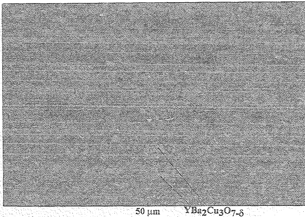
Abb. 25: Querschliff einer bei 26 kW gespritzten Schicht. LM. Die Einbettung nicht vollständig aufgeschmolzener 123-Partikel ist gut erkennbar.
