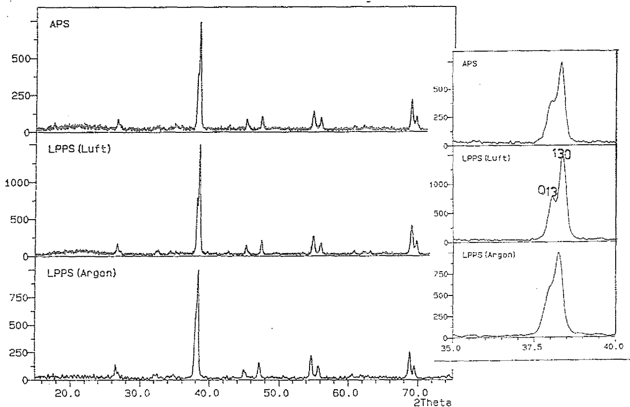
Abb. 39: Röntgenbeugungsdiagramm der mit APS, LPPS (Luft) und LPPS (Argon) gespritzten und bei 950°C/O 2 nachbehandelten Schichten Co K \alpha -Strahlung.
