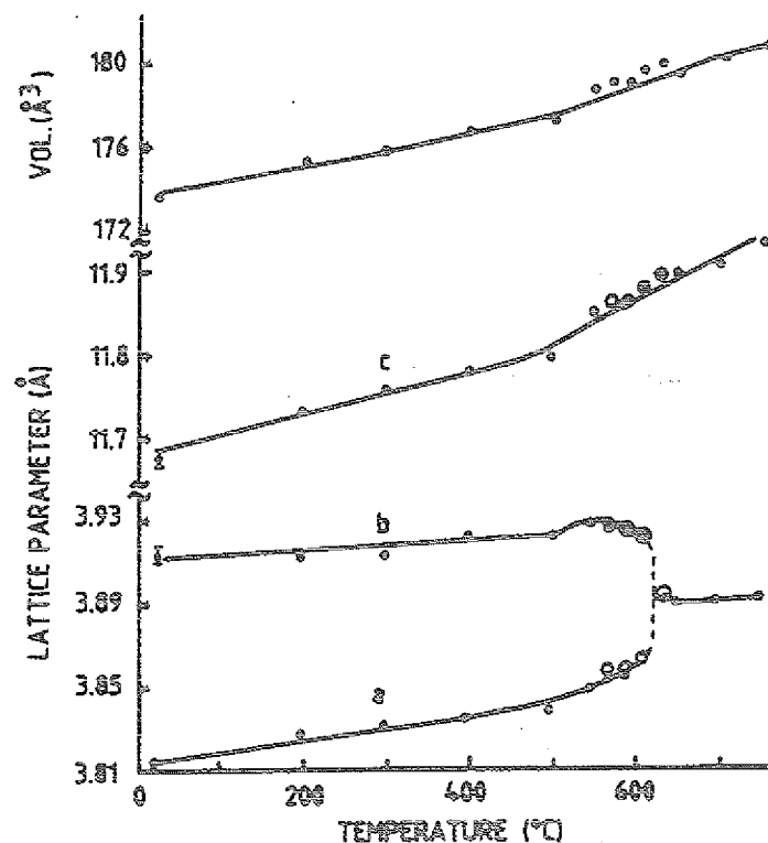
Abb. 8: Temperaturabhängigkeit der Gitterparameter und des Volumens der Elementarzelle der 123-Phase nach /Jor90/.
