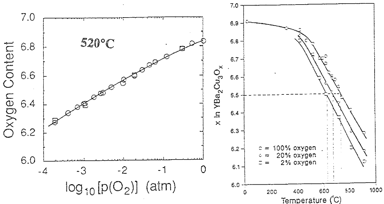
Abb. 5: Abhängigkeit des Sauerstoffgehaltes von der Temperatur und dem Sauerstoffpartialdruck /Jor90/.
