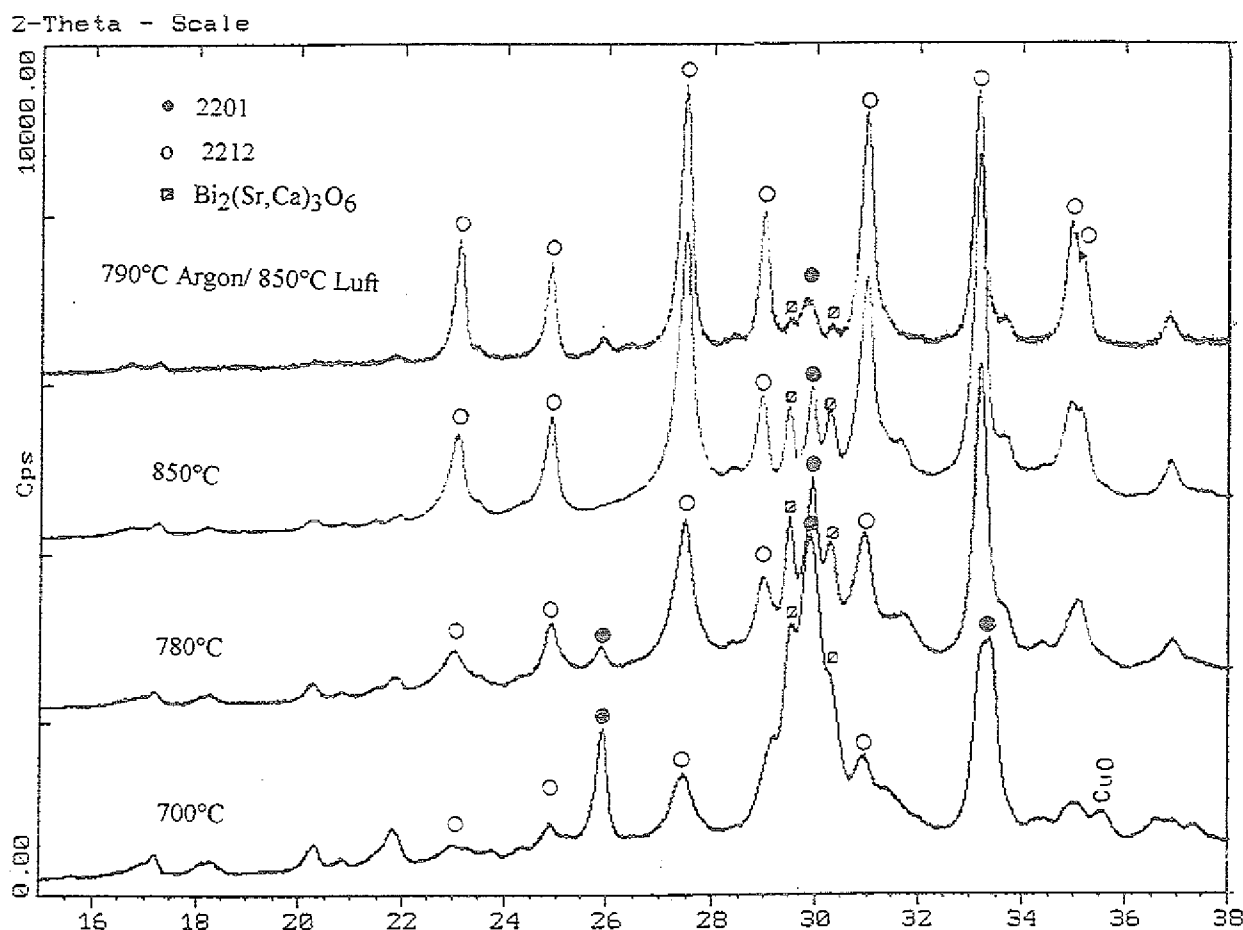
Abb.73: Röntgenbeugungsdiagramm der bei unterschiedlichen Temperaturen 10 Stunden an Luft nachbehandelten 3212-Schichten, im Vergleich zu einer 2-stufig nachbehandelten Spritzschicht. CuK \alpha -Strahlung
