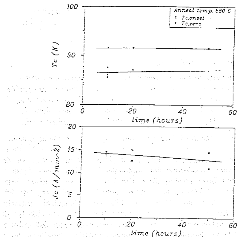
Abb. 35: Sprungtemperatur (a) und kritische Stromdichte bei 4,2 K (b) für unterschiedliche Haltezeiten bei 980°C.
