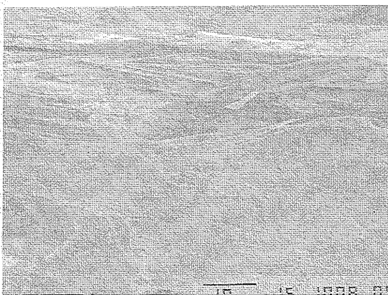
Abb. 82: Bruchfläche einer optimiert schmelzbehandelten Probe. REM-Aufnahme. Die RBA ( \text{CuK}\alpha ) in Reflexion (oben) zeigt die Textur im oberflächennahen Bereich.
