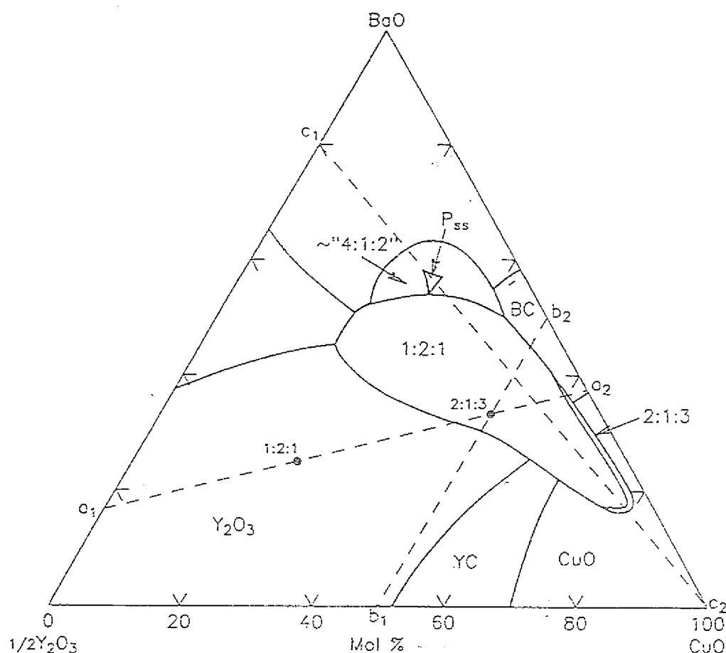
Abb. 6: Primärausscheidungsfelder im System \text{Y}_2\text{O}_3 -BaO-CuO /Rot88/.
