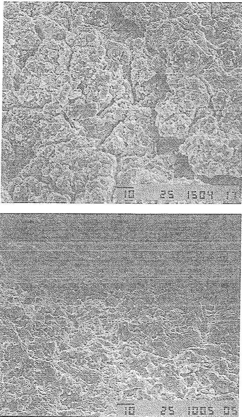
Abb. 95: Oberflächen der mit \text{BaTiO}_3 (links oben) bei 920^\circ\text{C} , sowie der ohne \text{BaTiO}_3 bei 930^\circ\text{C} (unten 130\text{ }\mu\text{m} Schichtdicke) getemperten Schichten. Der untersuchte Probenbereich ist jeweils der Übergang von der Zylinderfläche zur geschlossenen Seite. REM 750.
