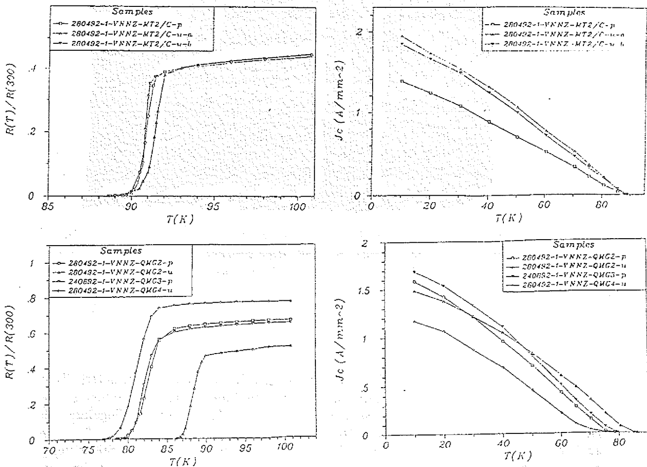
Abb. 55: Temperaturabhängigkeit des Widerstandes und der Stromdichte schmelztexturierter YBaCuO Proben.
