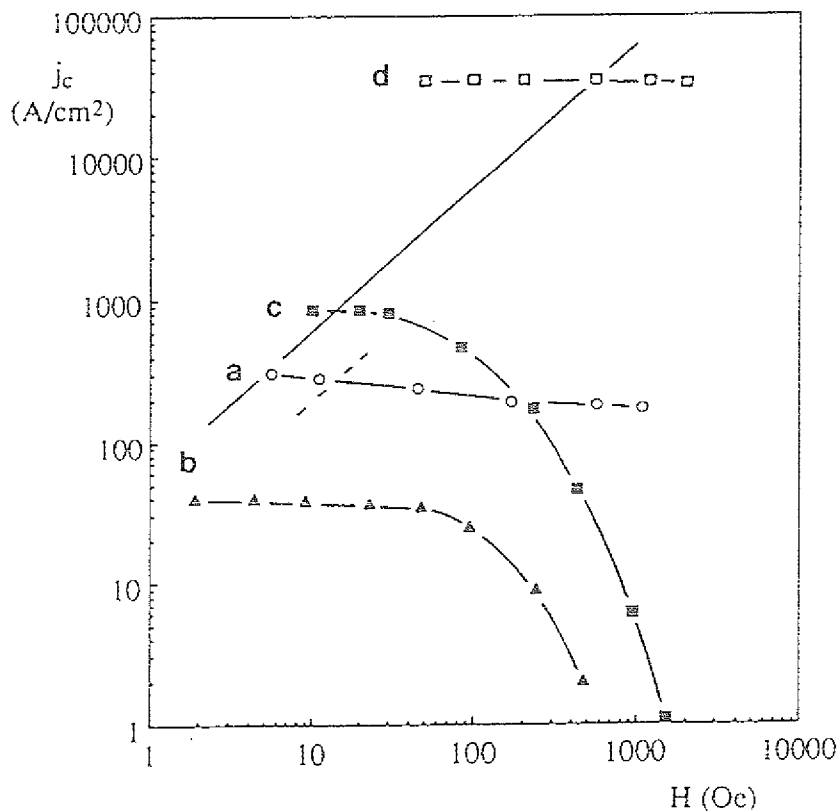
Abb. 16: J_c(H) für 2212. (a) Gesinterte Keramik bei 4,2 K. (b) "Melt cast" Proben (nach dem Hoechst Verfahren [Boc89]) bei 77 K. (c) Schmelztexturierte Keramik bei 77 K. (d) Schmelztexturierte Keramik bei 4,2 K [Pau91].
