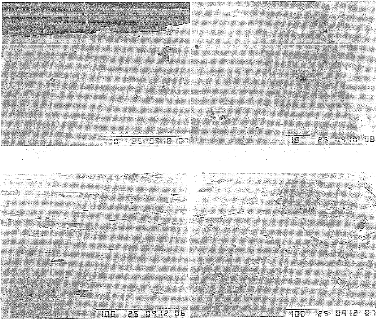
Abb. 91: Bereich guter Textur der a,b -Ebenen parallel zum Substrat bei einer mechanisch zwischen 2 Silbersubstraten eingebetten, schmelztexturierten \text{BiSrCaCuO} -Probe (unten) und bei einer auf 60\text{ }\mu\text{m} reduzierten Schichtdicke (oben). REM.
