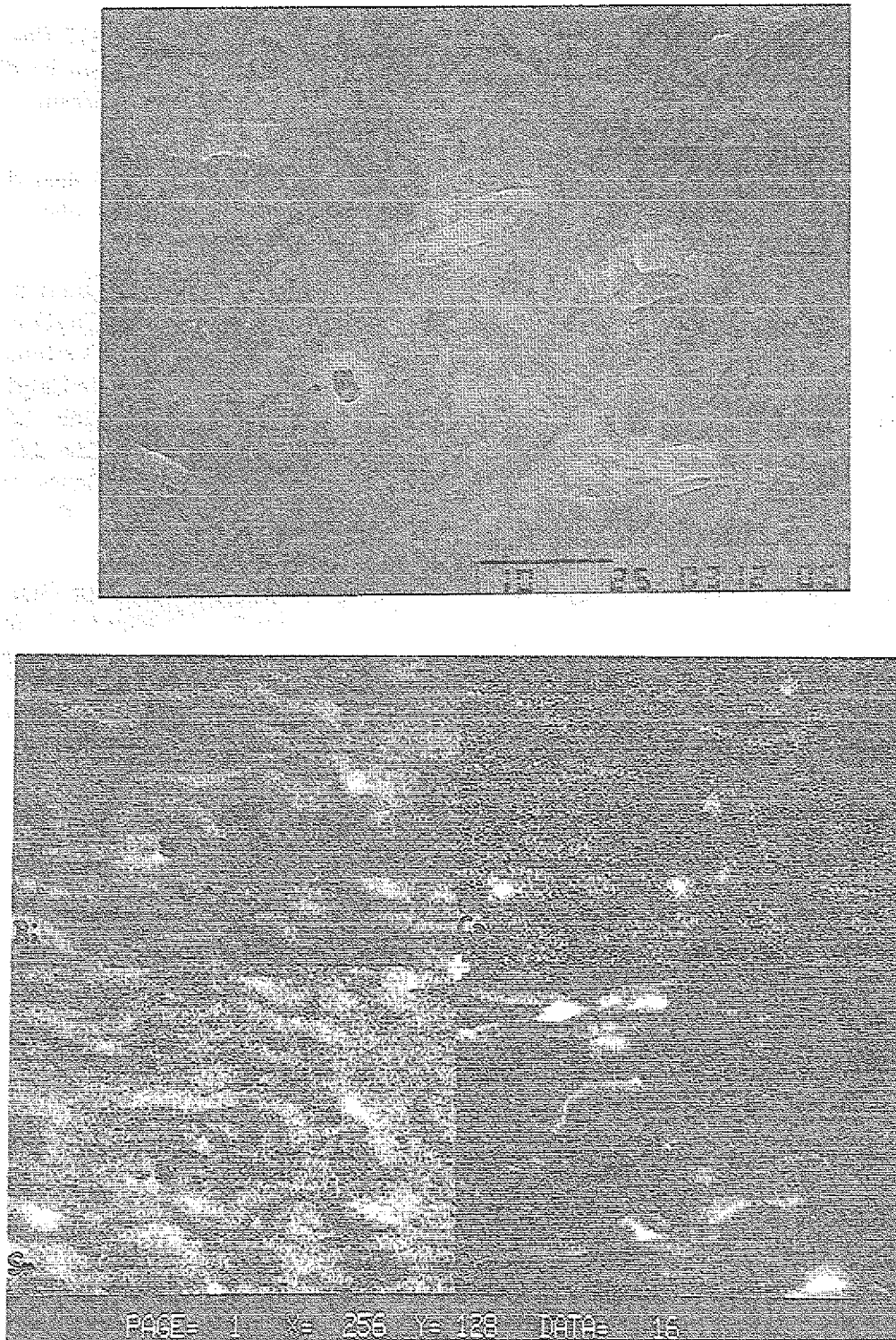
Abb. 68: REM-Aufnahme des Schliffbildes einer bei 40 kW gespritzten Probe mit dazugehörigem Elementverteilungsbild.
