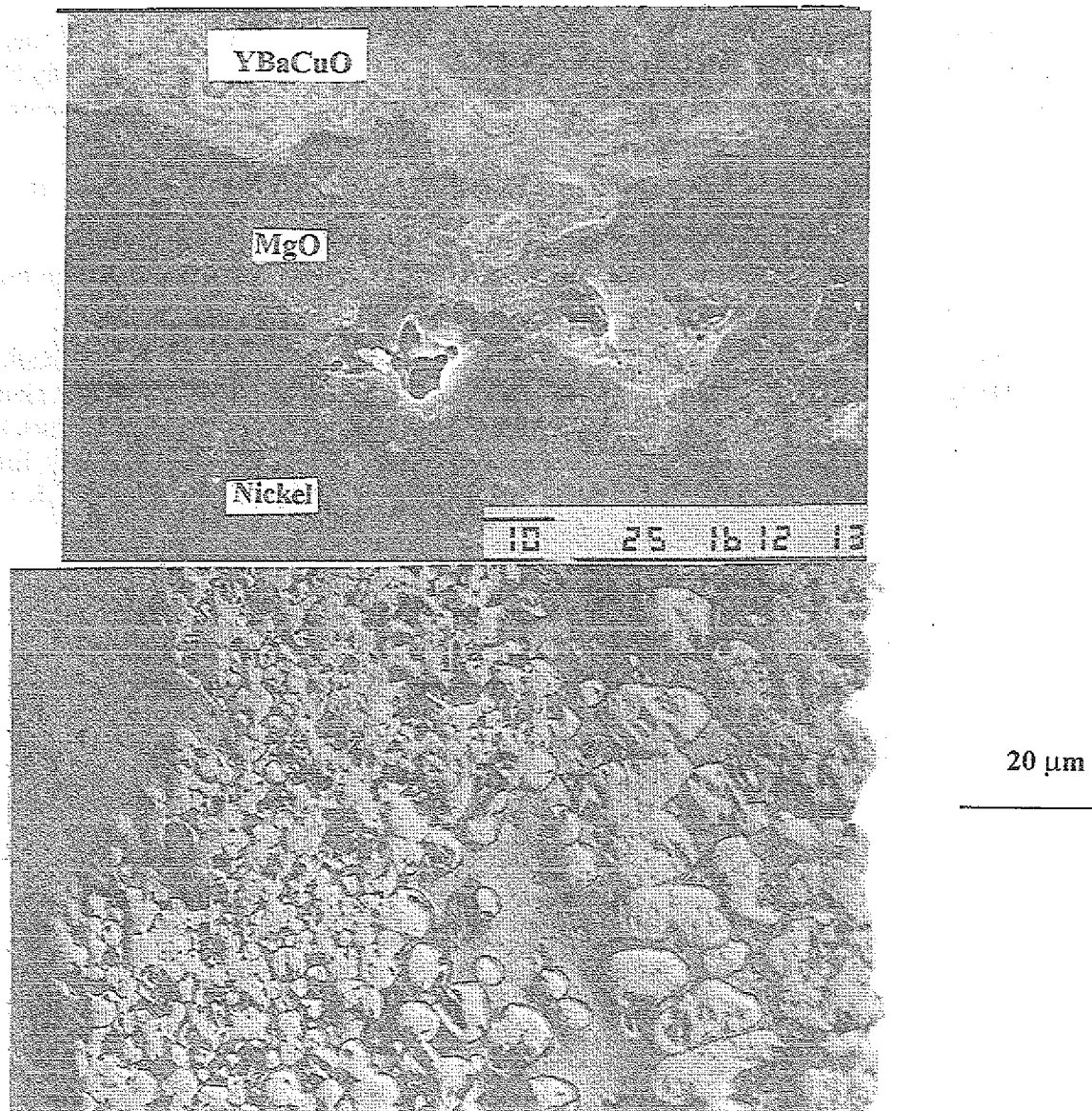
Abb. 47: Ni 200-MgO-YBaCuO Schichtverbund vor (REM 1000 fach) und nach der Schmelztextur (LM 1000 fach). Deutlich ist die Zerstörung der vorher dichten MgO-Schicht zu erkennen.
