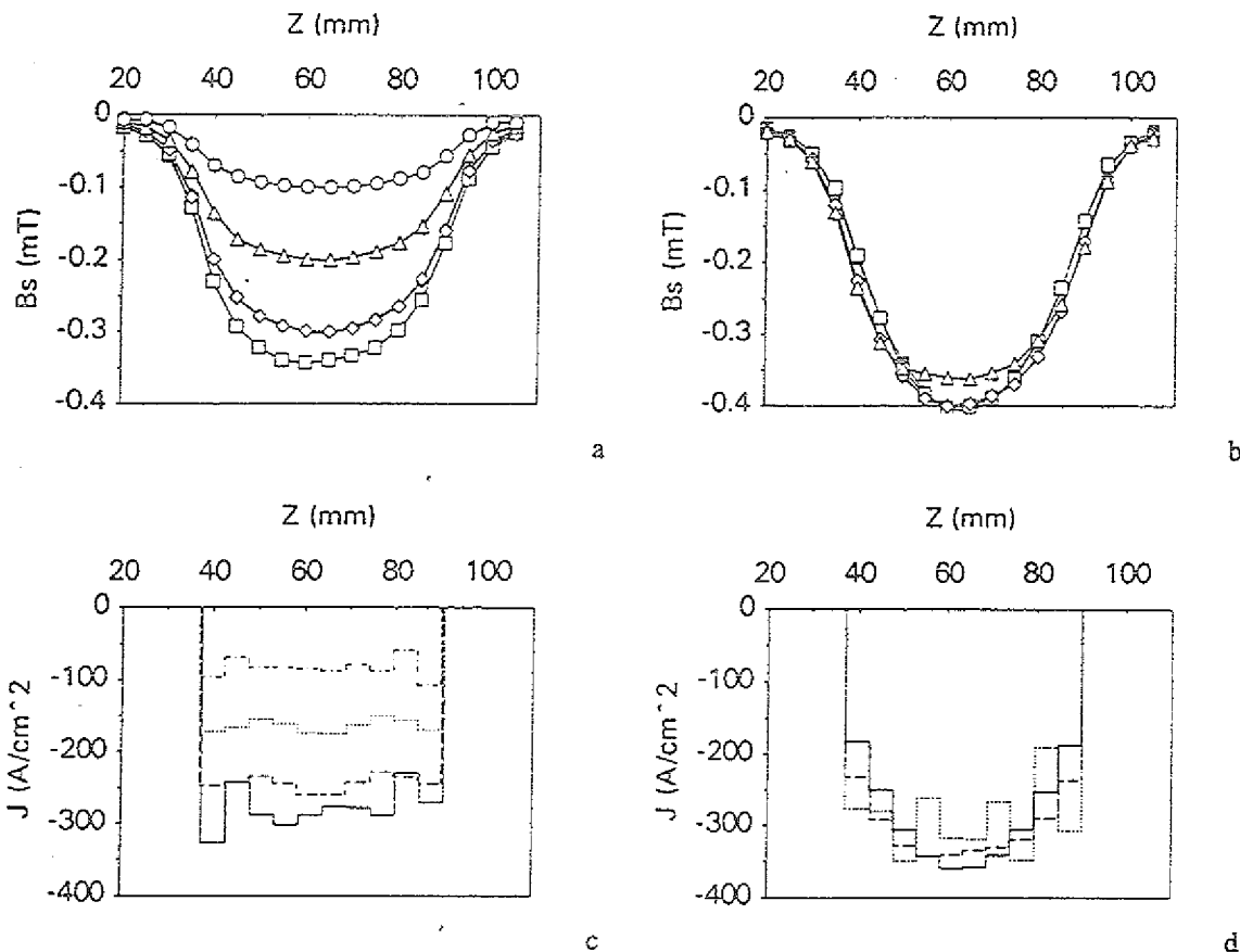
Abb. 98: Schirmungsfeldprofile und davon abgeleitete Stromdichtenprofile für das LPPS-Rohr mit \text{BaTiO}_3 Diffusionsbarriere, gemessen bei 20 K. (a,c) O, strichpunktiert: 0,1 mT; \Delta , punktiert: 0,2 mT; \diamond , gestrichelt: 0,3 mT; o, durchgezogen: 0,4 mT. (b,d) \Delta , punktiert: 0,5 mT; \diamond , gestrichelt: 0,7 mT; o, durchgezogen: 1,0 mT. Offene Symbole sind gemessen, geschlossene berechnet.
