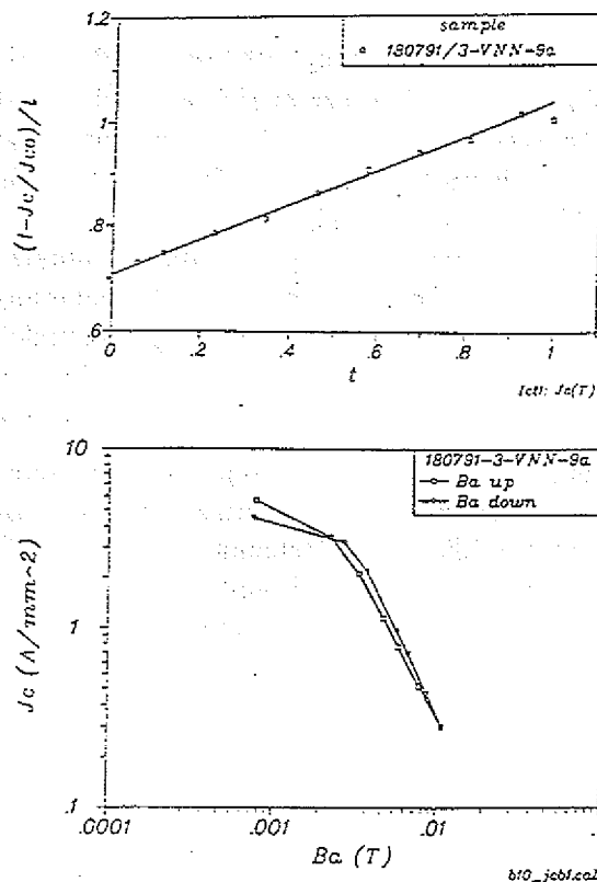
Abb. 36: Oben: Typische Darstellung der Temperaturabhängigkeit der kritischen Stromdichte für YBaCuO auf Ni 200. J_{c0} = 1340 \text{ A/cm}^2 und T_c = 87 \text{ K} . Unten: Typische Magnetfeldabhängigkeit der kritischen Stromdichte bei 4 K für YBaCuO auf Ni 200.
