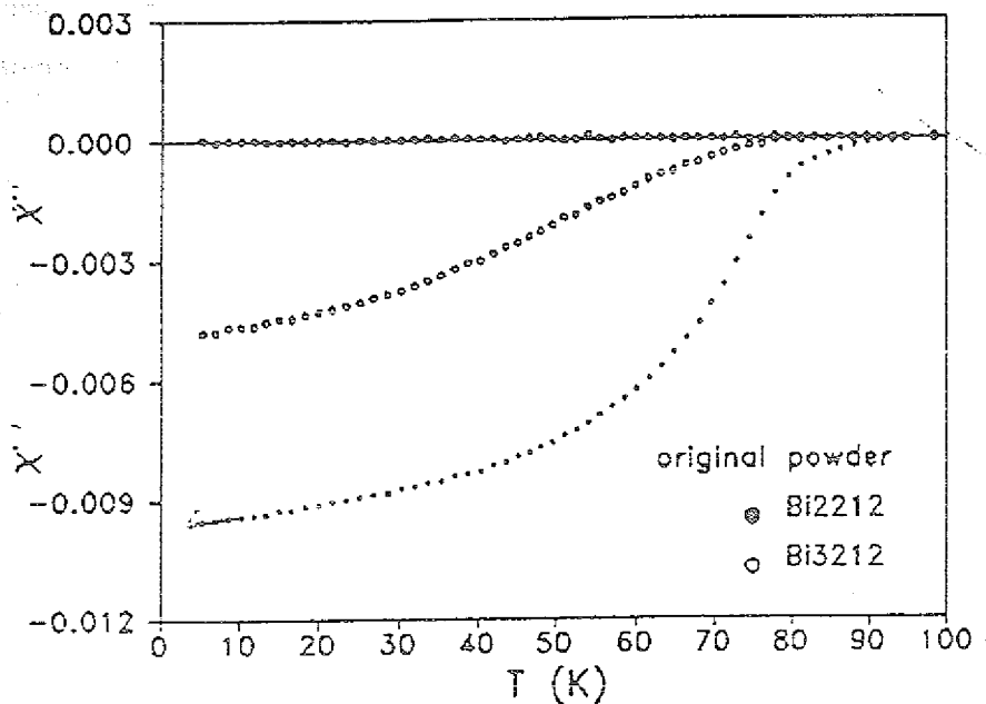
Abb. 60: AC-Suszeptibilität der verwendeten Spritzpulver.
