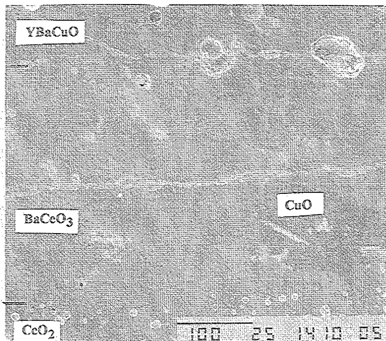
Abb. 45: Querschnitt der Grenzflächenreaktion zwischen \text{CeO}_2 und \text{YBa}_2\text{Cu}_3\text{O}_7 nach der Schmelzbehandlung. REM 200. Deutlich ist die etwa 300\ \mu\text{m} breite Reaktionszone zu erkennen (Bildmitte), bestehend aus \text{BaCeO}_3 , \text{CuO} und 211.
