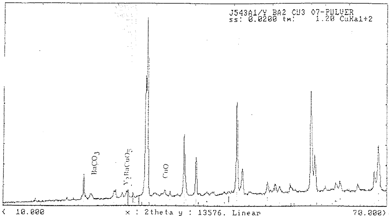
Abb. 23: Röntgenbeugungsdiagramm des gesinterten, für die weiteren Versuche verwendeten YBa 2 Cu 3 O 7 -Spritzpulvers. Cu-K α Strahlung.
