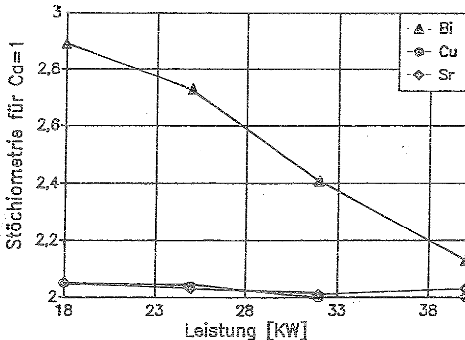
Abb. 66: Zusammenhang zwischen Leistung und Schichtstöchiometrie (normiert auf Calcium = 1). Die Variationen erfolgten ausgehend von dem als Standard gewählten Parameter: 32 kW Leistung; 300 mm Abstand; 200 mbar Argon Kammerdruck; 40 SLPM Argon, 50 SLPM Helium.
