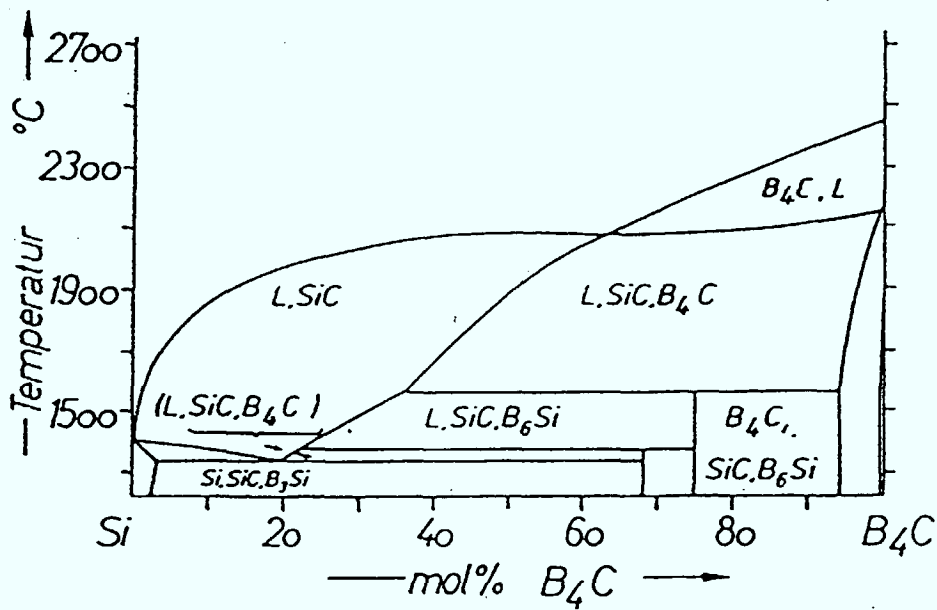
Bild 2.11: Berechneter Temperatur-Konzentrations-Schnitt im System B-C-Si von Si bis \text{B}_{12}\text{C}_3 nach /132/.
