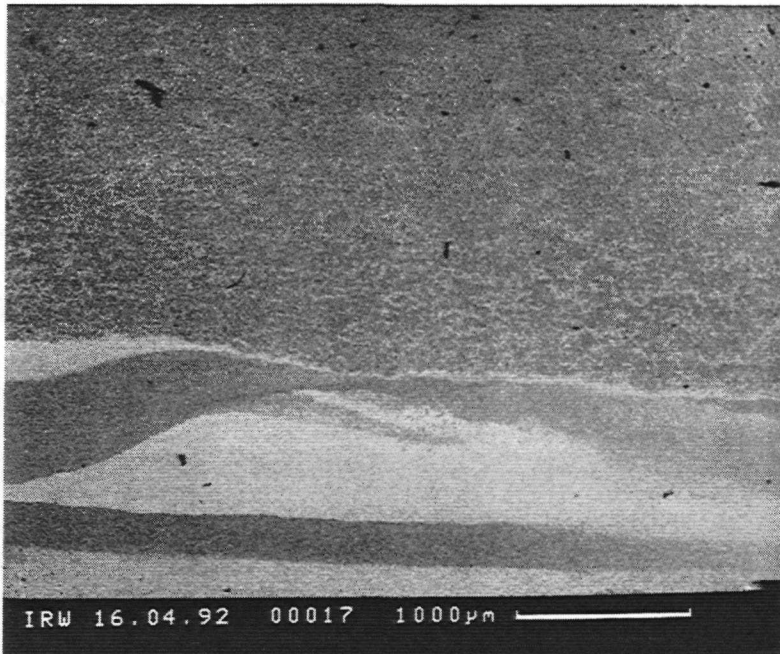
Bild 4.1: Füge-naht-Bruchfläche einer mit Si+Al-Sputterschichten gefügten Probe. Im unteren Bereich des Bildes (Streifen) wurden durch EDAX-Analyse Agglomerate höherer Al-Konzentration festgestellt.
