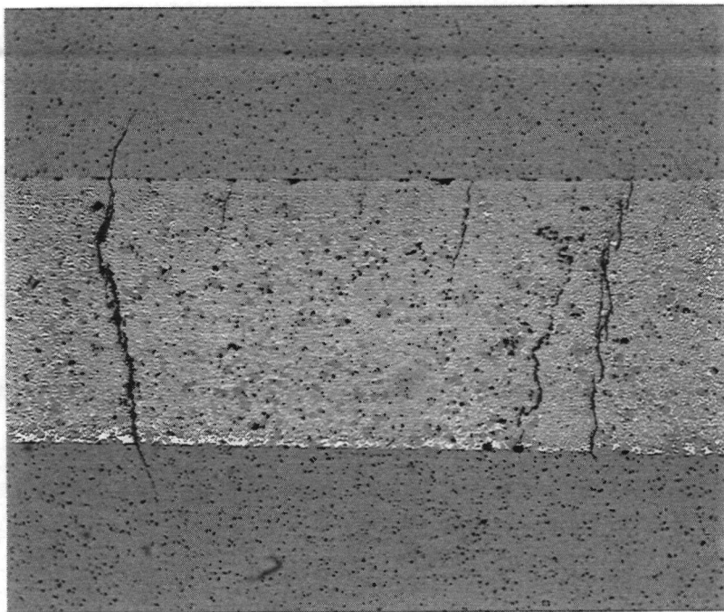
Bild 4.24: Fügenähte aus den Experimenten mit heißgepreßten Pulvermischungen aus Borcarbid, Silicium und Kohlenstoffzumischung.
