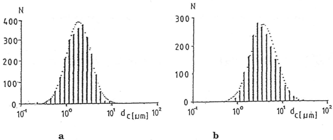
Bild 3.2: Parameter d_c in Histogrammform a) für SiC-HD und b) für SSiC; Gaußverteilung gestrichelt eingezeichnet.
