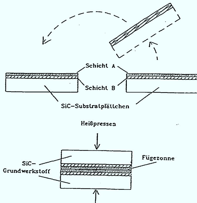
Bild 3.8: Schematische Darstellung des Heißpressens der beschichteten \alpha -SiC-Substrate.
