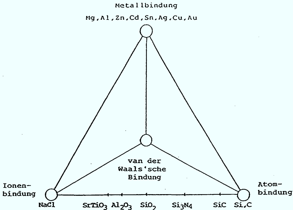
Bild 2.4: Darstellung der Übergänge der vier Bindungstypen mit Hilfe eines Tetraeders /28/.
