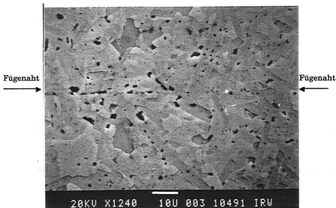
Bild 4.11: Fügenaht aus Si- und C-Sputterschichten, angeätzt mit Murakami-Lösung, um das Zusammenwachsen der Körner sichtbar zu machen.
