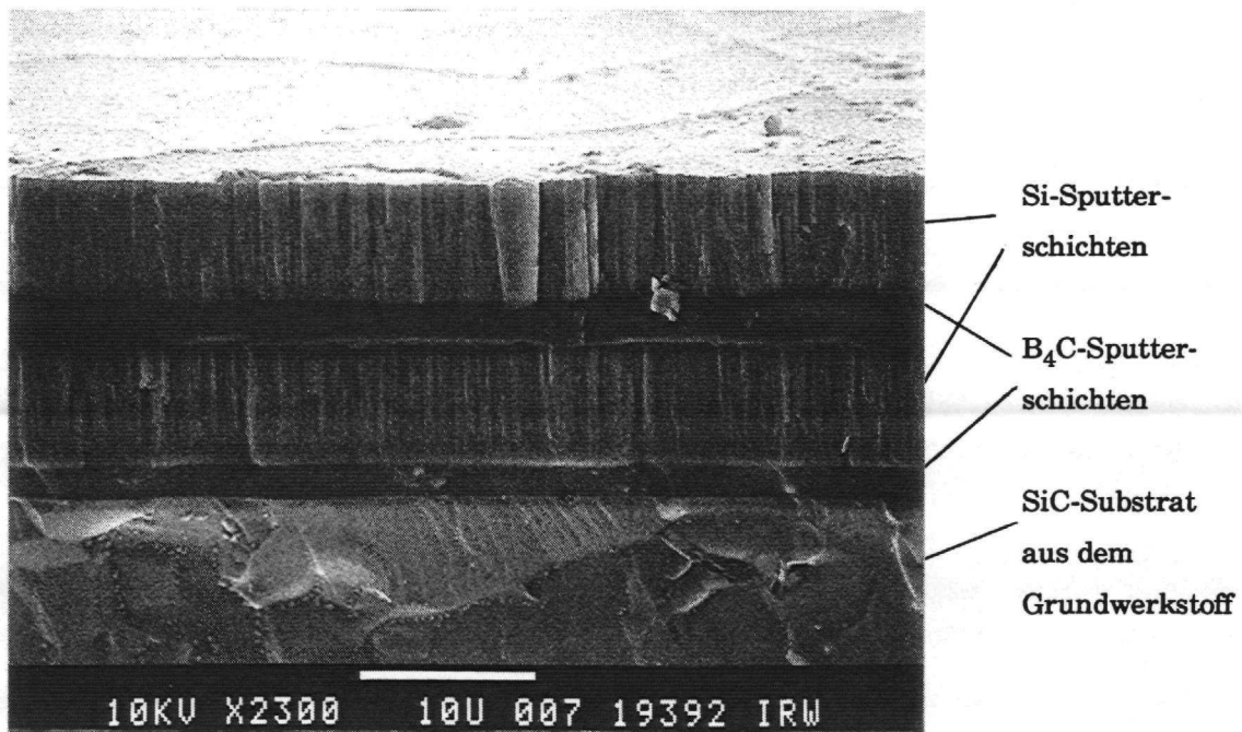
Bild 3.7: Bruchfläche durch vier abwechselnd aufeinander gesputterte Schichten von B 4 C und Si auf einem \alpha -SiC-Substrat.
