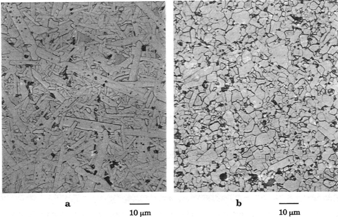
Bild 3.1: Korngrenzengeätzte keramographische Schiffe
