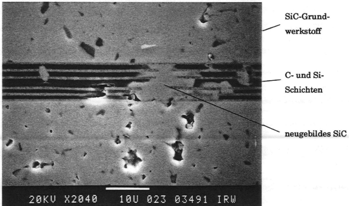
Bild 4.9: Stellenweise Bildung von SiC in den heißgepreßten Schichten.
