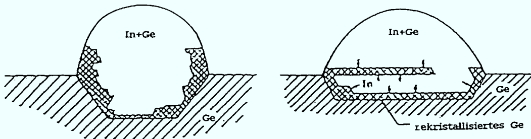
Bild 2.3: Veränderungen an der Grenzfläche fest/flüssig. Benetzung von Germanium durch Indium /21/.
