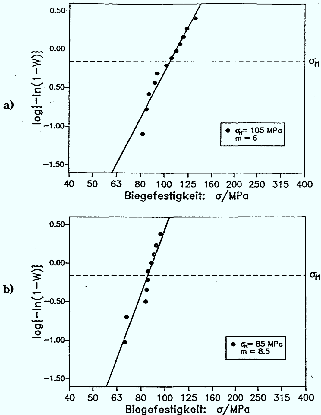
Bild 4.20: 4-Punkt-Biegefestigkeiten der mittels Si-Aufdampfschicht und C-Sputterschicht gefügten Proben.
