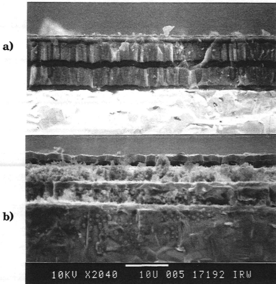
Bild 4.10: Bruchflächen von Silicium- und Kohlenstoff-Schichten. a) vor der Glühung, b) nach der Glühung (porös).
