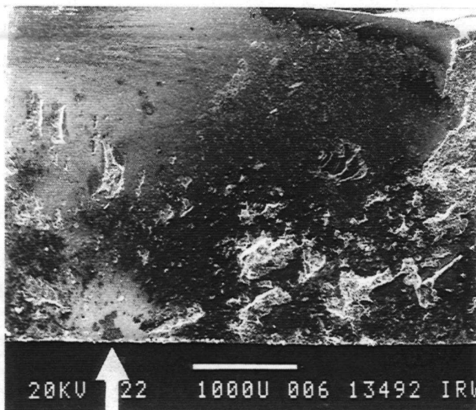
Bild 4.2: Fügenaht-Bruchfläche einer mit B_4C+Si -Sputterschicht gefügten Probe. Hier wurde der Bruch ausnahmsweise durch einen Fehler in der Fügenaht initiiert (Pfeil).
