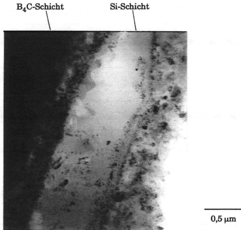
Bild 4.5: TEM-Aufnahme der bei 1450^\circ C heißgepreßten B_4C - und Si-Schichten. Die Si-Schicht, die als amorph identifiziert wurde, ist auf ca. 1/4 der ursprünglichen Schichtdicke zusammengepreßt.
