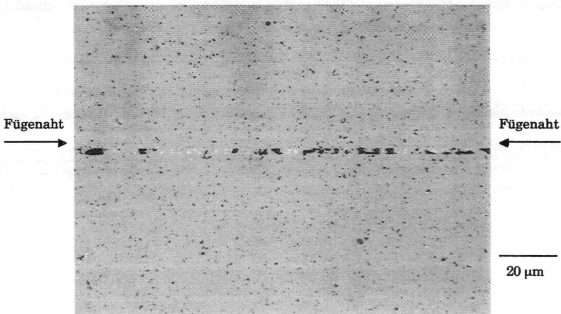
Bild 4.15: Porosität in der Fügezone einiger Proben.
