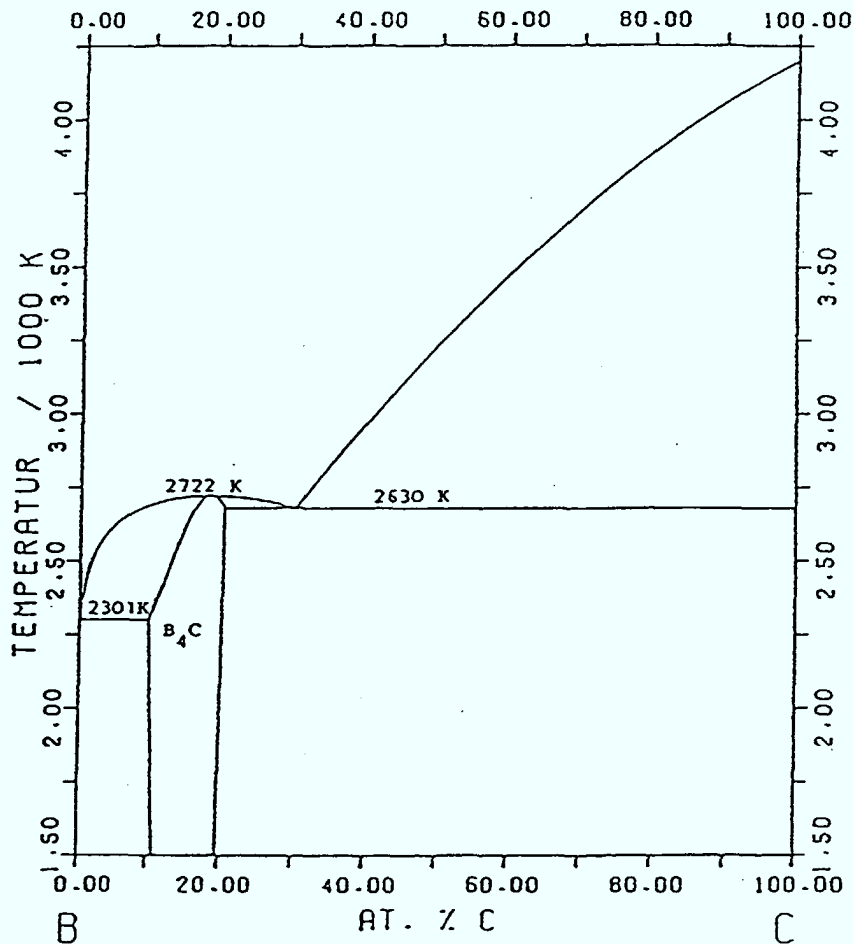
Bild 2.9: Das binäre System B-C nach /132/.
