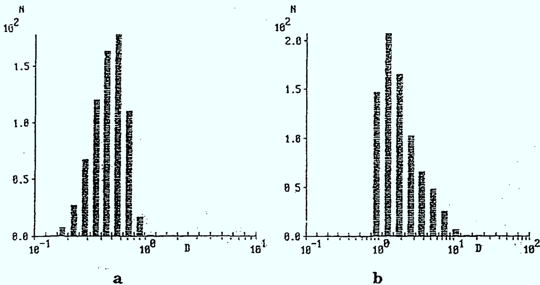
Bild 3.3: Korngrößenverteilung (Parameter d_c ) in Histogrammform nach Herstellerangaben a) für Borcarbid- und b) für Siliciumpulver.
