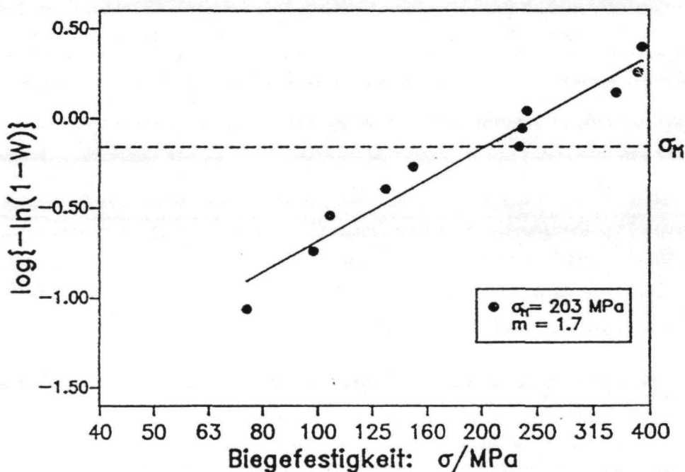
Bild 4.12: Raumtemperaturfestigkeit von Biegebruchstäbchen aus der mittels Si- und C-Sputterschichten gefügten Proben. Fügebedingungen: T = 1450^{\circ}\text{C} , P = 30\text{ MPa} , t = 0.5\text{ h} .
