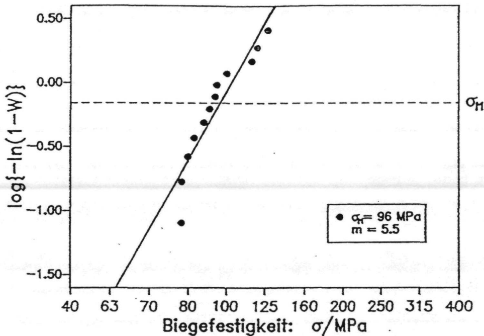
Bild 4.19: Raumtemperaturfestigkeit der mittels Si-Folie und C-Sputterschicht gefügten SiC-Proben. ( T=1650^{\circ}\text{C} , P=30\text{ MPa} , t=30\text{ Min.} )
