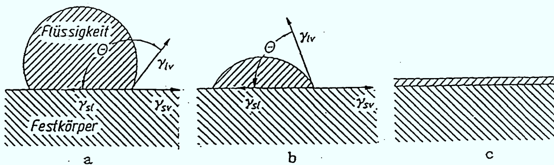
Bild 2.2: Beispiele für das Benetzungsverhalten von Flüssigkeiten auf Festkörpern a) nicht benetzend ( \theta > 90^\circ ), b) benetzend ( \theta < 90^\circ ) und c) vollständig benetzend ( \theta = 0 ) /16/.
