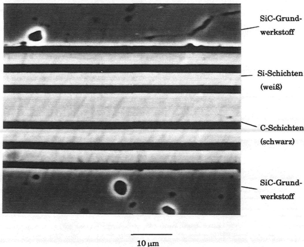
Bild 4.7: Mikrosondeaufnahme (Absorberbild-invertiert) der heißgepreßten, aber nicht miteinander reagierten Si- und C-Sputterschichten ( T = 1370^{\circ}\text{C} , P = 30\text{ MPa} , t = 0.5\text{ h} ).
