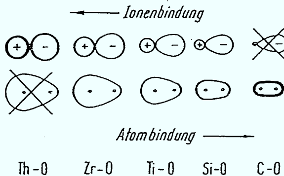
Bild 2.5: Schematische Darstellung des Übergangs zwischen Atom- und Ionenbindung /16/.
