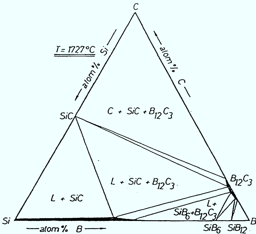
Bild 2.10: Berechnete Phasenfeldaufteilung bei 1727^\circ\text{C} im System B-C-Si nach /132/.
