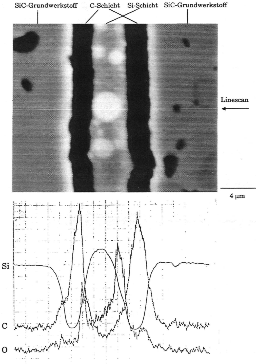
Bild 4.8: Mikrosondeaufnahme (Absorberbild-invertiert).
