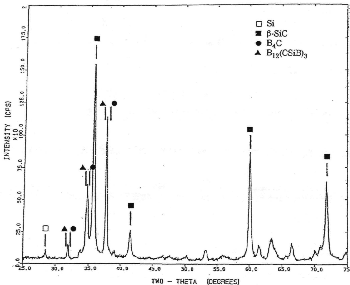
Bild 4.21: Diffraktometrische Aufnahme der Reaktionsprodukte. Die neugebildete Phase ( B_4C_{(1-x)}Si_x ) liegt zwischen B_4C und B_{12}(CSiB)_3 aus JCPDS-Datei 19-178.
