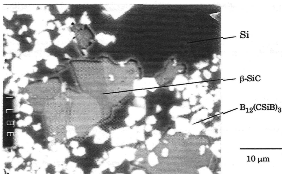
Bild 4.23: Mikrosondaufnahme (Absorberbild) zur Unterscheidung der Phasen \beta\text{-SiC} (grau), B_{12}(\text{CSiB})_3 (weiß) und freies Silicium (schwarz).
