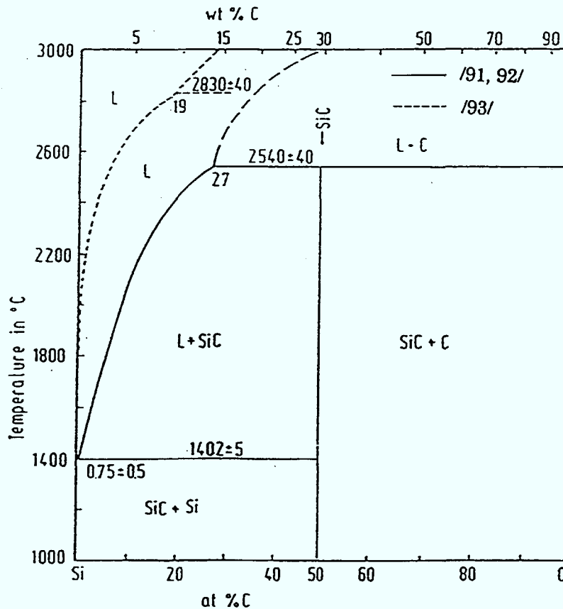
Bild 2.7: Si-C-System nach /94/.
