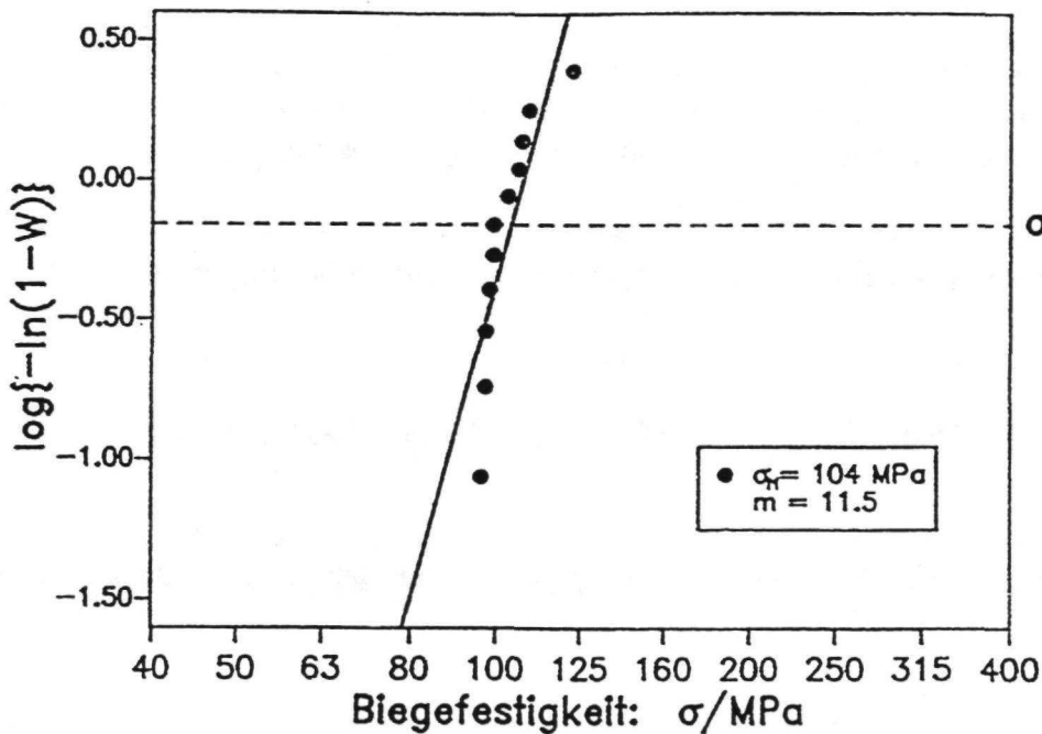
Bild 4.14: Hochtemperaturfestigkeit (Testtemperatur=1370° C) einer bei 1650° C mittels Si- und C-Sputterschichten gefügten Probe. (Fügebedingungen: T = 1650^\circ \text{C} , P = 30 \text{ MPa} , t = 0.5 \text{ h} )
