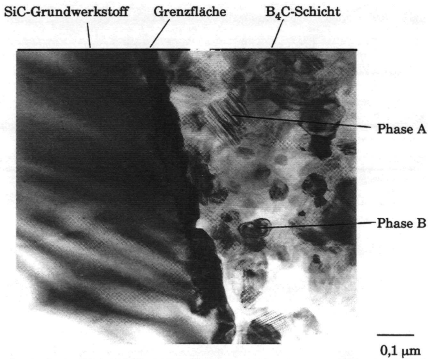
Bild 4.6: TEM-Aufnahme der Grenzfläche SiC-Grundwerkstoff/ B_4C -Schicht mit einer dünnen Si-Zwischenschicht von 0,5\ \mu m .
