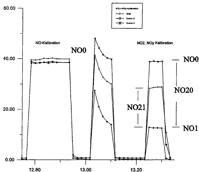
Abb 6 : Beispiel einer Eichung. Auf der x-Achse die Zeit, y-Achse Meßsignal der CLD's in ppb. Im Zeitraum von 12.79-12.95 findet die NO-Kalibration der CLD's statt. Von 13.00- 13.10 sieht man, daß das Kalibrationsgas noch nicht vollständig durch die Leitung gepumpt wurde und das Einstellen der Konzentration im Mischsystem noch nicht beendet ist. Ab 13.25 die \text{NO}_2 bzw. \text{NO}_y Kalibration. Der NO-CLD sieht das kleinste Signal ( \text{NO}_{\text{gpt}} ). Der CLD mit Photolysekonverter mißt \text{NO}_x , wobei die Konversionsrate für \text{NO}_2 ca. 60% beträgt. Der CLD mit Goldrohrkonverter mißt aufgrund der hohen Konversionsrate >99% das gesamte \text{NO}_x .
