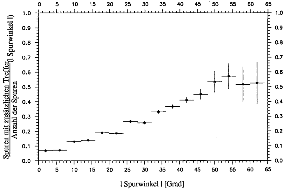
Abbildung 3.9: Zusatztreffer durch Berücksichtigung von Zellkreuzungen als Funktion des Winkels
