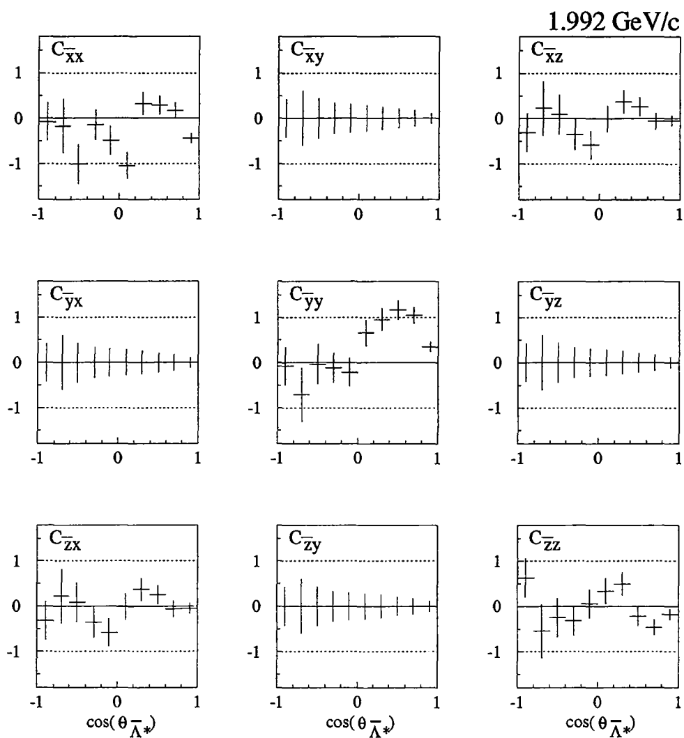
Abbildung 5.31: Daten: Intrinsisch korrigierte Spinkorrelationen als Funktion von \cos(\theta_{\Lambda^*}^-) für p_{\bar{p}} = 1.992 GeV/c
