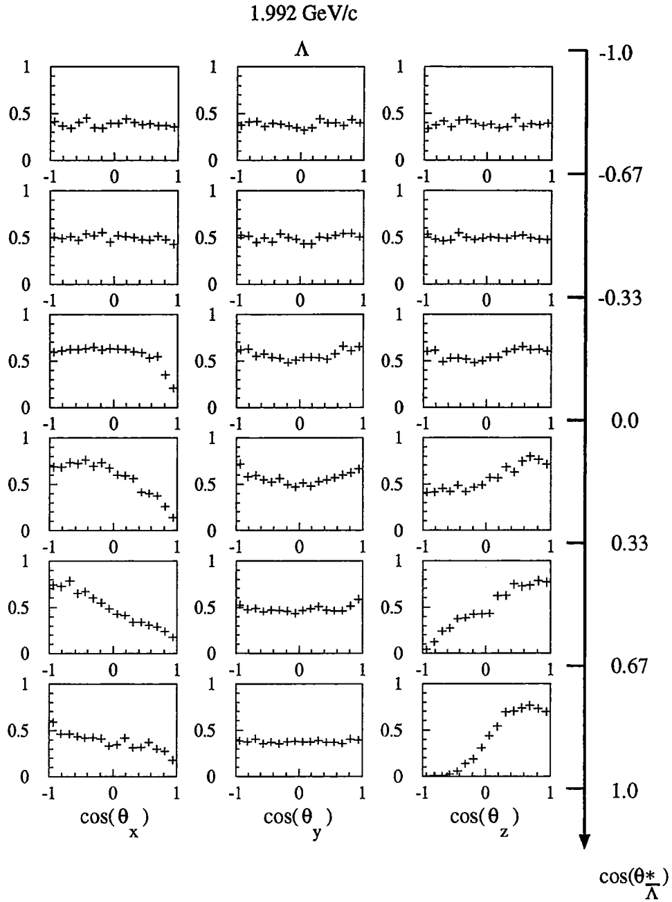
Abbildung 5.9: Monte-Carlo Daten ( p_{\bar{p}}=1.992 GeV/c): Akzeptanzen \mathcal{A}_i(\cos(\theta_{\Lambda}^*), \cos(\theta_i)) mit i = x, y, z in sechs Bereichen von \cos(\theta_{\Lambda}^*)
