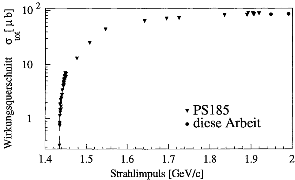
Abbildung 4.13: Totaler Wirkungsquerschnitt \sigma_{tot} als Funktion des Strahlimpulses aus verschiedenen Messungen der PS185-Kollaboration (incl. der Ergebnisse dieser Arbeit)
