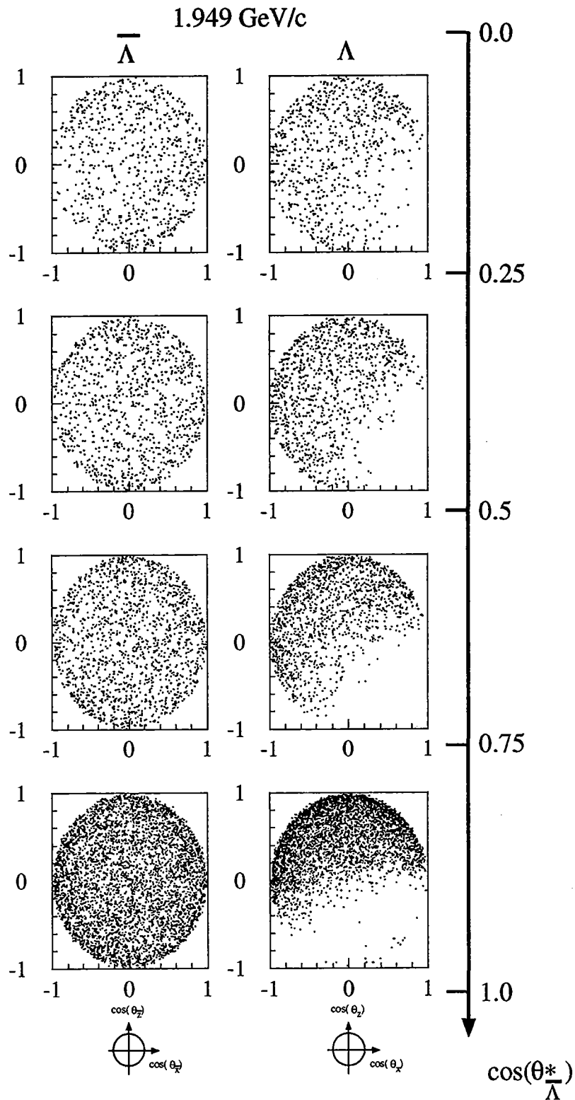
Abbildung 5.6: Daten ( p_{\bar{p}}=1.949 GeV/c): Verteilung der Zerfallsantiprotonen und -protonen im \bar{\Lambda}(\Lambda) -Ruhesystem auf der Produktionsebene der \bar{\Lambda}\Lambda -Hyperonen für den \theta_{\Lambda^*} -Vorwärtsbereich
