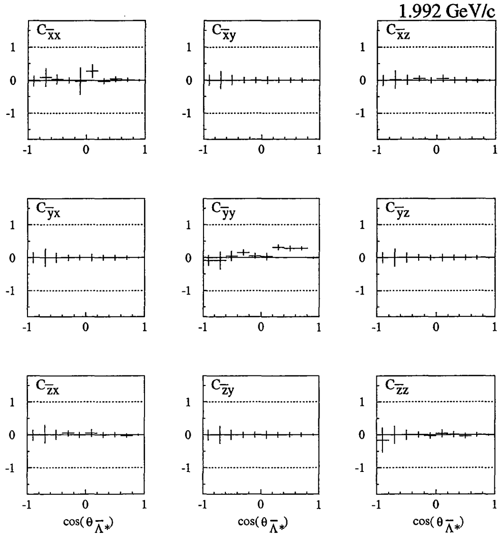
Abbildung 5.27: Experimentelle Monte-Carlo Daten: Korrigierte Spinkorrelationen als Funktion von \cos(\theta_{\Lambda^*}^-) für p_{\bar{p}} = 1.992 \text{ GeV}/c
