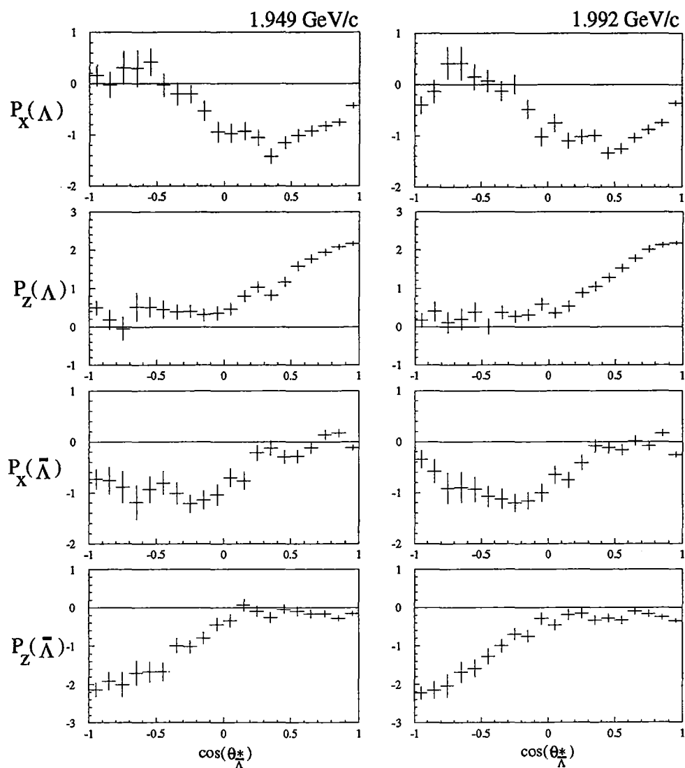
Abbildung 5.18: Daten:
