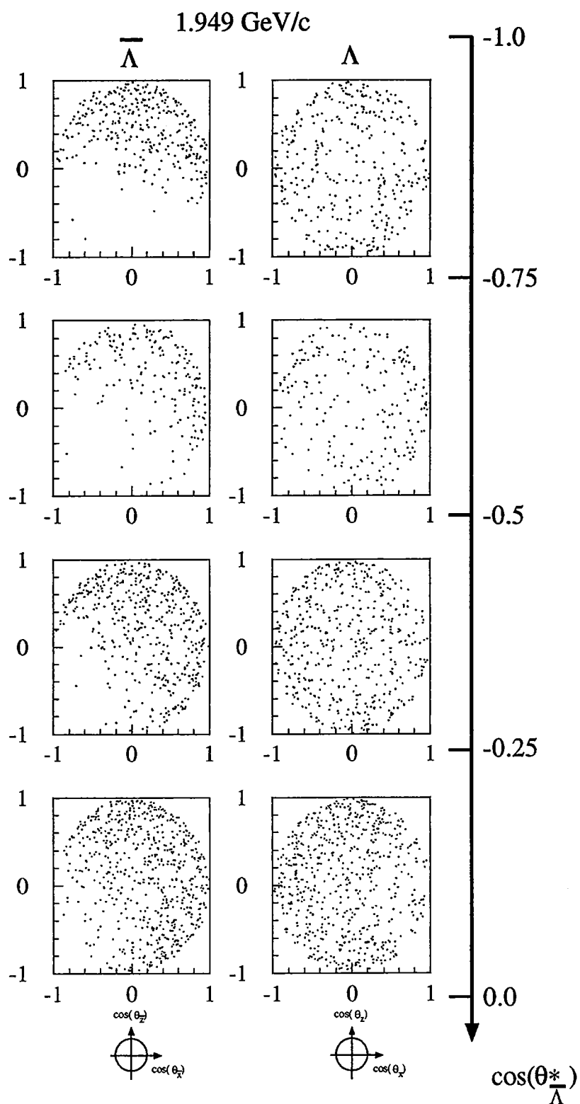
Abbildung 5.5: Daten ( p_{\bar{p}}=1.949 GeV/c):
