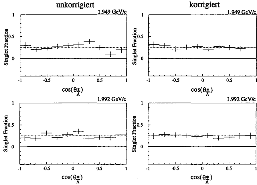
Abbildung 5.32: Monte-Carlo Daten: Singlet Fraction als Funktion von \cos(\theta_{\Lambda}^*) für die beiden Strahlimpulse von 1.949 GeV/c und 1.992 GeV/c
