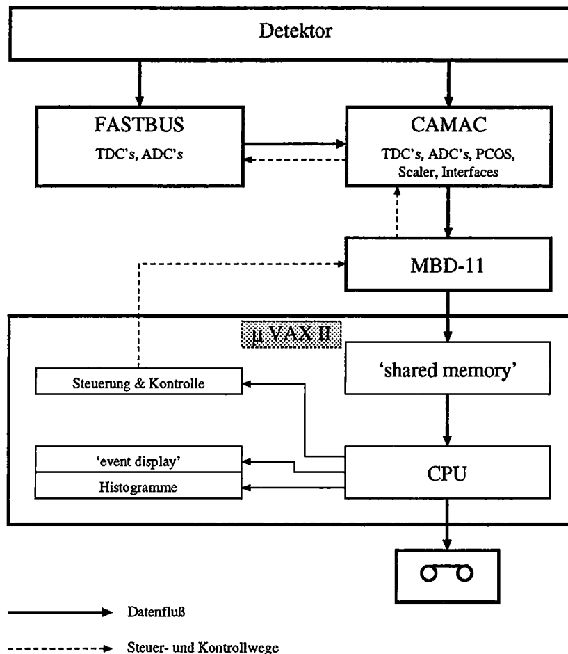
Abbildung 2.3: Das Datenaufnahme-System
