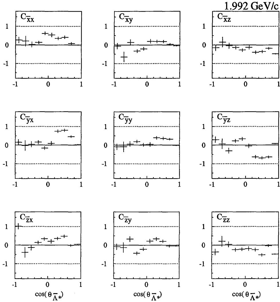
Abbildung 5.23: Experimentelle Monte-Carlo Daten: Unkorrigierte Spinkorrelationen als Funktion von \cos(\theta_{\bar{\Lambda}^*}) für p_{\bar{p}} = 1.992 GeV/c
