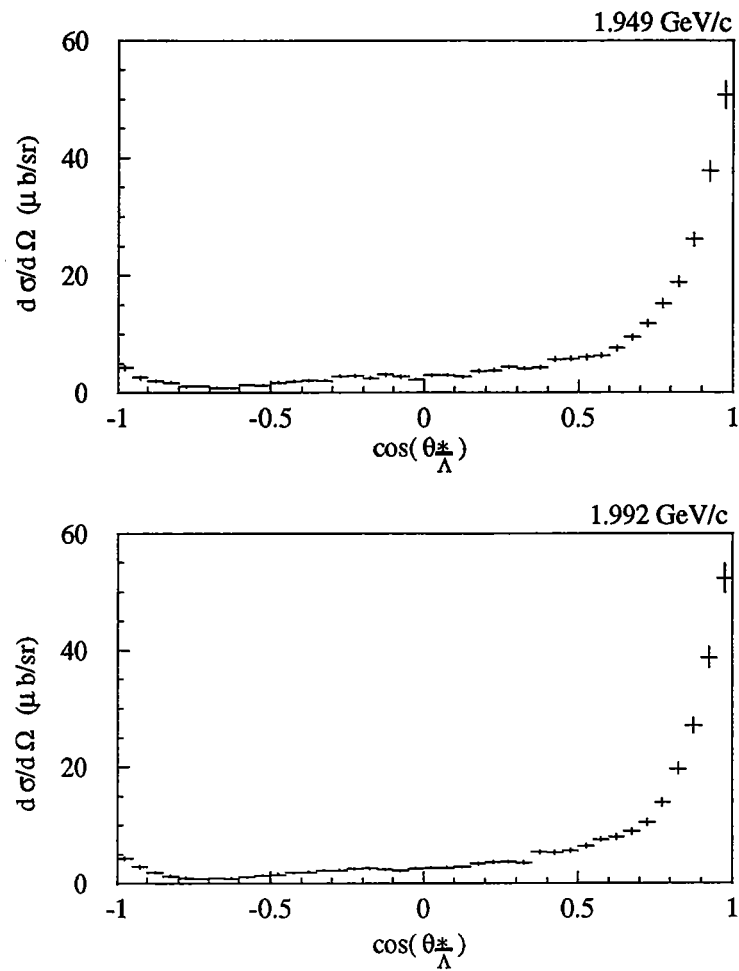
Abbildung 4.14: Differentieller Wirkungsquerschnitt (korrigiert) als Funktion von \cos(\theta_{\Lambda}^*) für die beiden Strahlimpulseinstellungen von 1.949 GeV/c und 1.992 GeV/c
