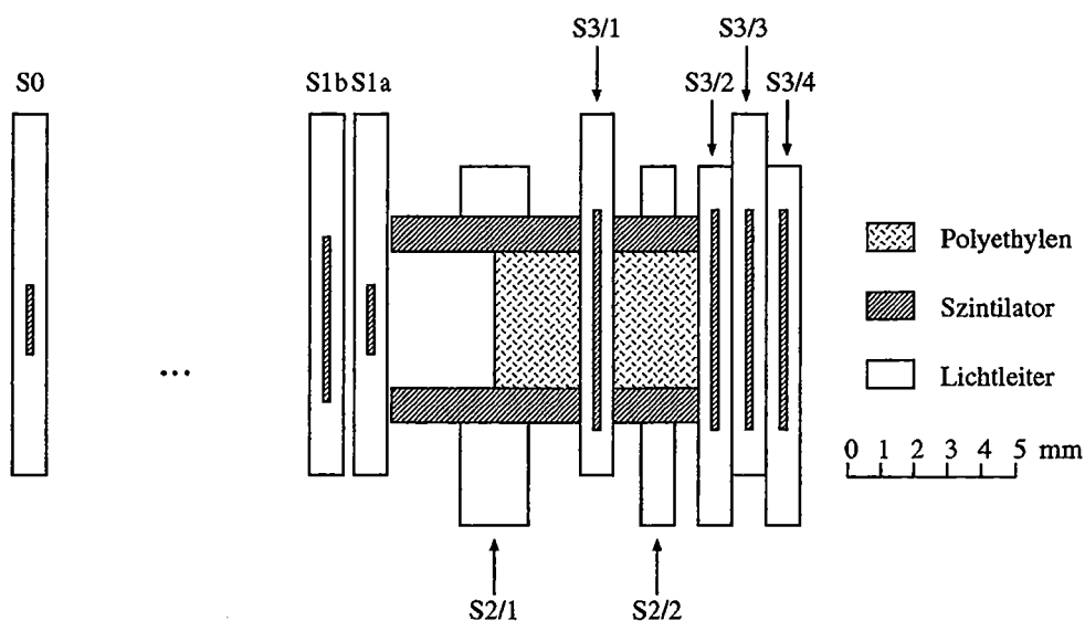
Abbildung 2.2: Die Targetregion
