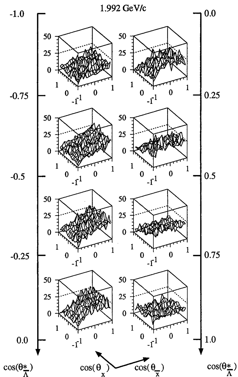
Abbildung 5.11: Monte-Carlo Daten ( p_{\bar{p}}=1.992 GeV/c): Akzeptanzfläche \mathcal{A}_{\bar{x},x}(\cos(\theta_{\bar{A}}^*), \cos(\theta_{\bar{x}}), \cos(\theta_x)) in acht Bereichen von \cos(\theta_{\bar{A}}^*)
