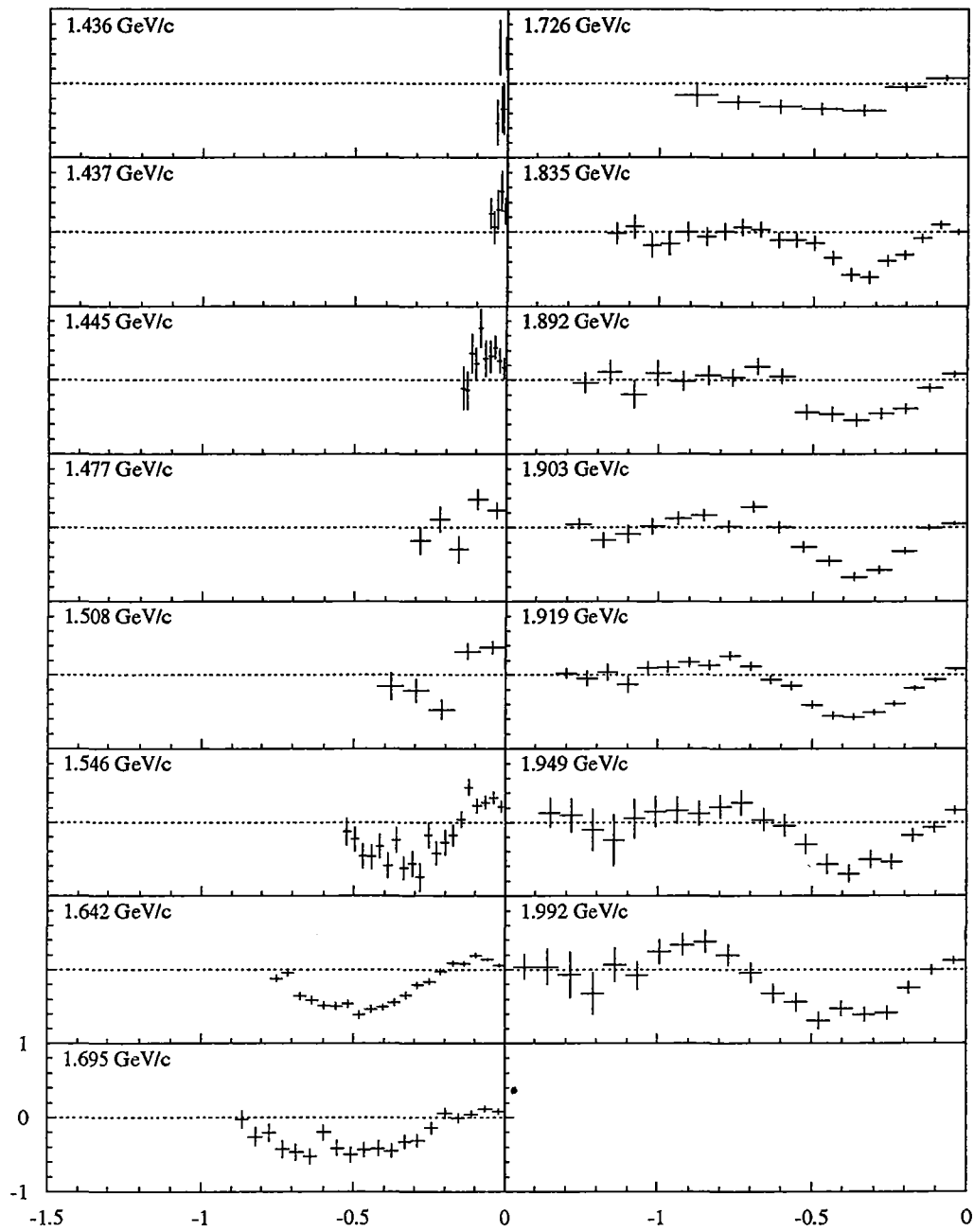
Abbildung 5.21: Daten:
