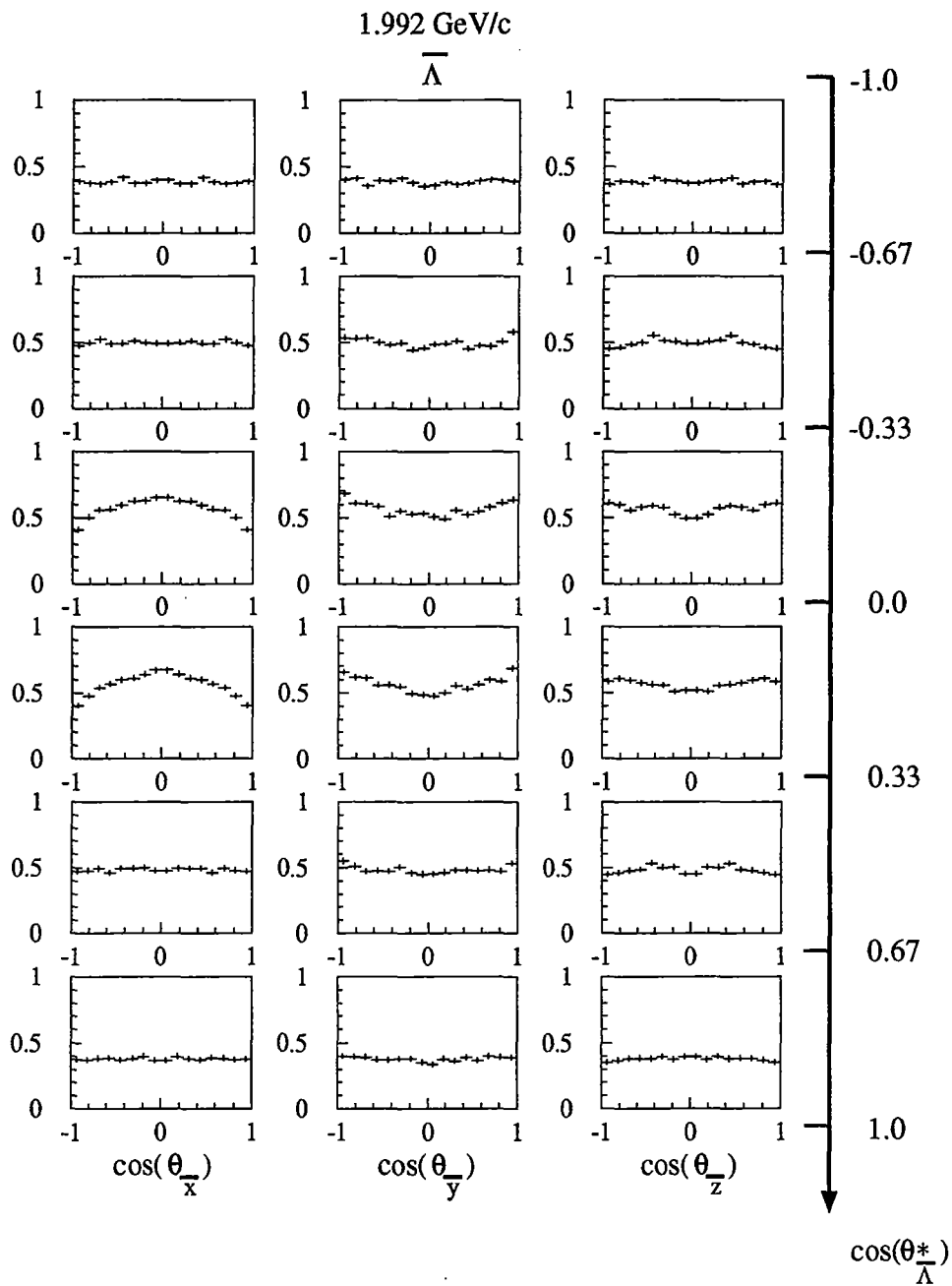
Abbildung 5.14: Monte-Carlo Daten ( p_{\bar{p}}=1.992 GeV/c) (symmetrisiert): Akzeptanzen \mathcal{A}_i(\cos(\theta_{\bar{\Lambda}}^*), \cos(\theta_i)) mit i = x, y, z in sechs Bereichen von \cos(\theta_{\bar{\Lambda}}^*)
