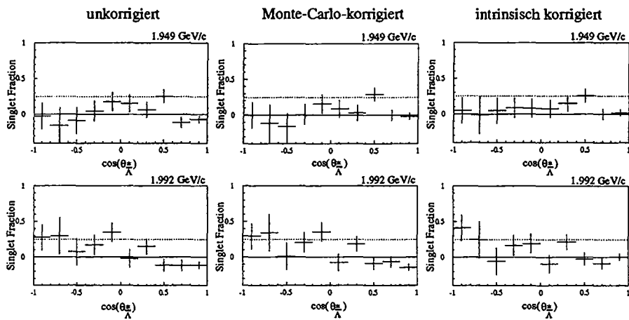
Abbildung 5.34: Daten:
