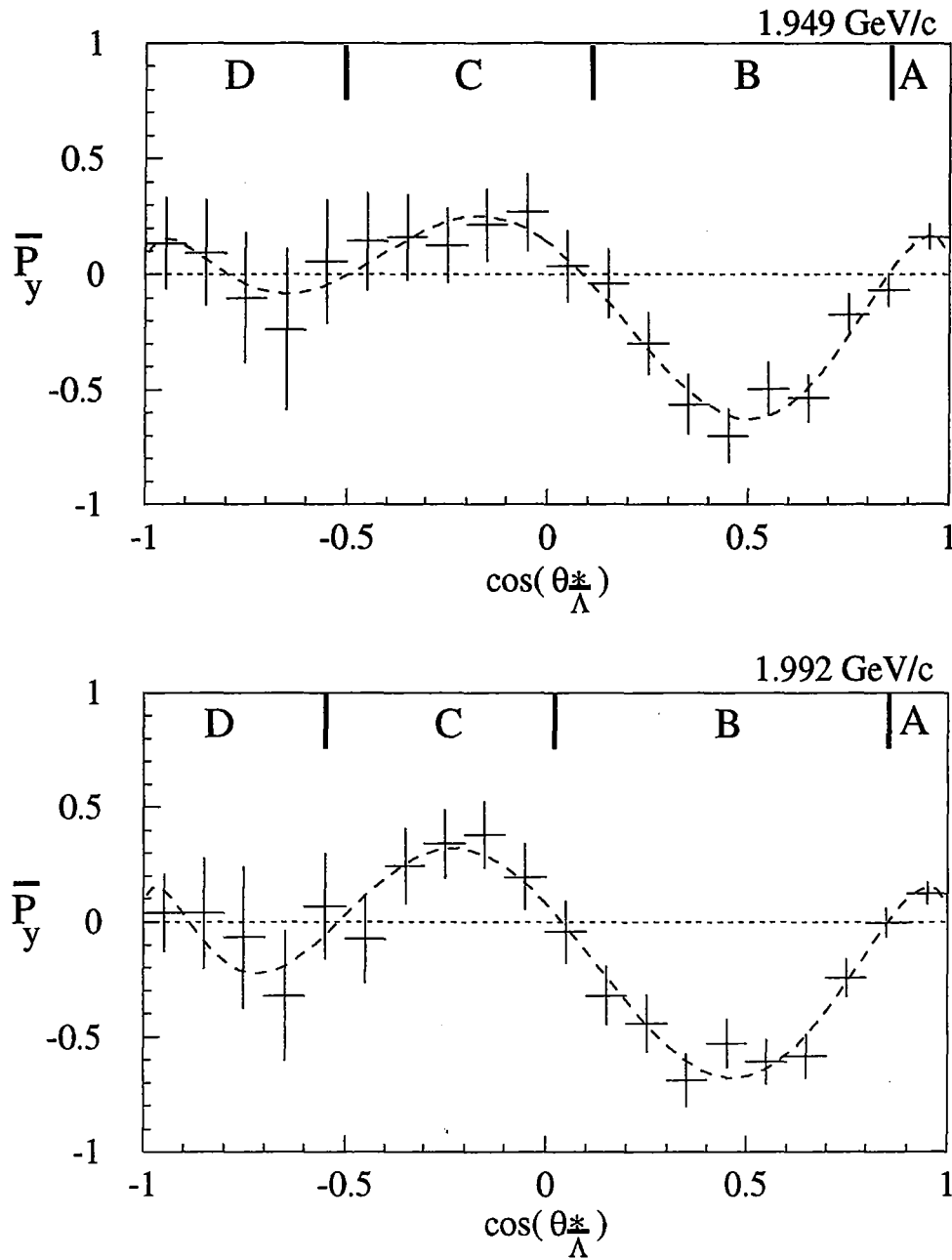
Abbildung 5.20: Daten:
