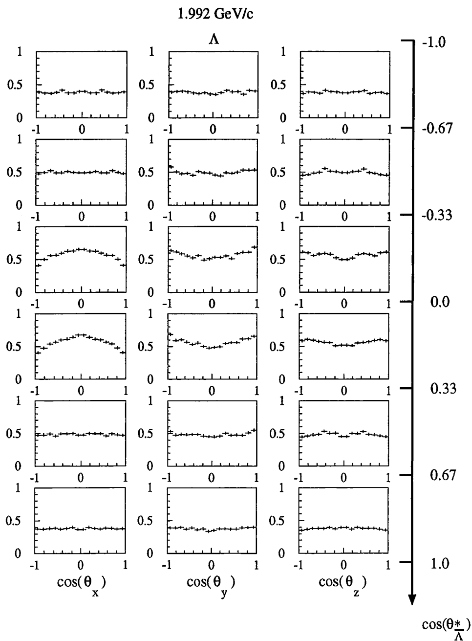
Abbildung 5.13: Monte-Carlo Daten ( p_{\bar{p}}=1.992 GeV/c) (symmetrisiert): Akzeptanzen \mathcal{A}_i(\cos(\theta_{\Lambda}^*), \cos(\theta_i)) mit i = x, y, z in sechs Bereichen von \cos(\theta_{\Lambda}^*)
