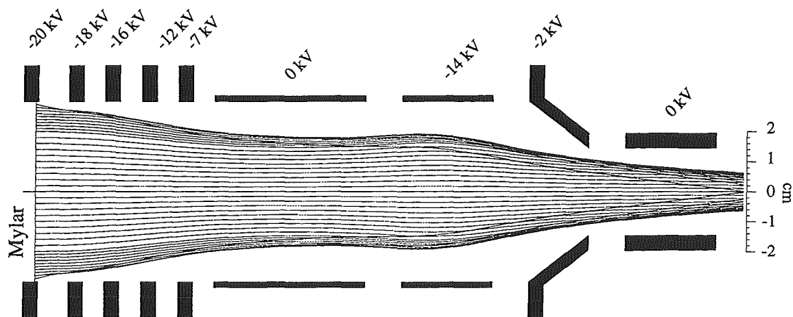
Abb. [2.11.]: Die Neuentwicklung der elektrostatischen Linse für den RFD-II Detektor
