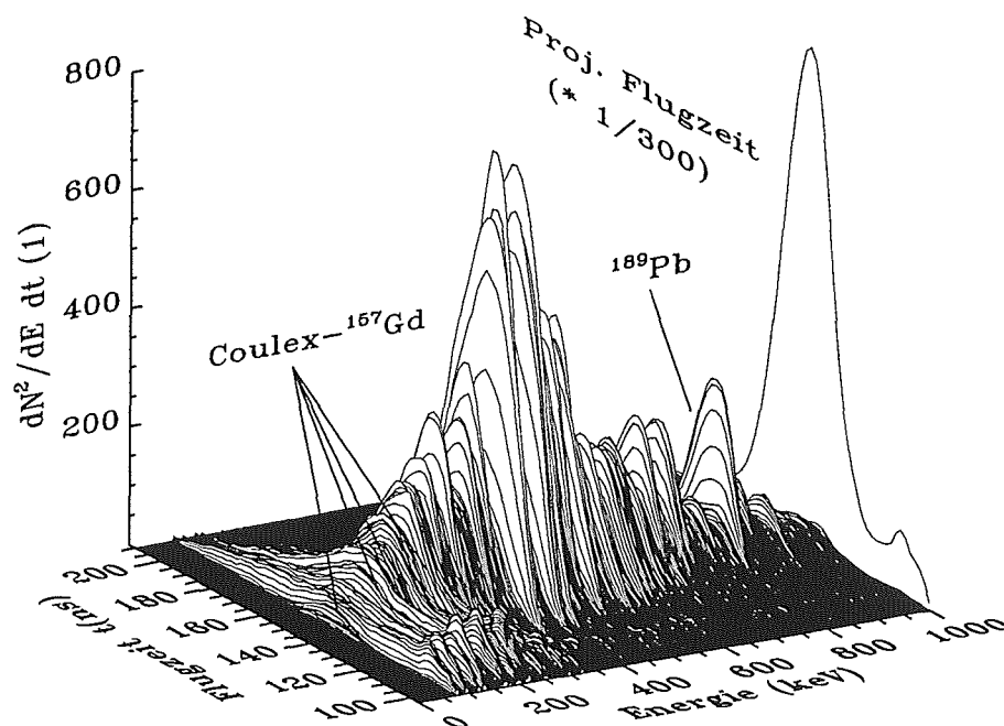
Abb. [3.6.]: Die gemessene E_\gamma -Flugzeitverteilung im Experiment an ^{189}\text{Pb}
