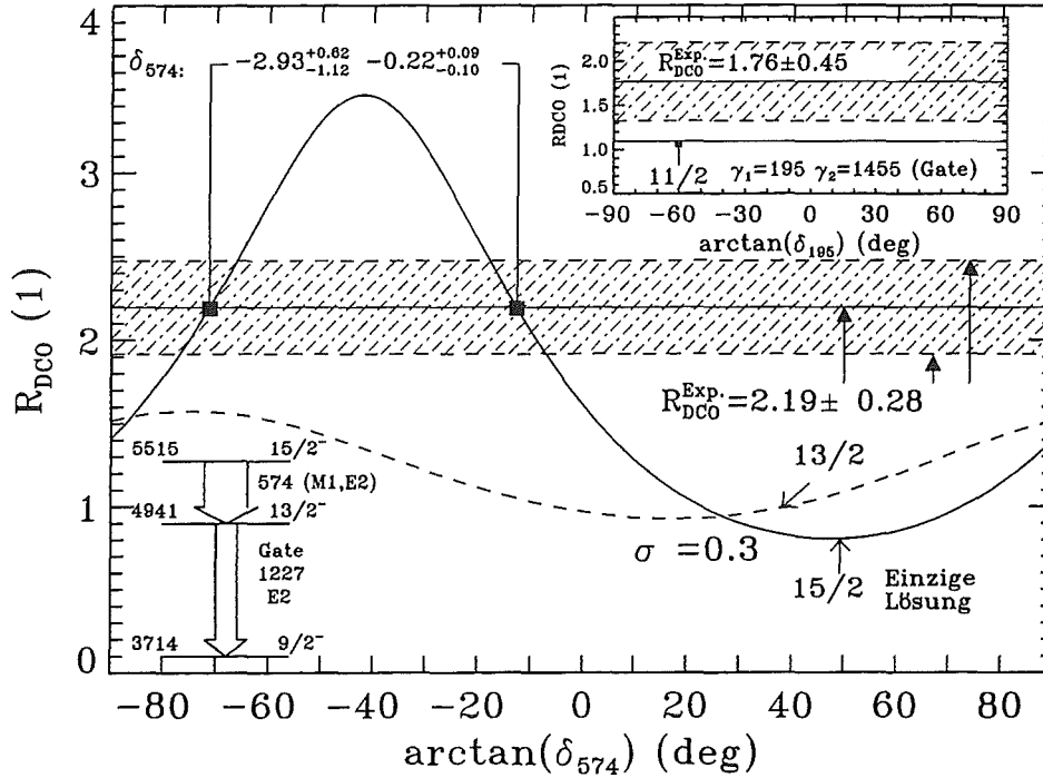
Abb. [3.41.]: Experimentelle und theoretische DCO-Verhältnisse für das 5515 \text{ keV} -Niveau von ^{57}\text{Ni}
