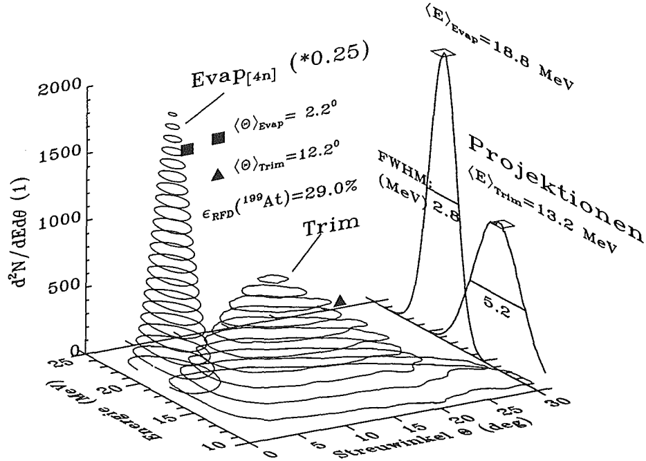
Abb. [3.22.]: Die Verteilung [d^2N/dE d\theta]_{199\text{At}}^{\text{Trim}} der transmittierten ^{199}\text{At} -Kerne, sowie [d^2N/dE d\theta]_{199\text{At}}^{\text{Evap}} aus ^{175}\text{Lu}(^{28}\text{Si}, 4n)^{199}\text{At} bei E_{\text{kin}}(^{28}\text{Si}) = 141.0 \text{ MeV} und d_{\text{Target}} = 1.0 \text{ mg/cm}^2
