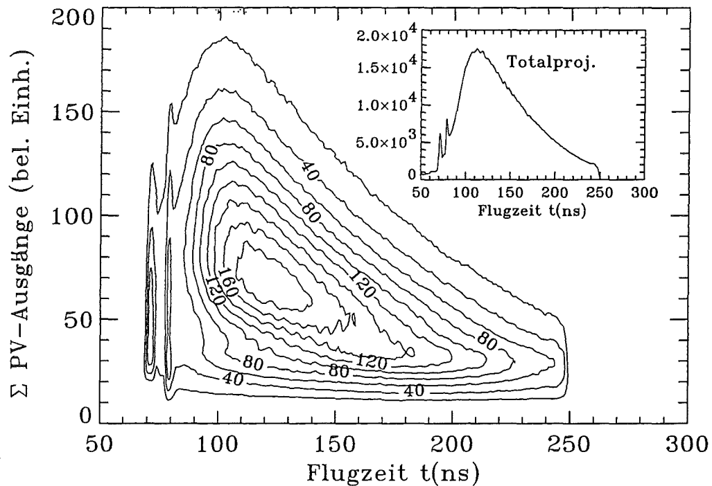
Abb. [3.31.]: Die Korrelation zwischen Flugzeit und Impulshöhe in den 18 Photovervielfachern des RFD's im ^{57}\text{Ni} Experiment
