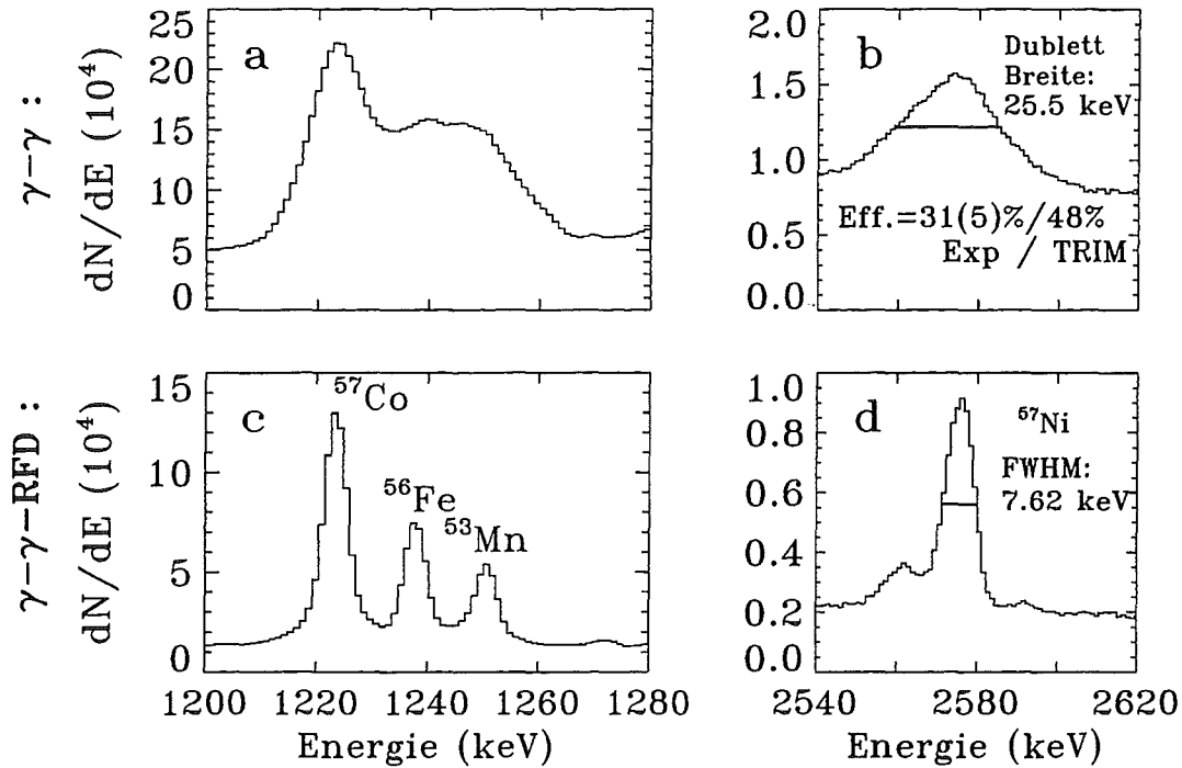
Abb. [3.34.]: Der Vergleich der gemessenen Linienbreiten für das ^{57}\text{Ni} -Experiment zwischen den \gamma - \gamma -Daten (ca. 70% nur mit mittleren |\vec{v}| dopplerkorrigiert) und den \gamma - \gamma -RFD Daten (individuelle Dopplerkorrektur)
