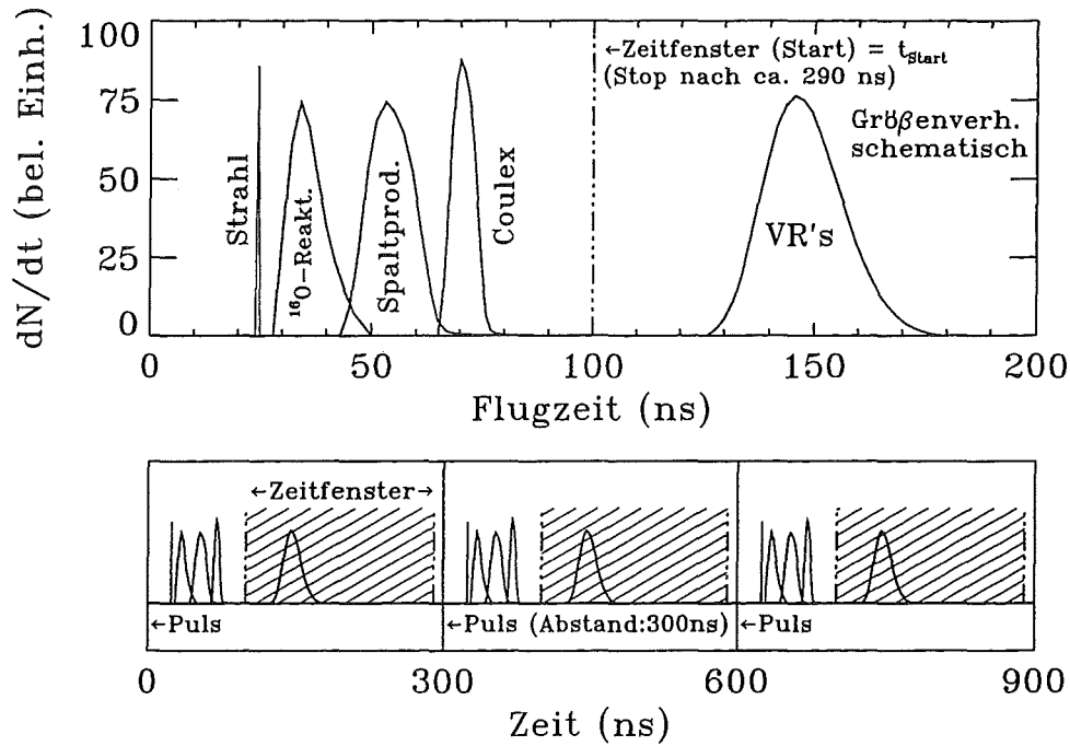
Abb. [2.17.]: (oben) Flugzeitverteilung (schematisch) der in Strahlrichtung gestreuten Teilchen im Experiment ^{36}\text{Ar} \rightarrow ^{157}\text{Gd} bei E_{kin}(^{36}\text{Ar}) = 173.0 \text{ MeV} , d_{\text{Target}} = 0.9 \text{ mg/cm}^2 und oxidiertem Target // (unten) Systematik der Strahlpulsung
