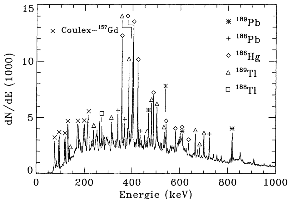
Abb. [3.9.]: Die Reaktionskanäle aus ^{36}\text{Ar} \rightarrow ^{157}\text{Gd} in der Energieprojektion der \gamma -RFD Matrix
