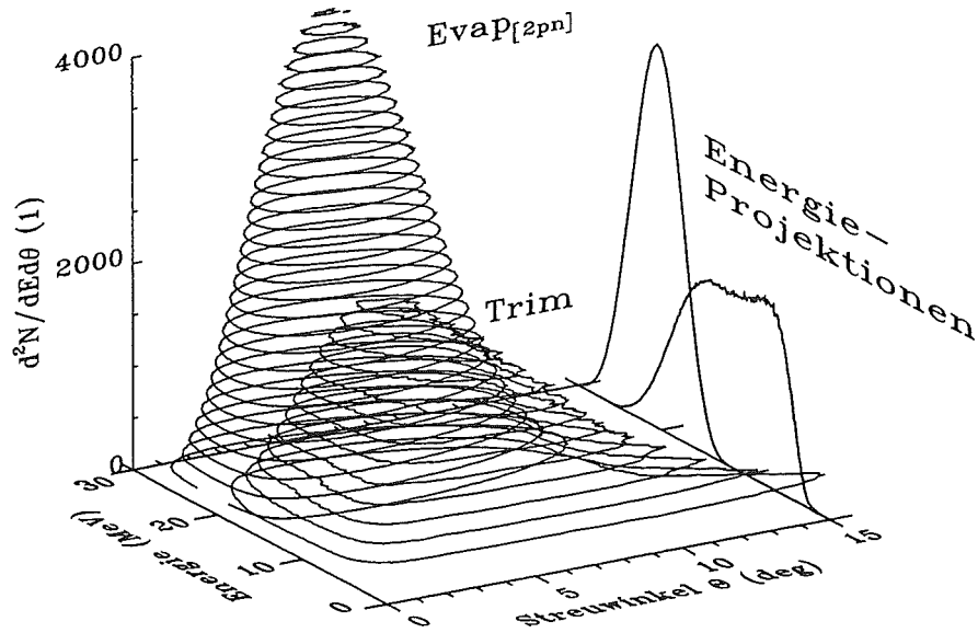
Abb. [2.5.]: Die Verteilungen [d^2N/dE d\Theta]_{57Ni}^{Trim} der transmittierten ^{57}Ni -Kerne und [d^2N/dE d\Theta]_{57Ni}^{Evap} aus: ^{40}Ca(^{20}Ne, 2pn)^{57}Ni bei E_{kin}(^{20}Ne) = 68.0 MeV und d_{Target} = 1.0 mg/cm^2
