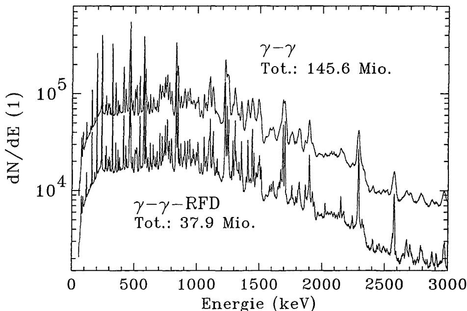
Abb. [3.33.]: Die Totalprojektionen der \gamma - \gamma - und \gamma - \gamma - \text{RFD} -Matrix
