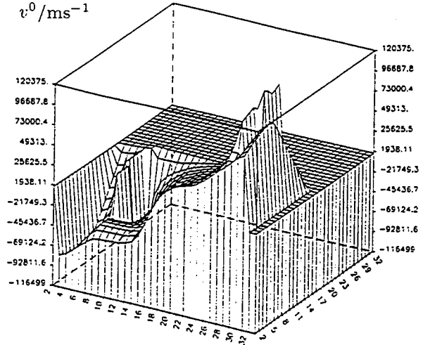
Abbildung 4.5: Dichte- und Geschwindigkeitsprofil des Hintergrundplasmas aus B2-EIRENE-Rechnung.
