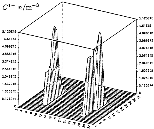
Abbildung 4.6: Dichteprofile der Kohlenstoffionen aus der Monte-Carlo-Rechnung.
