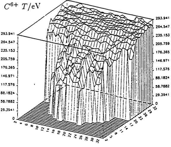
Abbildung 4.11: Temperaturprofile der Kohlenstoffionen aus der Monte-Carlo-Rechnung.
