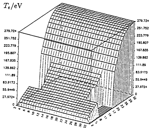
Abbildung 4.4: Elektronen- und Ionentemperatur des Hintergrundplasmas aus B2-EIRENE-Rechnung.
