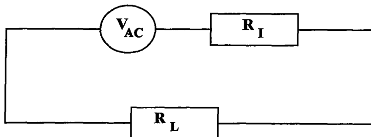
Abb. A.1: Ersatzschaltbild einer AC - Spannungsquelle mit Innenwiderstand R_I und Last R_L .
