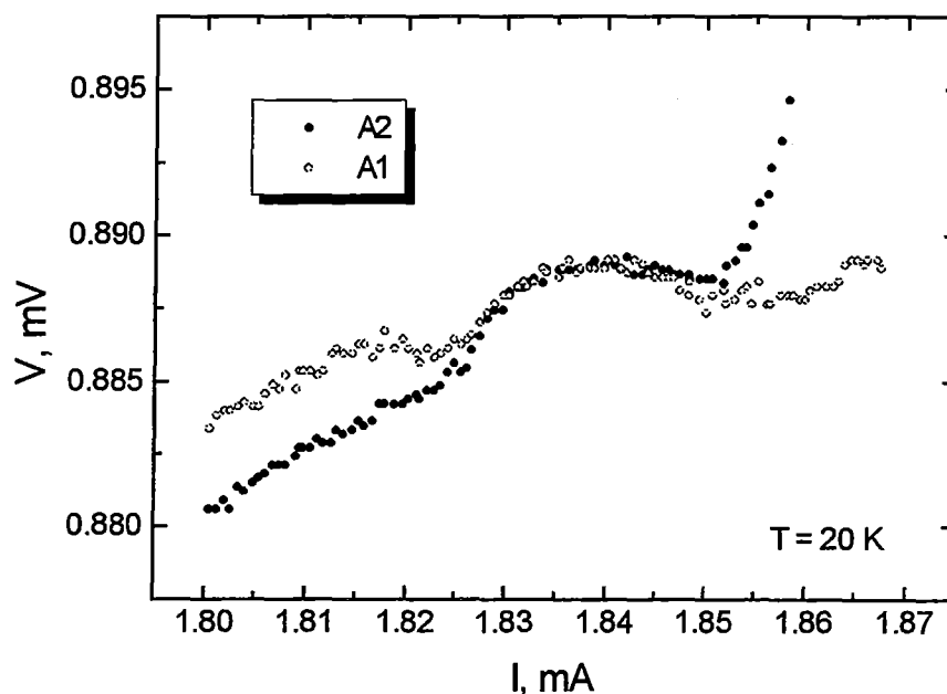
Abb. 6.11: Vergrößerter Ausschnitt des Kopplungsbereiches bei 20 K. Der induktive Einfluß der Kopplungsschleife verursacht einen nach oben gekrümmte Bogen [JAI84].
