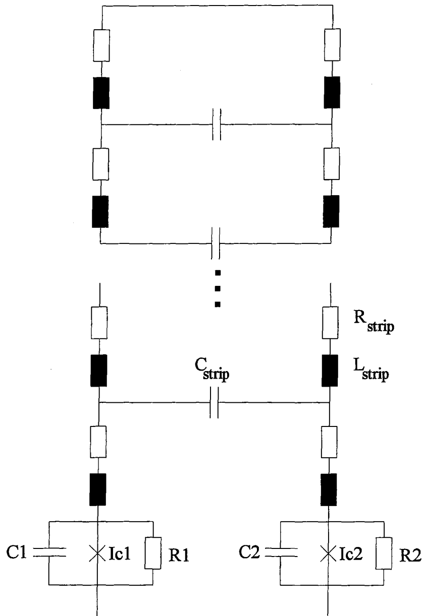
Abb. 6.2: Ersatzschaltbild einer koplanaren Streifenleitung, die an einem Ende kurzgeschlossen und an dem anderen Ende mit zwei Josephson - Kontakten abgeschlossen ist.
