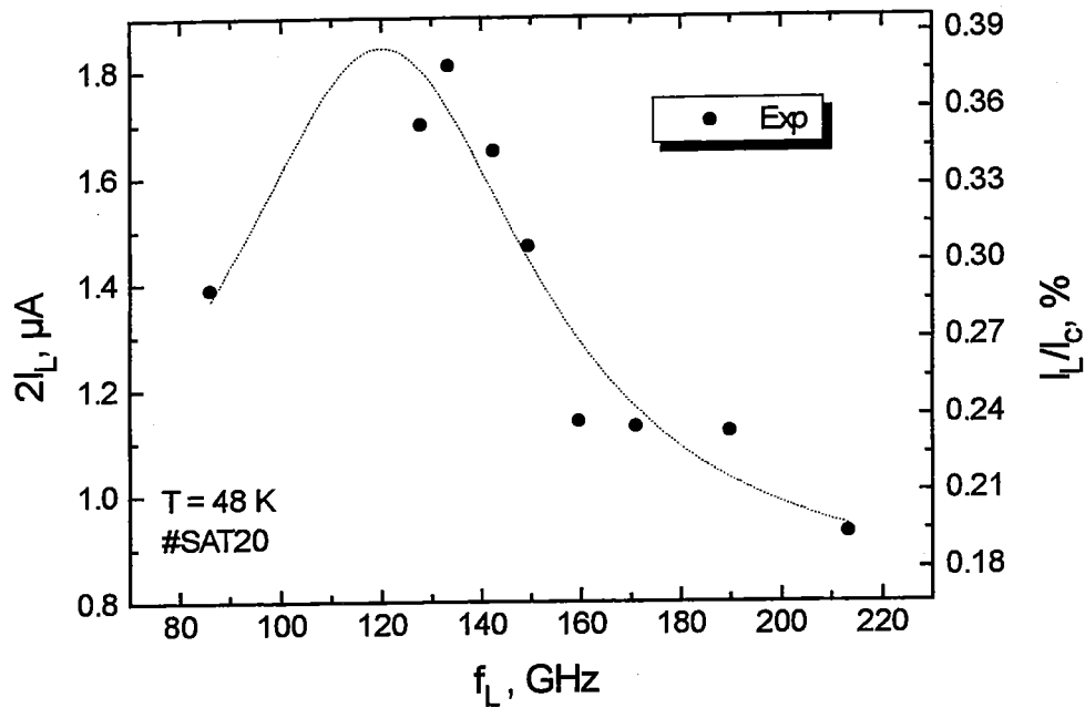
Abb. 5.14: Kopplungsstärke I_L gegen Kopplungsfrequenz f_L bei 48 K und Führungslinie, die den Verlauf approximieren soll.
