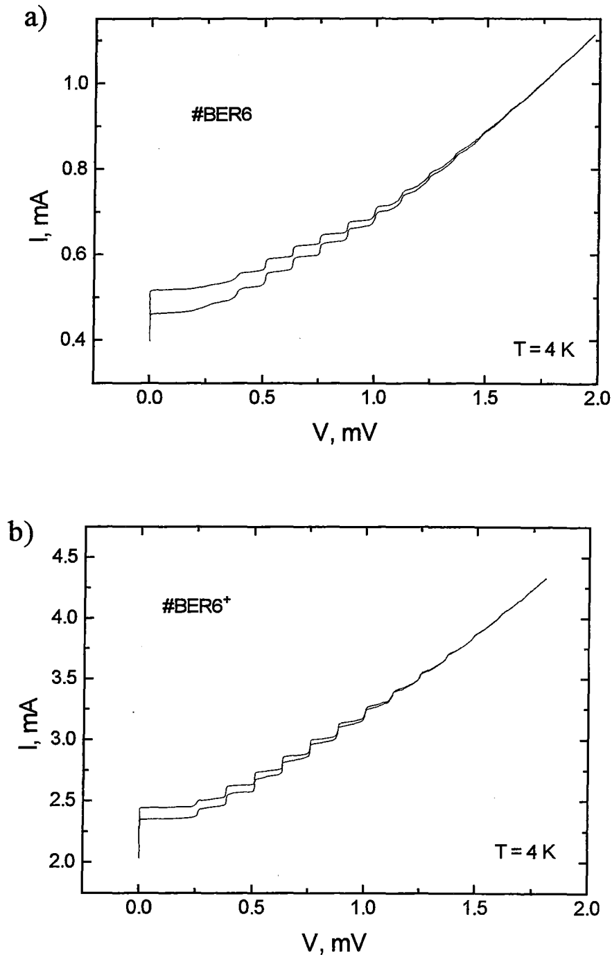
Abb. 6.3: Aufnahmen der I - V Kennlinie der Probe BER6 vor (a) und nach (b) einer 2 - stündigen Sauerstoffbeladung bei 400 °C.
