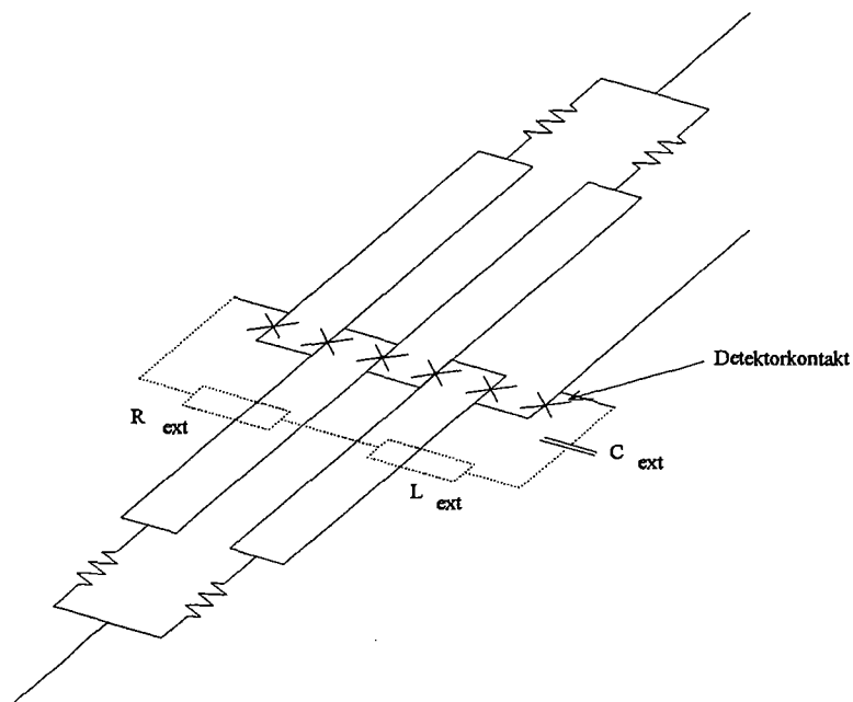
Abb. 6.17: Ersatzschaltbild eines fünf Josephson Kontaktarrays mit Detektorkontakt. Der vom Array emittierte Hochfrequenzstrom wird über eine resistive Kopplungsschleife mit einer Induktivität L_{ext} und einer Kapazität C_{ext} zum Detektorkontakt übertragen
