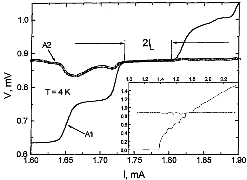
Abb. 6.9: Die I - V Kennlinie eines 4 - Kontaktarrays (A2) und eines 6 - Kontaktarrays (A1) bei T = 4 \text{ K} . A2 wird mit einer festen Spannung von 0.88 \text{ mV} gespeist, während der Strom durch A1 langsam verändert wird. Die Stufenstruktur ist deutlich sichtbar und die Definition der Kopplungsstärke I_L ist graphisch dargestellt.
