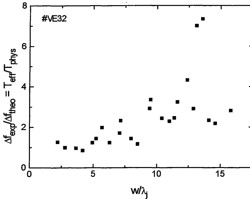
Abb. 4.3: Experimentelle Linienbreite in Einheiten der theoretischen Linienbreite aufgetragen gegen die Kontaktbreite w in Einheiten der Josephson - Eindringtiefe \lambda_J . Bis w/\lambda_J \sim 4 stimmen Theorie und Experiment über ein. Die verschiedenen Meßpunkte sind über die Temperaturabhängigkeit von \lambda_J(T) eingestellt worden
