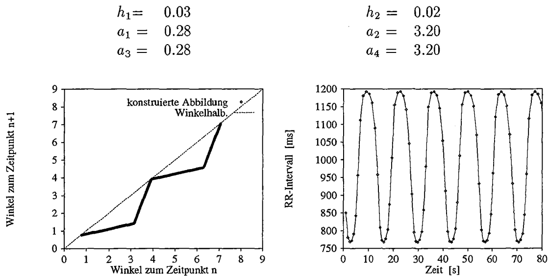
Abbildung 4.26: Kreisabbildung und daraus resultierende Zeitreihe für den Referenzfall der konstruierten, abschnittsweise linearen Abbildung
