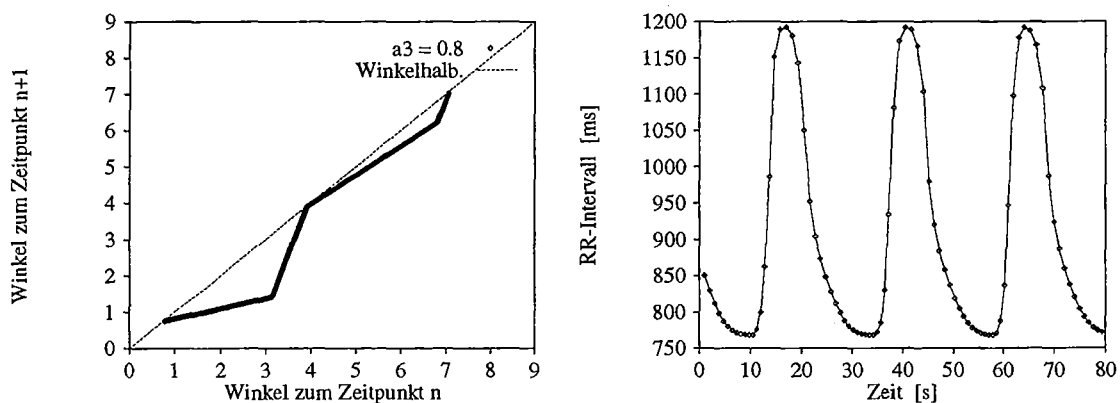
Abbildung 4.27: Abbildung und Zeitreihe, wenn ausgehend vom Referenzfall 4.26 der Parameter a_3 verkleinert wird.
