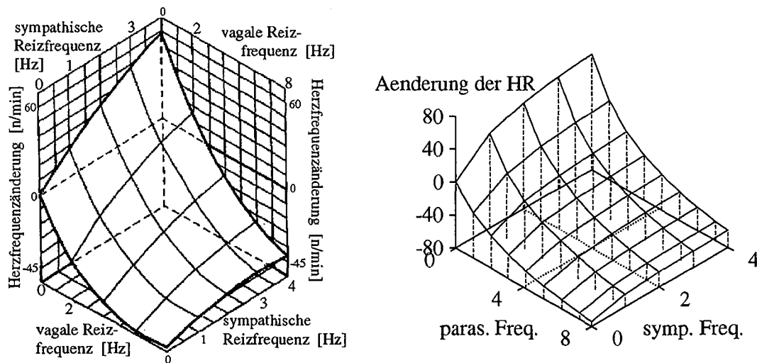
Abbildung 2.6: Darstellung der absoluten Herzfrequenzänderung bei sympathischer und parasympathischer Reizung. Links experimentelle Daten nach Levy [19], rechts simulierte Daten nach Gleichung B.7.
