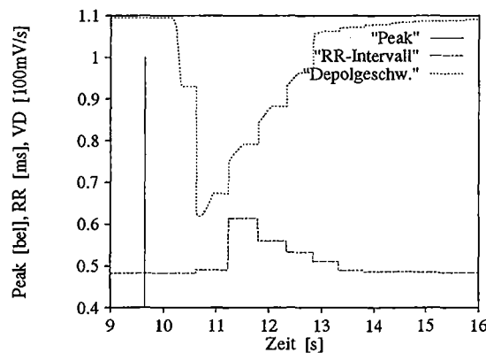
Abbildung 2.7: Simulation der Auswirkung eines \delta -förmigen Barorezeptor-Impulses (links im Bild) auf die Depolarisationsgeschwindigkeit VD (obere Kurve) und die Herzschlaglänge RR (untere Kurve). Um deutlicher zwischen Aktionspotential und langsamer Depolarisation zu unterscheiden, wurde für VD während des APs ein konstanter Wert angenommen. So entstehen die Treppen im Verlauf von VD und auch von FP in Abb. 2.8 links.
