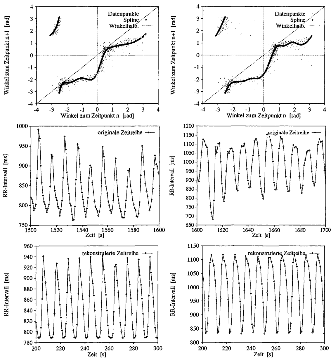
Abbildung 4.23: Vergleich von originalen und rekonstruierten Daten. Neben der Kreisabbildung (oben) sind die Zeitreihen der Herzschlaglängen dargestellt, wobei links die Daten von Proband 1 und rechts die von Proband 2 verwendet wurden.
