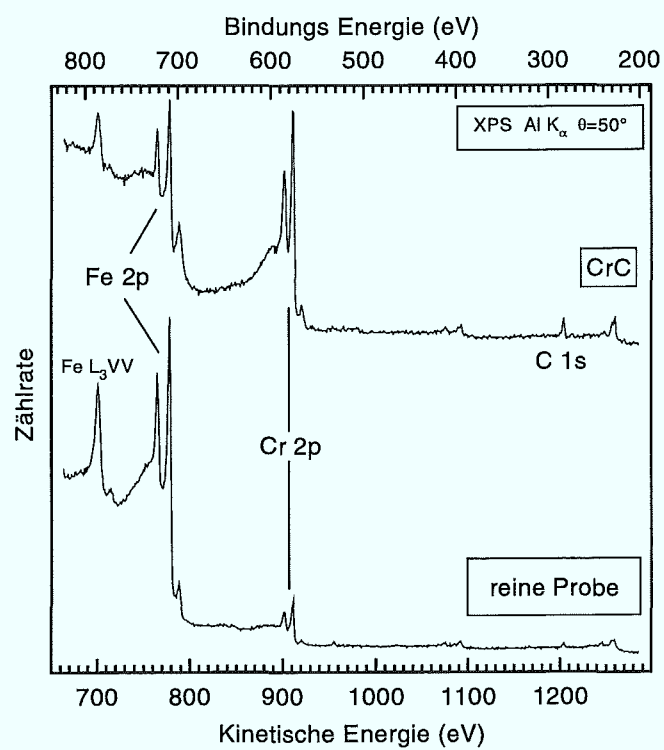
Abbildung 2.27: XP-Spektrum der reinen Fe-15%Cr(100)-Oberfläche im Vergleich mit der CrC-bedeckten Probe.
