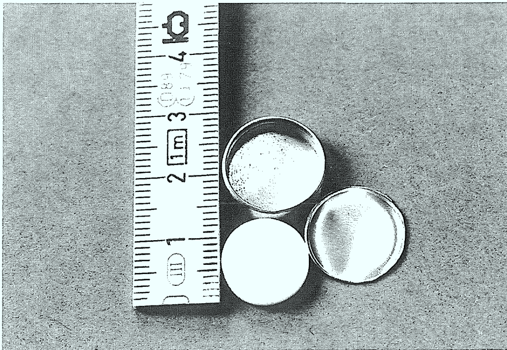
Abbildung 1: NaI-Target
