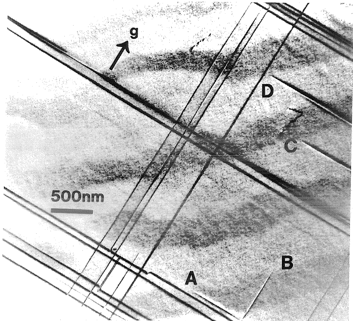
Abbildung 4.22: Hellfeldabbildung, \vec{g} = (220) , eines (18/25)-Übergitters. Die Aufsicht enthält ein System aus breiten, hellen und dunklen Streifen, die mit den Austrittsflächen von GaAs- (hell) und InGaAs-Einzelschichten (dunkel) korrespondieren. An den Orten (A), (B), (C) und (D) befinden sich Austrittspunkte von Fehlpasungsversetzungen an den Übergitterergrenzflächen, die exakt auf einer Streifengrenze enden.
