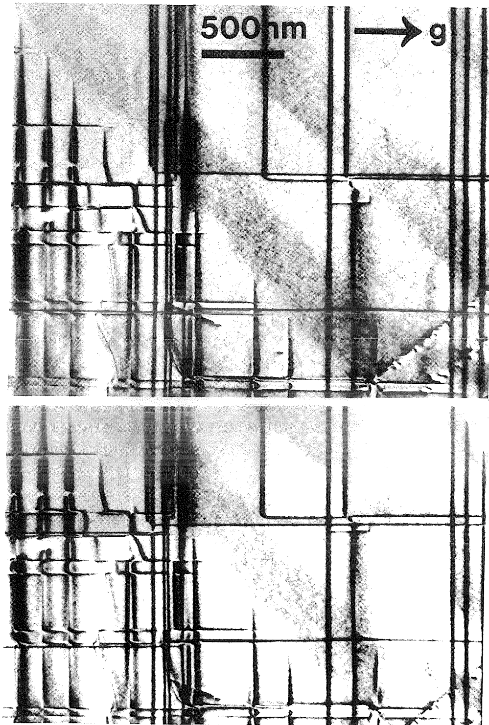
Abbildung 4.23: Stereopaar zweier Hellfeldabbildungen, \vec{g} = (220) , eines (18/25)-Übergitters. Der Projektion durch das Übergitter ist ein System aus breiten, hellen und dunklen Streifen überlagert, die mit den Austrittsflächen von GaAs- (hell) und InGaAs-Einzelschichten (dunkel) korrespondieren. Der linke untere Teil enthält zusätzlich eine Projektion der Substratgrenzfläche, an der Grenzlinie zwischen beiden Projektionen endet das dichte Substratversetzungsnetzwerk.
