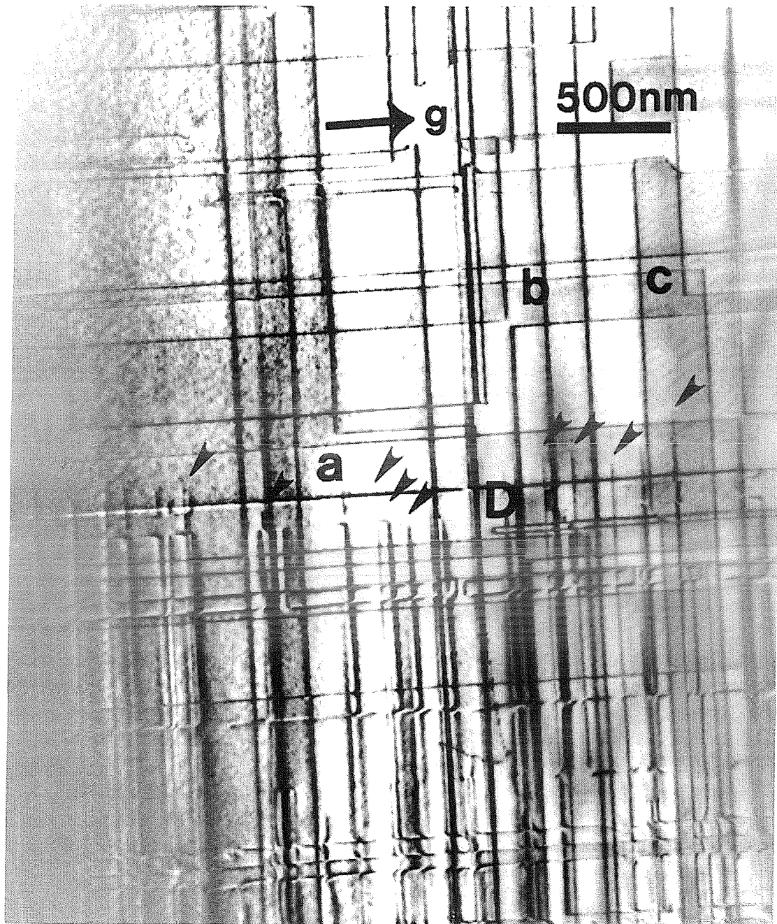
Abbildung 4.3: Schnittlinie zwischen der Substratgrenzfläche eines (18/16)-Übergitters und der Probenunterseite. In der Hellfeldabbildung, \vec{g} = (220) , sind Austrittspunkte der Versetzungslinien des Fehlpassungsnetzwerkes an der Substratgrenzfläche mit Pfeilen markiert. Bei (D) befindet sich eine Haarnadelkonfiguration zweier Fehlpassungsversetzungen, an den Stellen (a), (b) und (c) knicken Fehlpassungssegmente rechtwinklig ab.
