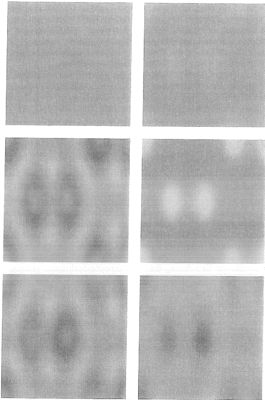
Abbildung 11.2: Simulierte Austrittswellenfunktionen von GaAs in der [110]-Projektion mit einer Ortsauflösung von 0.133 nm. Die linke Spalte zeigt die Amplitude, die rechte Spalte die Phase. Die drei verschiedenen Probendicken sind: (oben) t = 0.8 nm, (Mitte) t = 5.6 nm, (unten) t = 11.2 nm.
