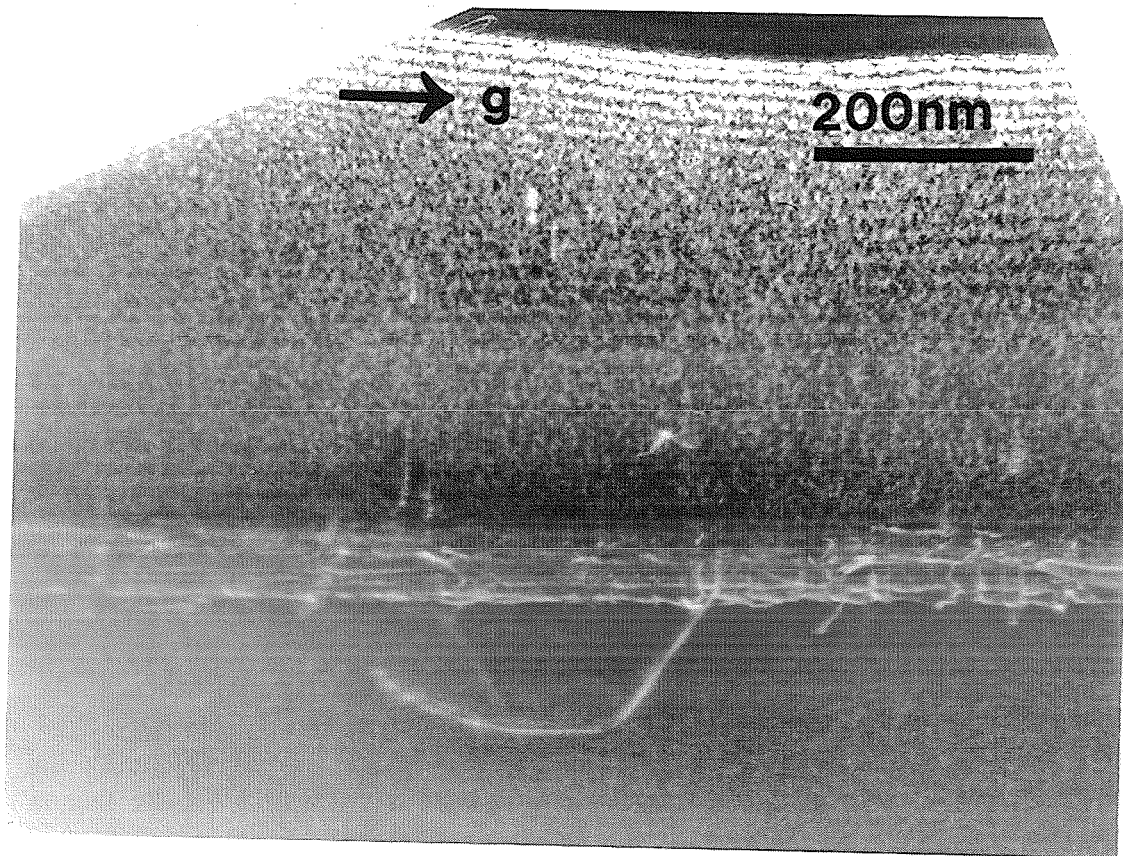
Abbildung 4.17: Weak-Beam-Dunkelfeldabbildung, \vec{g} = (220) , (\vec{g}/4\vec{g}) eines Querschnitts durch ein (18/2) -Übergitter. Unterhalb des dichten Substratversetzungsnetzwerks verläuft eine Versetzungsschleife in das Substrat hinein.
