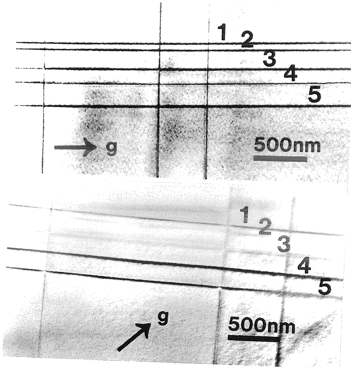
Abbildung 4.4: Auslöschung des Versetzungskontrastes von Fehlpassungssegmenten. In der Hellfeldabbildung mit dem Beugungsvektor \vec{g} = (220) sind die parallelen Fehlpassungsversetzungen (1), (2), (3), (4), (5) in Kontrast (oben). In der Hellfeldabbildung mit dem Beugungsvektor \vec{g} = (400) sind die Versetzungen (2) und (3) bis auf einen schwachen Restkontrast ausgelöscht (unten).
