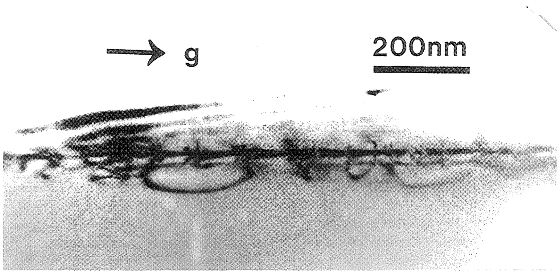
Abbildung 4.15: Hellfeldabbildung, \vec{g} = (220) , eines Querschnitts durch ein (18/6)-Übergitter. Unterhalb des dichten Substratversetzungsnetzwerks verlaufen Versetzungsschleifen in das Substrat hinein.
