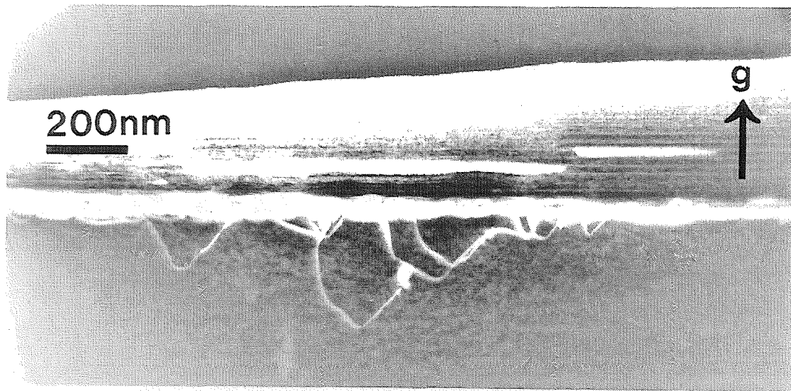
Abbildung 4.18: Weak-Beam-Dunkelfeldabbildung, \vec{g} = (004) , (\vec{g}/4\vec{g}) eines Querschnitts durch ein (18/6)-Übergitter. Unterhalb des dichten Substratversetzungsnetzwerks verläuft eine Versetzungsschleife etwa 200 nm in das Substrat hinein. Es sind außerdem zwei geradlinige Fehlpassungssegmente an den Übergittergrenzflächen in Kontrast.
