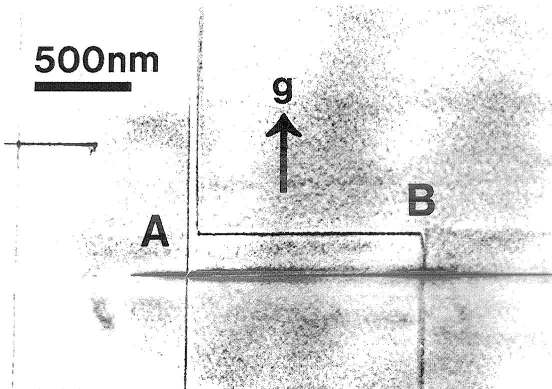
Abbildung 4.11: Hellfeldabbildung, \vec{g} = (220) , einer mehrfach abknickenden Fehlpassungsversetzung an einer Übergittergrenzfläche. Das Fehlpassungssegment wechselt die Linienrichtung bei (A) von einer auf die andere \langle 110 \rangle -Richtung, und bei (B) wieder zurück auf die ursprüngliche Richtung.
