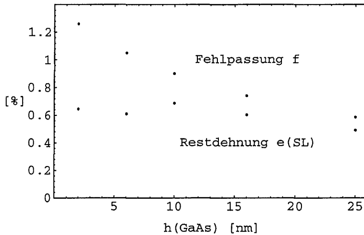
Abbildung 4.28: Abhängigkeit der homogenen Restdehnung \epsilon_{\text{SL}} der Übergitter von der GaAs-Einzelschichtdicke h_{\text{GaAs}} . Zusätzlich ist die Fehlpassung f_{\text{SL}} der entsprechenden Übergitter eingetragen.
