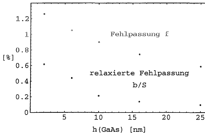
Abbildung 4.27: Abhängigkeit des relaxierten Anteils der Fehlpassung b_{eff}/S der Übergitter von der GaAs-Einzelschichtdicke h_{GaAs} . Zusätzlich ist die Fehlpassung f_{SL} der entsprechenden Übergitter eingetragen.
