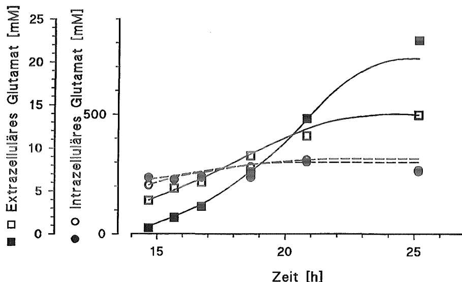
Abb. 5: L-Glutamatexport und zellinterne Glutamatkonzentrationen in der Lysinexport-defekten Mutante C. glutamicum NA8 und dem Ausgangsstamm R127. Geschlossene Symbole, C. glutamicum NA8, offene Symbole, C. glutamicum R127. ●,○ zellinternes Glutamat; ■,□ extrazelluläres Glutamat.
