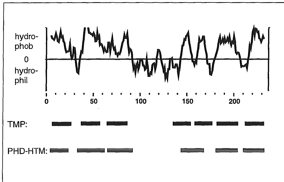
Abb. 13: Hydrophobizitätsanalyse für LysE nach Kyte & Doolittle (1982) mit einem Fenster von 13 Aminosäuren (PEPPLOT, Husar 4.0). Aufgetragen ist die durchschnittliche lokale Hydrophobizität auf der vertikalen Achse für den jeweiligen Aminosäurerest auf der horizontalen Achse. Die sechs bzw. sieben Balken geben die mögliche Lage transmembraner Helices an, deren Lage mittels der Sekundärstrukturvorhersage-Programme PHD.htm Neuronal Net (Rost et al. , 1995) bzw. TMP (Persson & Argos, 1994) ermittelt wurde.
