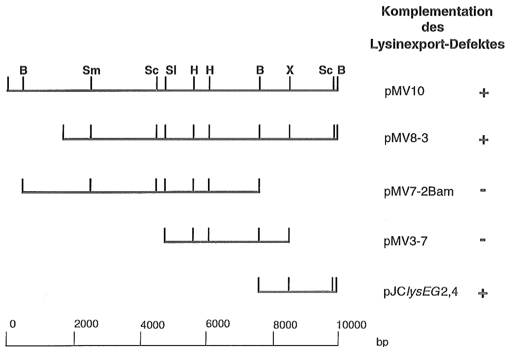
Abb. 8: Restriktionskarte der beiden Sau3A-BamHI -Fragmente der Vektoren pMV10 und pMV8-3 aus C. glutamicum R127. Beide rekombinanten Vektoren komplementieren den Lysinexport-Defekt von C. glutamicum NA8. Die Abbildung gibt zudem die Komplementation bei Subklonierung des chromosomalen DNA-Fragmentes aus dem Vektor pMV10 wieder. B = Bam HI, H = Hind III, Sc = Sac I, Sl = Sal I, Sm = Sma I, X = Xho I.
