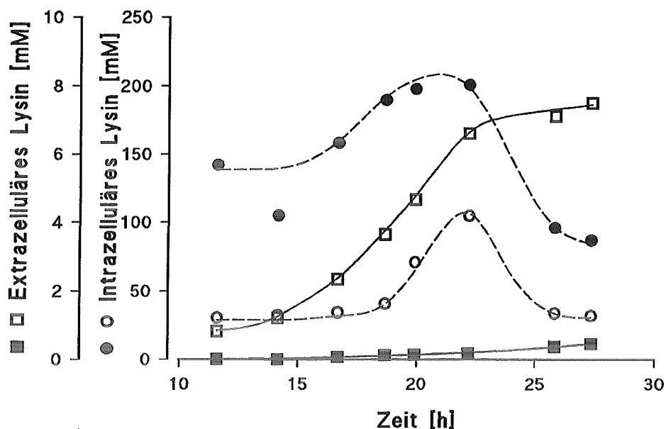
Abb. 3: Intrazelluläre und extrazelluläre Lysinkonzentrationen der Lysinexport-defekten Mutante C. glutamicum NA8 (geschlossene Symbole) und des Ausgangstammes C. glutamicum R127 (offene Symbole) nach Methioninzusatz. ●,○ intrazelluläres Lysin; ■,□ extrazelluläres Lysin.
