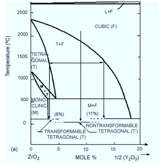
Fig. 2.11 ZrO 2 -Y 2 O 3 phase diagram [67].
