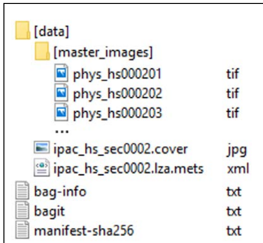
(Abb. 2: BagIt-Struktur)
