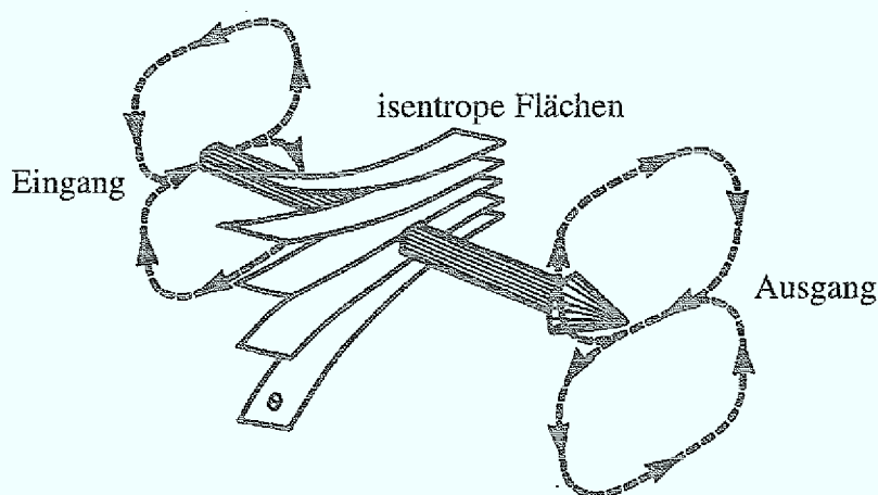
Abb. 5: Dreidimensionale Darstellung der ageostrophischen Zirkulationen (gestrichelte Linien) quer zur horizontalen Strömung in einem Jet Streak (runder Pfeil) für den Jeteingang und den -ausgang (Mattocks and Bleck, 1986). Die isentropischen Flächen liegen auf der antizyklonalen Jetseite vertikal weiter auseinander als auf der zyklonalen Jetseite.
