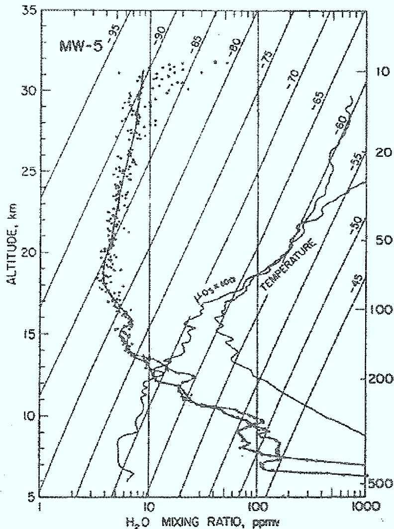
Abb. 14: Vertikalprofil der spezifischen Feuchte über Laramie, WY, am 08. September 1978. Punkte und Kreuze unterscheiden die Wasseradmpf-Profile des Aufstiegs beziehungsweise des Abstiegs. Die durchgezogenen Linien geben die Ozonkonzentration und die Temperatur wieder (Kley et al., 1979).
