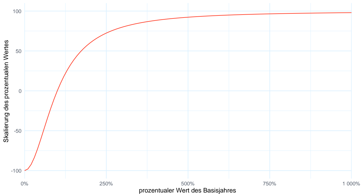
Abbildung 11: Vergleich prozentuale Veränderung mit skaliertes Veränderungsrate \ln(1 + p)
