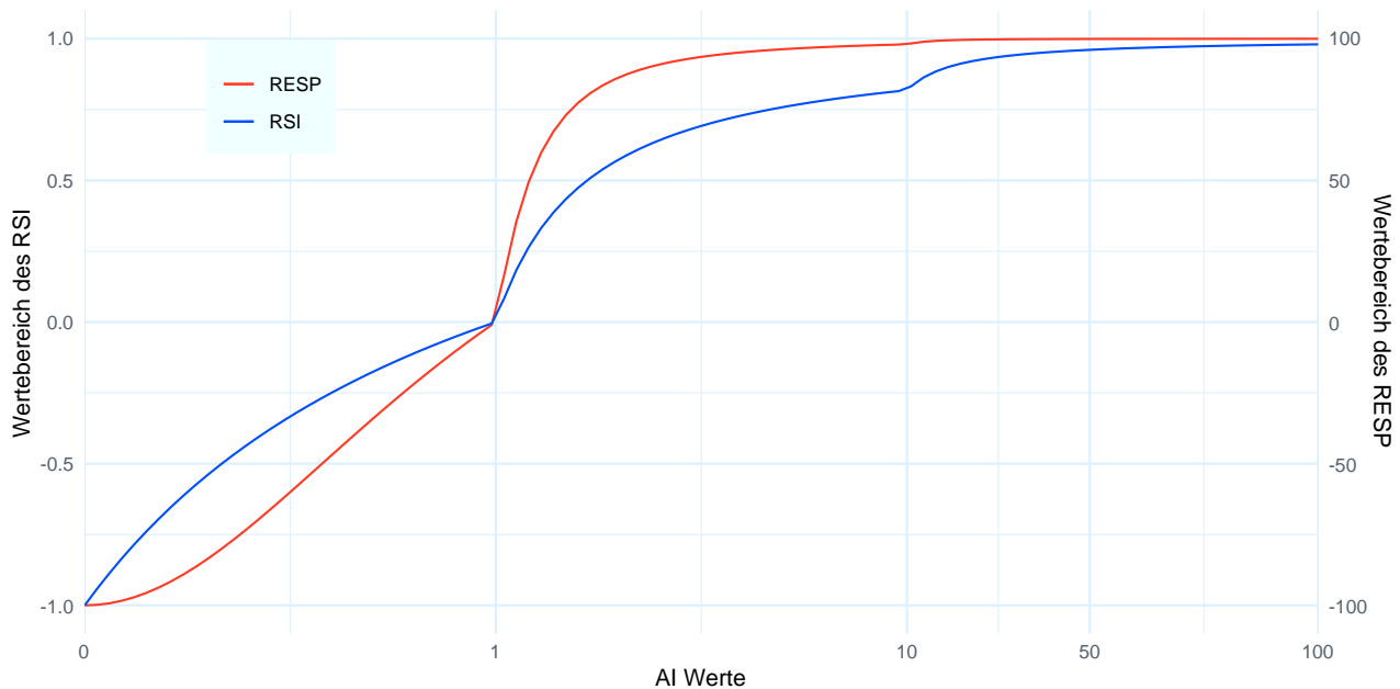
Abbildung 1: Vergleich RSI und RESP auf dem Intervall [-1, 1]
