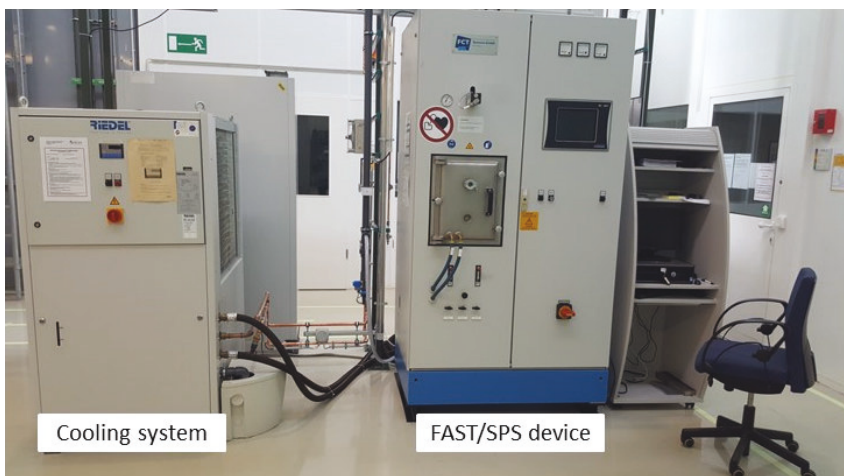
Figure 3-4 : FAST/SPS FCT-HP D 5/2, FCT system GmbH at IEK-1, Forschungszentrum Jülich GmbH
