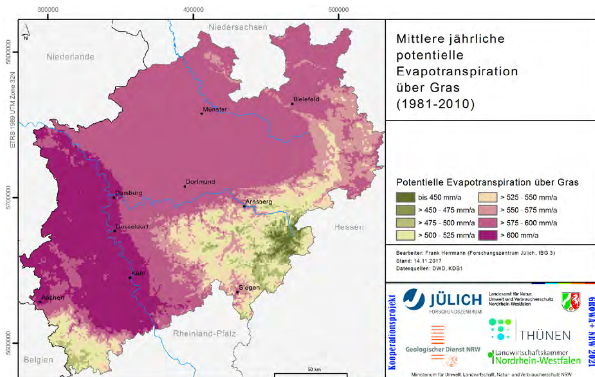
Abb. 8: Mittlere jährliche potentielle Evapotranspiration über Gras (1981-2010)
