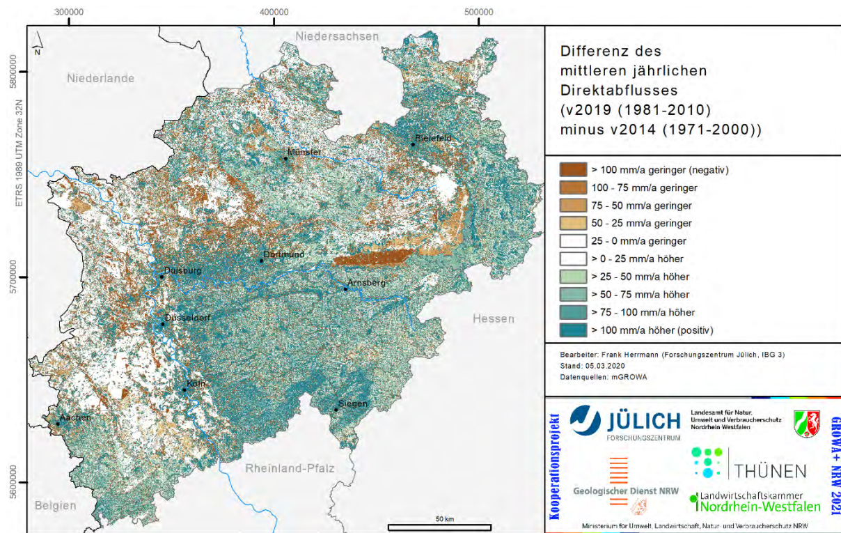
Abb. 53: Differenz des mittleren jährlichen Direktabflusses aus den Versionen v2019 (Periode 1981-2010, zusammengesetzt aus KDB1 und KDB2) und v2014 (Periode 1971-2000)
