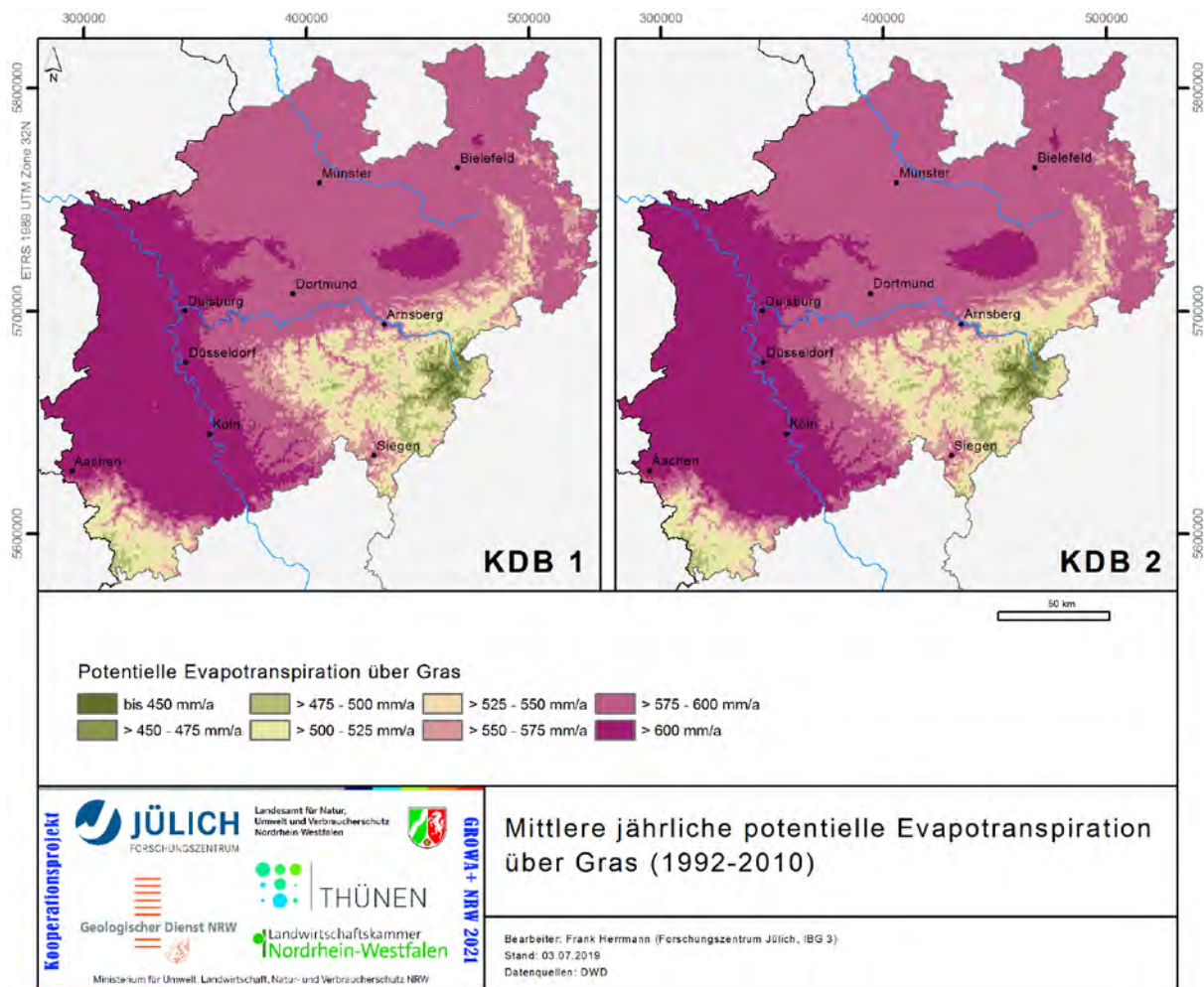
Abb. 9: Mittlere jährliche potentielle Evapotranspiration über Gras (1992-2010) in KDB1 (links) und KDB2 (rechts, mit Korrektur)
