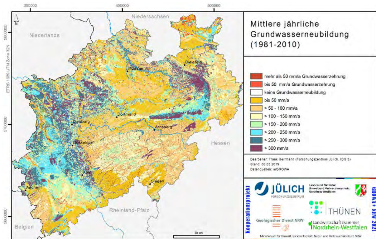
Abb. 43: Mittlere jährliche Grundwasserneubildung (1981-2010)
