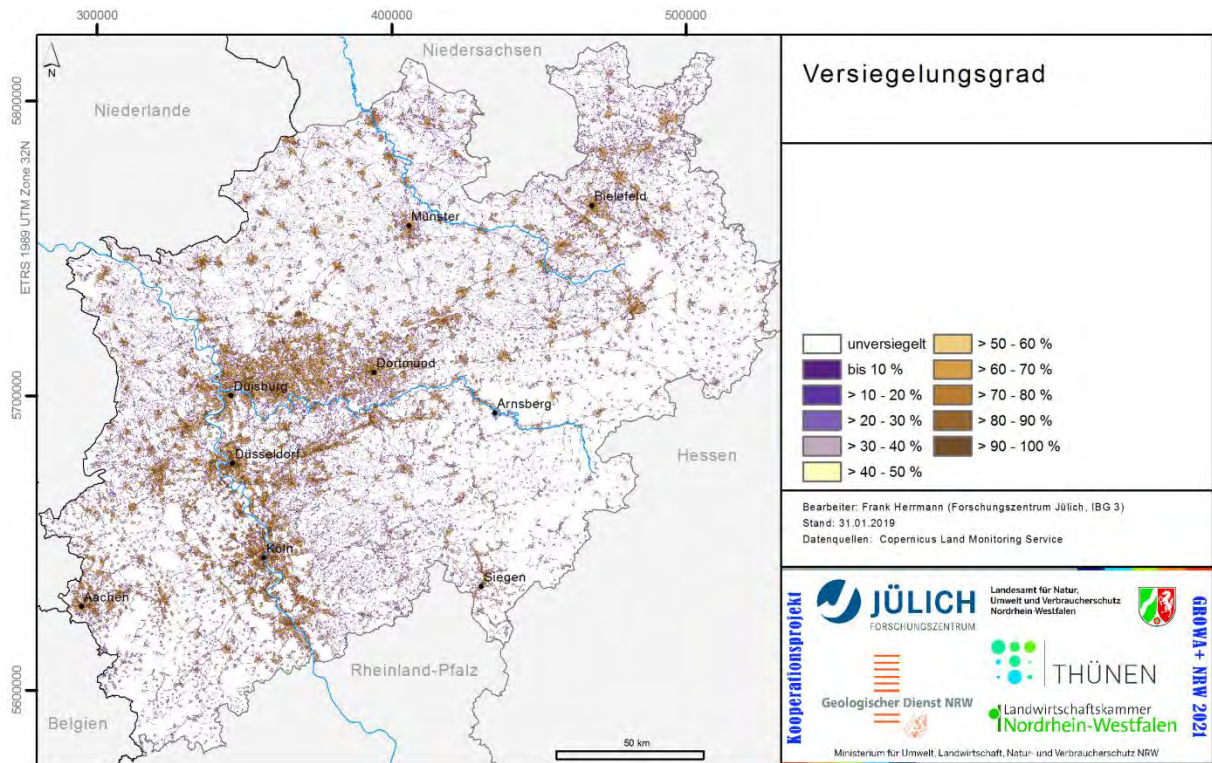
Abb. 11: Versiegelungsgrad der Erdoberfläche. Datenquelle: Copernicus Land Monitoring Service, High Resolution Layer Imperviousness (2012) 20 m
