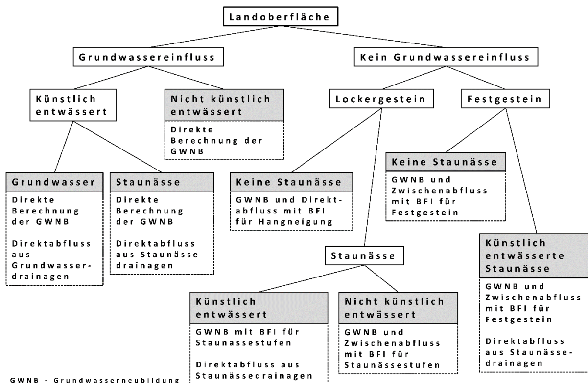
Abb. 3: Entscheidungsbaum in der mGROWA-Abflusseparation zur Bestimmung der für die Berechnung der Grundwasserneubildung und einzelner Direktabflusskomponenten relevanten Standorteigenschaften.
