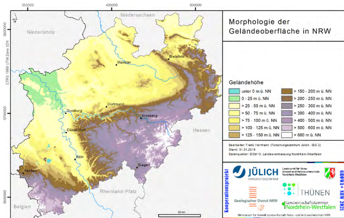
Abb. 13: Morphologie der Geländeoberfläche in Nordrhein-Westfalen Datenquelle: DGM10, Landesvermessung Nordrhein-Westfalen
