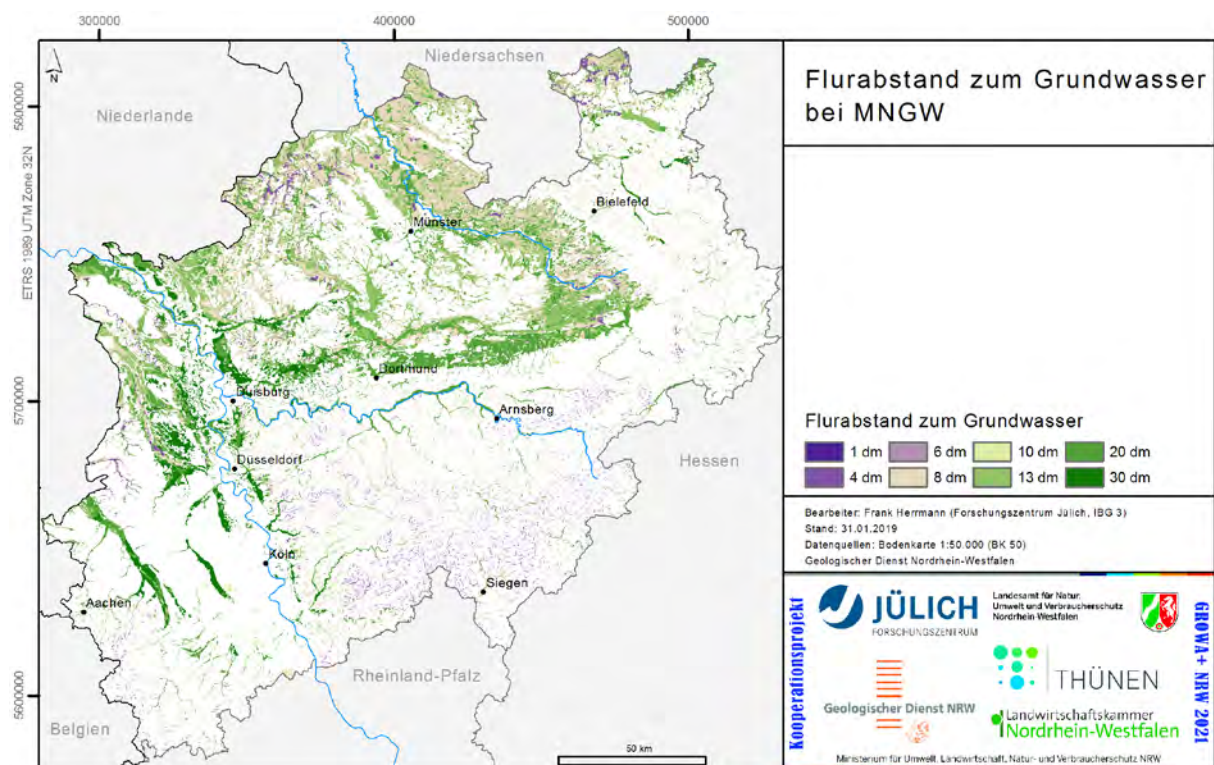
Abb. 23: Flurabstand des Grundwassers bei MNGW aus BK 50
