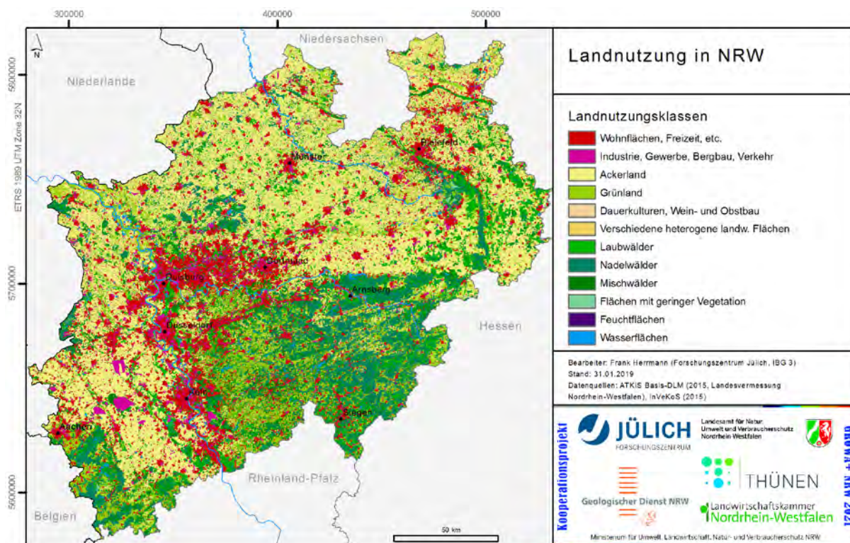
Abb. 10: Landnutzung in NRW, dargestellt sind Landnutzungsklassen
