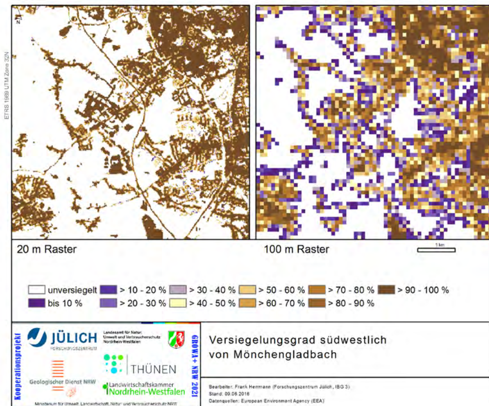
Abb. 12: Versiegelungsgrad südwestlich von Mönchengladbach vor (links) und nach (rechts) der Übertragung auf das 100 m Modellraster
