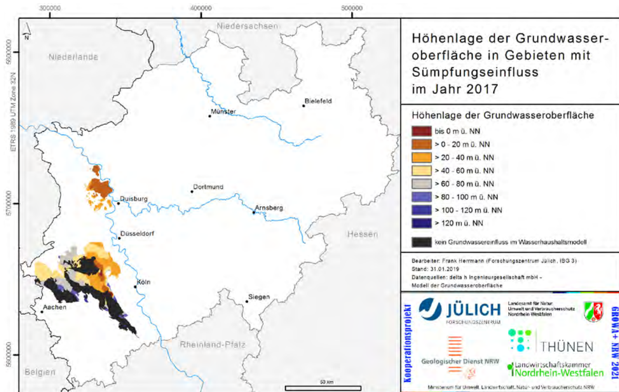
Abb. 25: Höhenlage der Grundwasseroberfläche in Gebieten mit Sumpfungseinfluss im Jahr 2017
