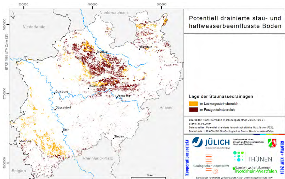
Abb. 19: Potentiell drainierte stau- und haftwasserbeeinflusste Böden
