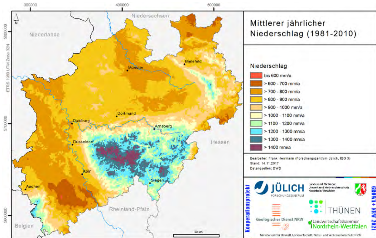
Abb. 7: Mittlerer jährlicher Niederschlag (1981-2010)
