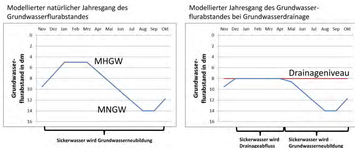
Abb. 4: Exemplarisch modellierter natürlicher Jahresgang des Grundwasserflurabstandes und dessen veränderter Jahresgang bei vorhandenen Grundwasserdrainagen
