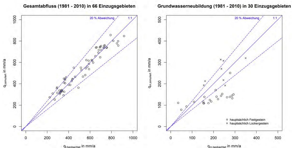
Abb. 49: Evaluierung des mit mGROWA ermittelten mittleren jährlichen Gesamtabflusses und der mittleren jährlichen Grundwasserneubildung in der Periode 1981-2010
