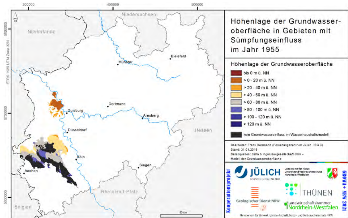
Abb. 26: Höhenlage der Grundwasseroberfläche in Gebieten mit Sumpfungseinfluss im Jahr 1955
