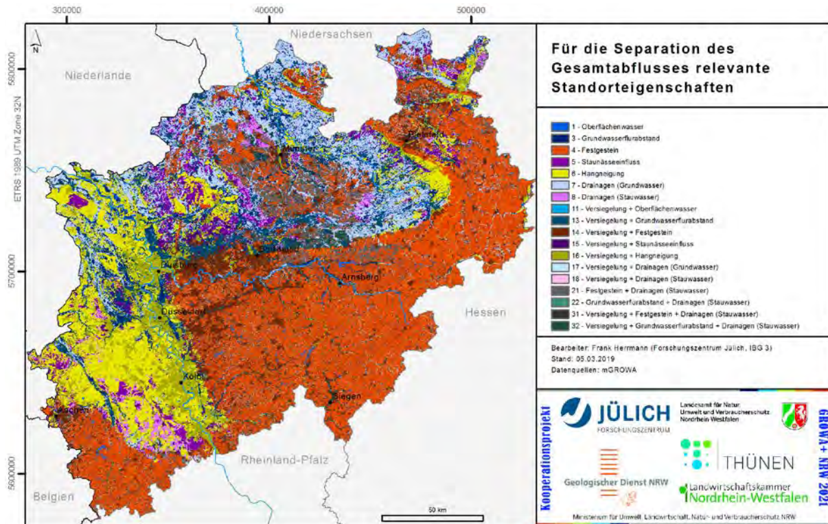
Abb. 5: Für die Separation des Gesamtabflusses relevante Standorteigenschaften
