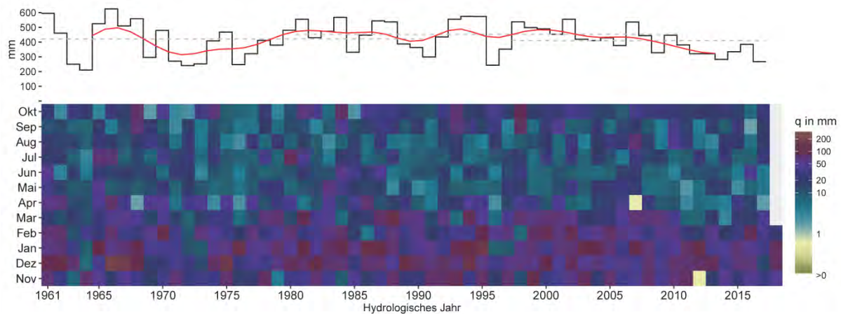
Abb. 33: Zeitreihendarstellung der Abflussbildung in NRW. Erläuterung der Darstellungsweise im Text am Kapitelanfang
