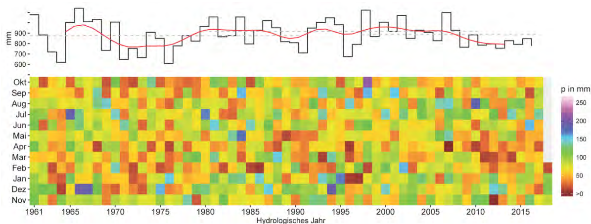
Abb. 29: Zeitreihendarstellung des Niederschlags in NRW. Erläuterung der Darstellungsweise im Text am Kapitelanfang
