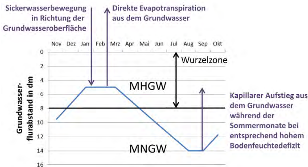
Abb. 2: Schematische Darstellung des Jahresganges des Grundwassers als Randbedingung sowie der in diesem Zusammenhang mit mGROWA simulierten Prozesse. MHGW – mittlerer Hochstand des Grundwassers; MNGW – mittlerer Niedrigstand des Grundwassers.
