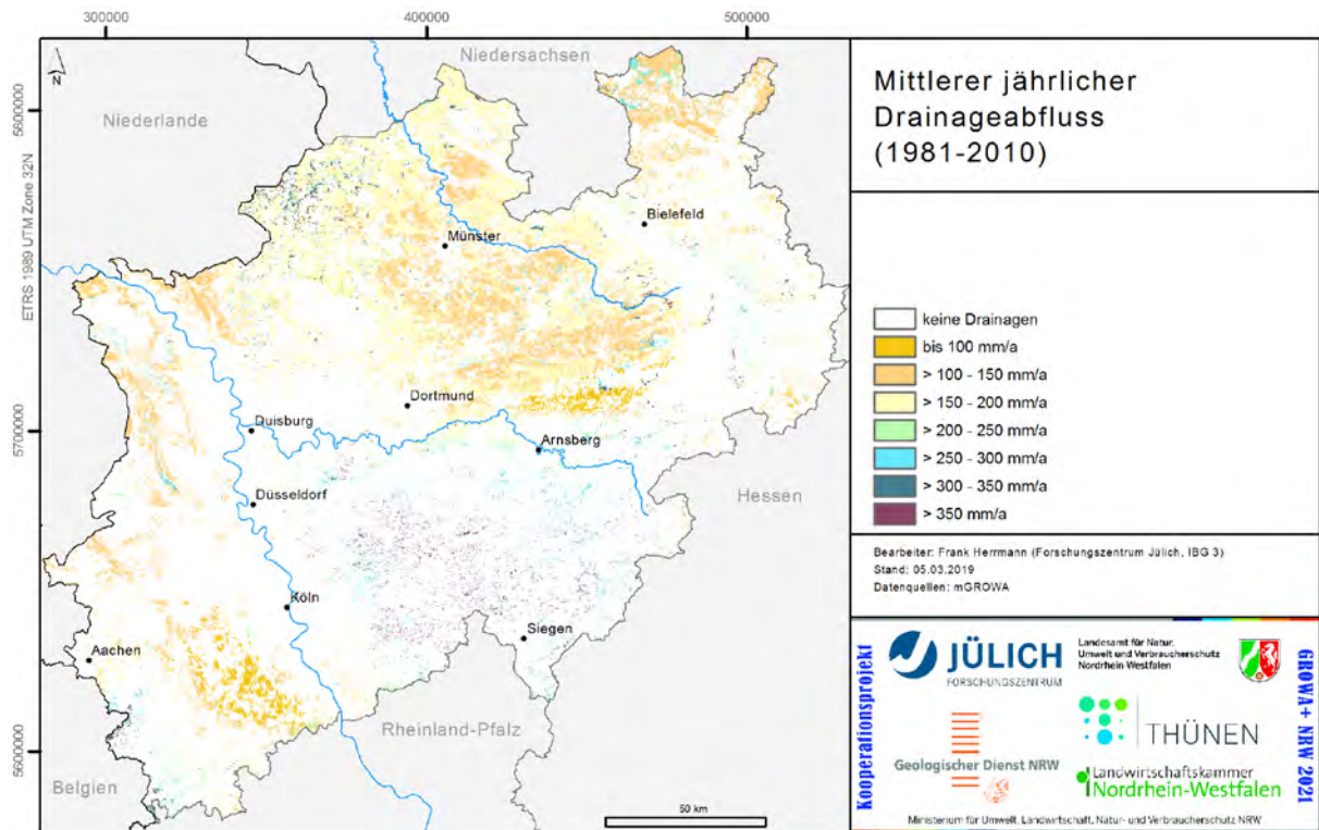
Abb. 40: Mittlerer jährlicher Drainageabfluss (1981-2010)
