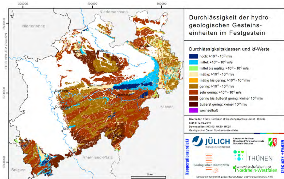
Abb. 20: Durchlässigkeit der hydrogeologischen Gesteinseinheiten im Festgestein
