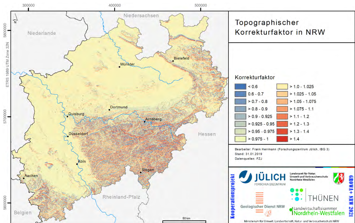
Abb. 16: Topographischer Korrekturfaktor in Nordrhein-Westfalen
