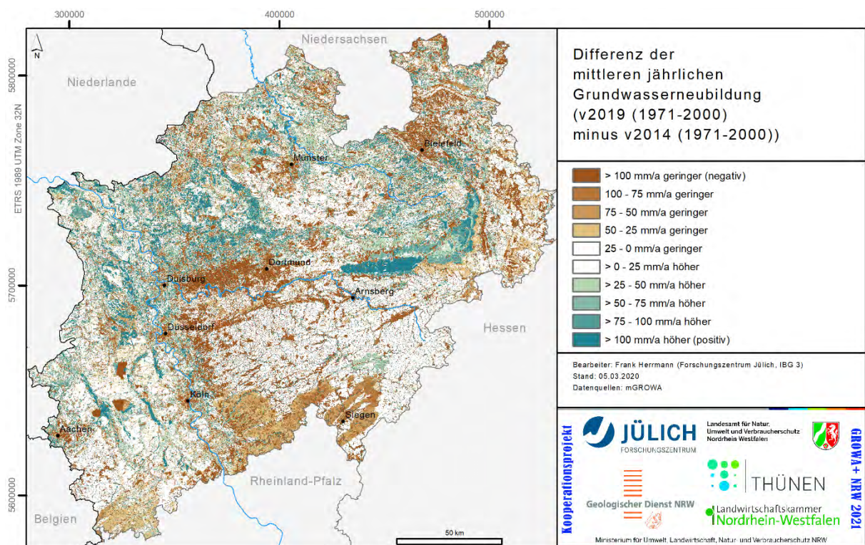
Abb. 52: Differenz der mittleren jährlichen Grundwasserneubildung aus den Versionen v2019 (Periode 1971-2000, KDB1) und v2014 (Periode 1971-2000)
