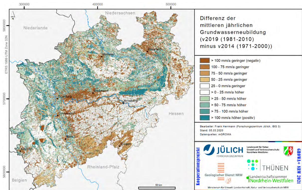
Abb. 51: Differenz der mittleren jährlichen Grundwasserneubildung aus den Versionen v2019 (Periode 1981-2010, zusammengesetzt aus KDB1 und KDB2) und v2014 (Periode 1971-2000)
