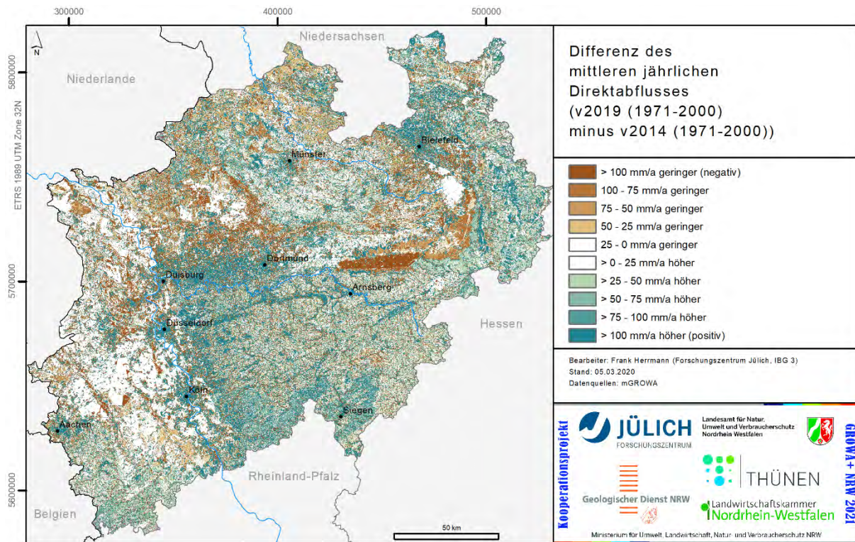
Abb. 54: Differenz des mittleren jährlichen Direktabflusses aus den Versionen v2019 (Periode 1971-2000, KDB1) und v2014 (Periode 1971-2000)
