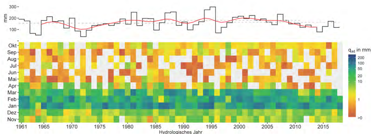
Abb. 35: Zeitreihendarstellung des Abflusses aus Grundwasserdrainagen in NRW. Erläuterung der Darstellungsweise im Text am Kapitelfanfang
