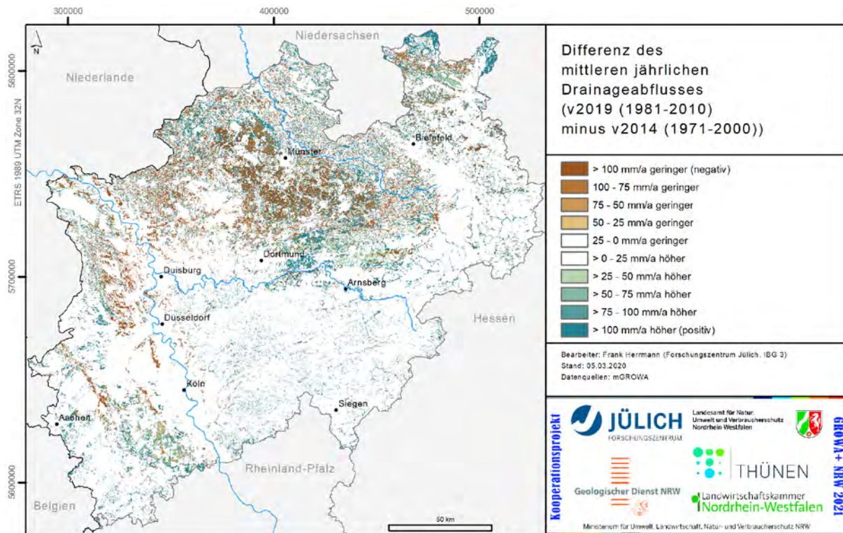
Abb. 55: Differenz des mittleren jährlichen Drainageabflusses aus den Versionen v2019 (Periode 1981-2010, zusammengesetzt aus KDB1 und KDB2) und v2014 (Periode 1971-2000)
