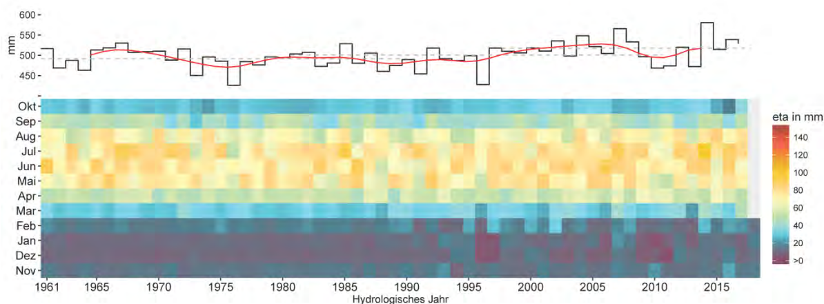
Abb. 30: Zeitreihendarstellung der tatsächlichen Evapotranspiration in NRW. Erläuterung der Darstellungsweise im Text am Kapitelanfang
