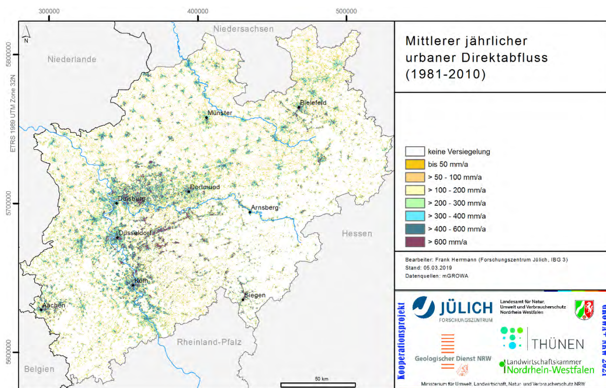
Abb. 37: Mittlerer jährlicher urbaner Direktabfluss (1981-2010)
