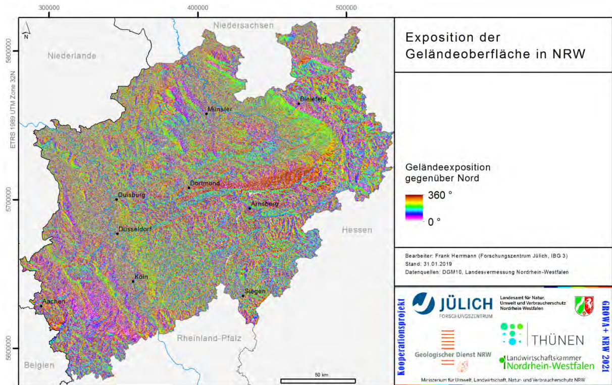
Abb. 15: Exposition der Geländeoberfläche gegenüber Nord in Nordrhein-Westfalen
