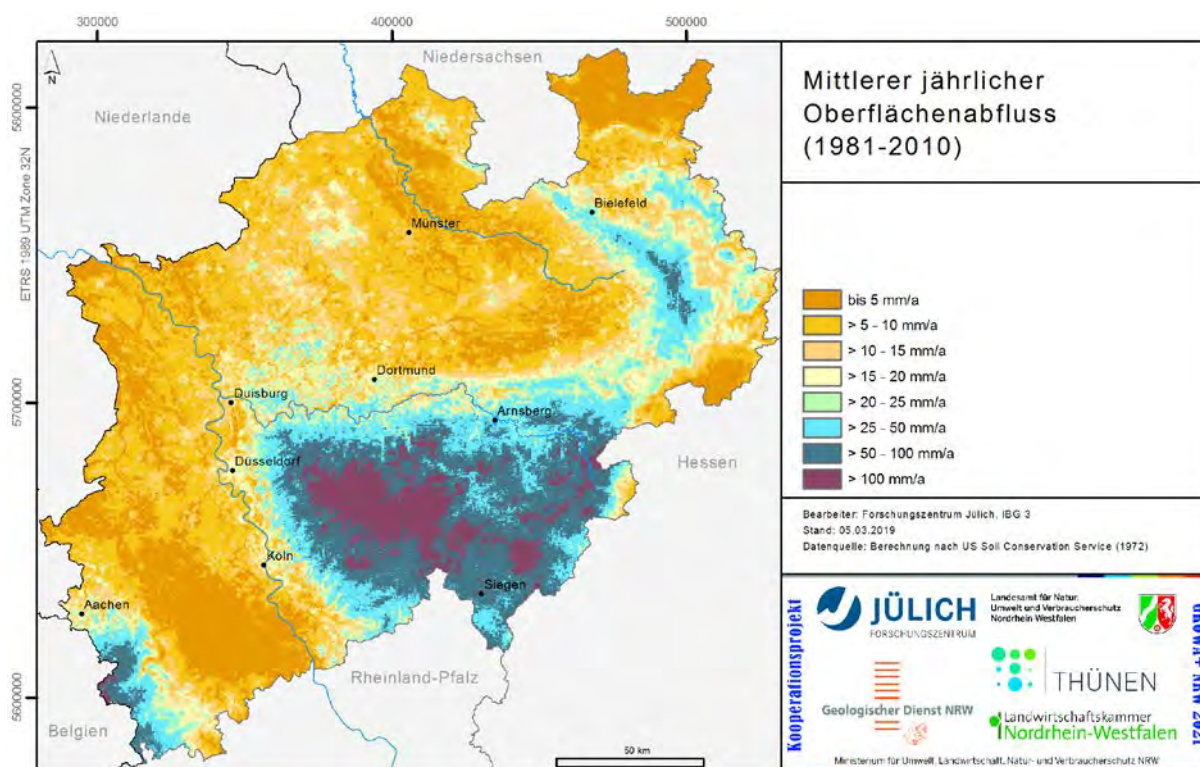
Abb. 44: Mittlerer jährlicher Oberflächenabfluss (1981-2010) berechnet nach US Soil Conservation Service (1972)
