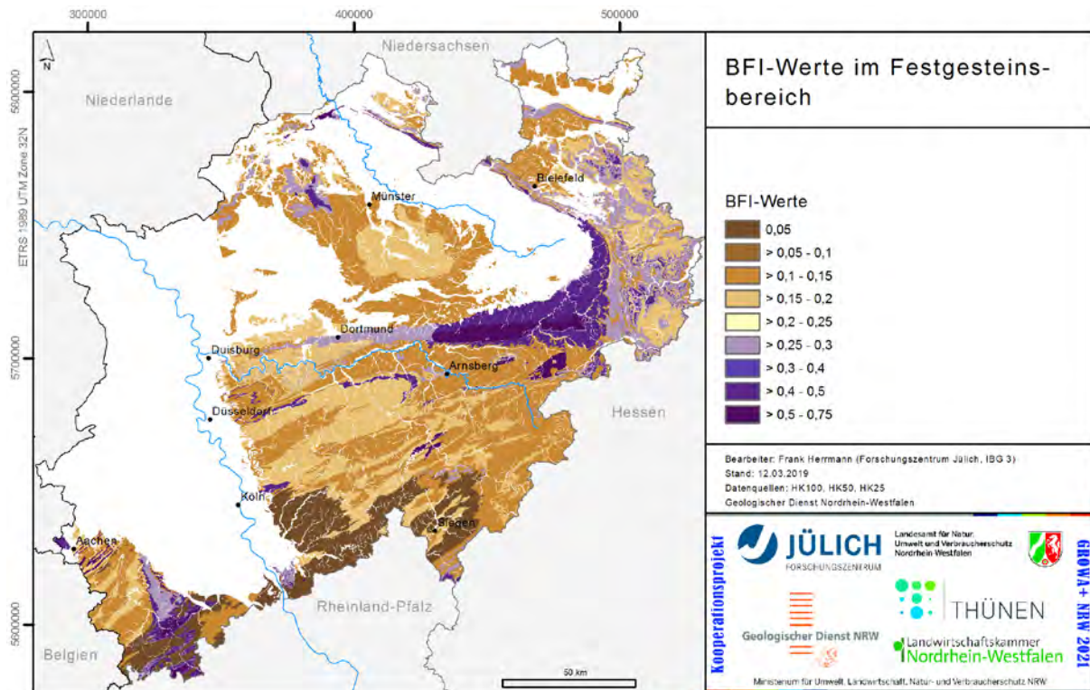
Abb. 21: BFI-Werte im Festgesteinsbereich
