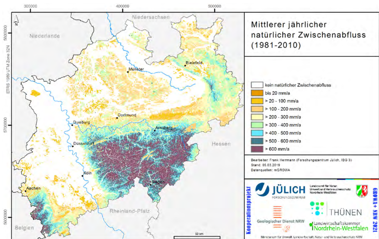
Abb. 41: Mittlerer jährlicher natürlicher Zwischenabfluss (1981-2010)
