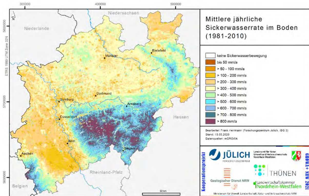
Abb. 38: Mittlere jährliche Sickerwasserrate im durchwurzelter Boden (1981-2010)
