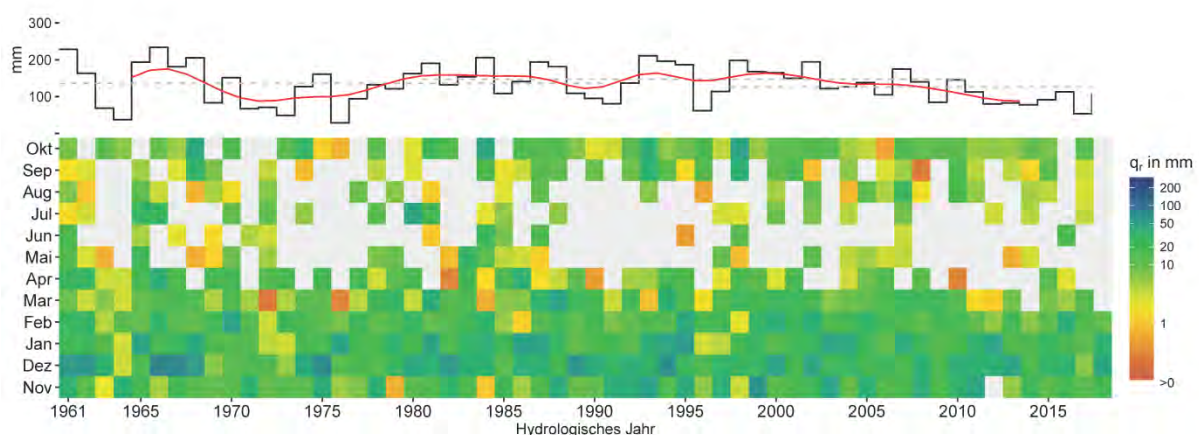
Abb. 34: Zeitreihendarstellung der Netto-Grundwasserneubildung in NRW. Erläuterung der Darstellungsweise im Text am Kapitelanfang
