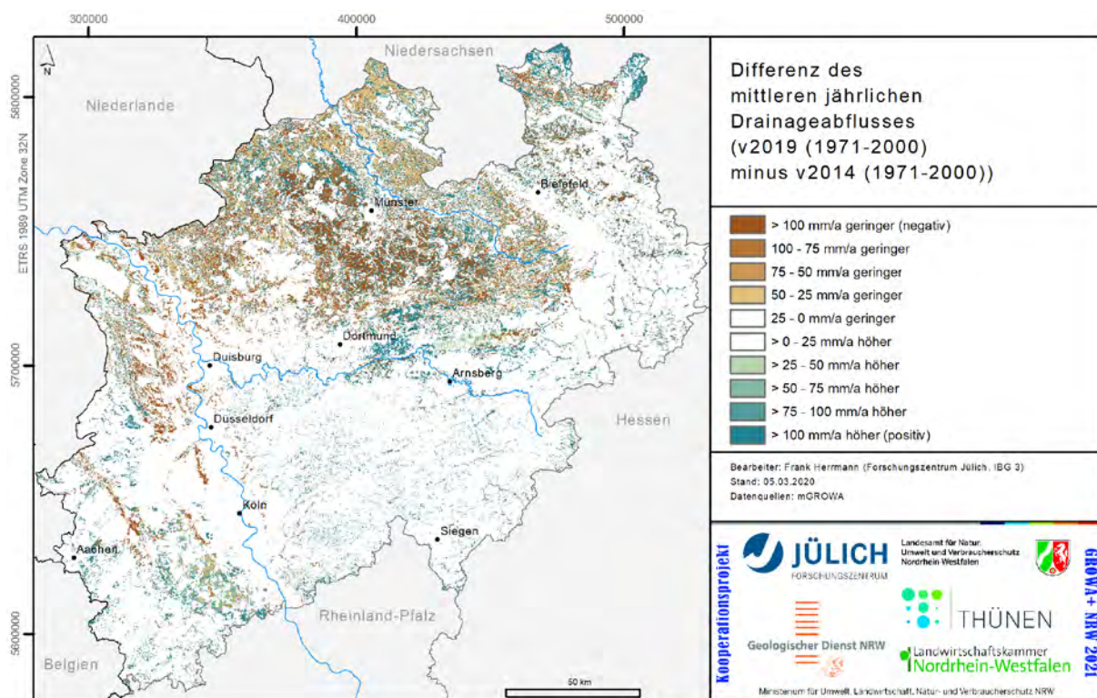
Abb. 56: Differenz des mittleren jährlichen Drainageabflusses aus den Versionen v2019 (Periode 1971-2000, KDB1) und v2014 (Periode 1971-2000)
