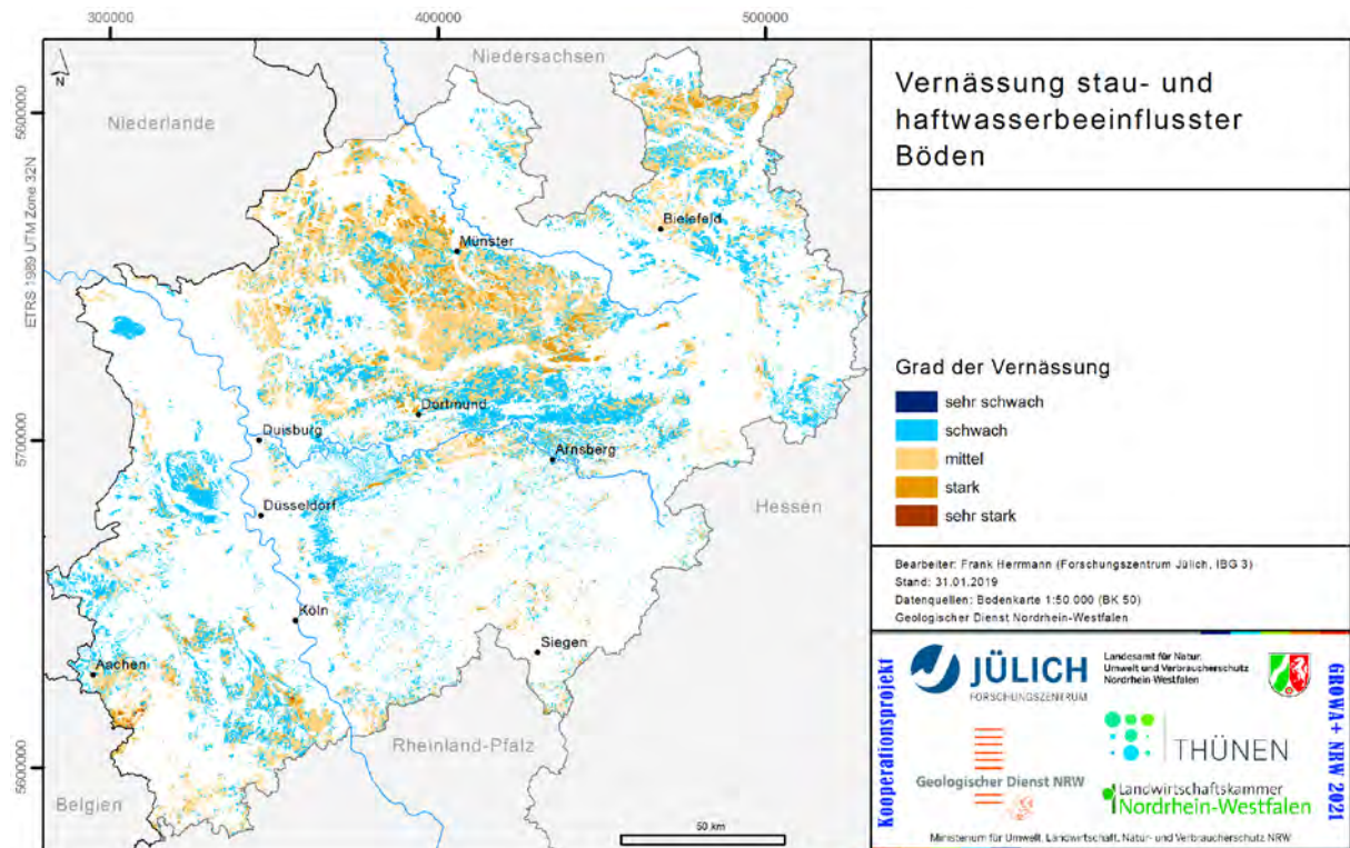
Abb. 18: Vernässung stau- und haftwasserbeeinflusster Böden
