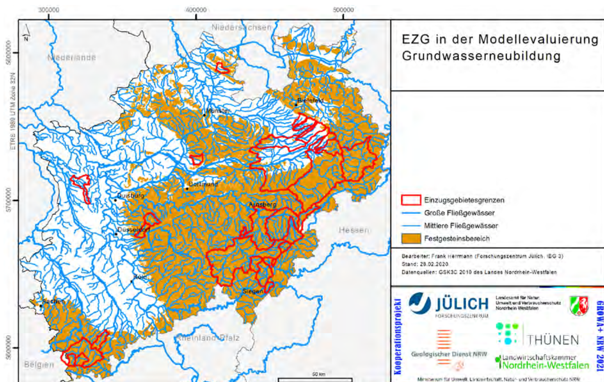
Abb. 48: Im Rahmen der Evaluierung der Grundwasserneubildung ausgewählte Einzugsgebiete
