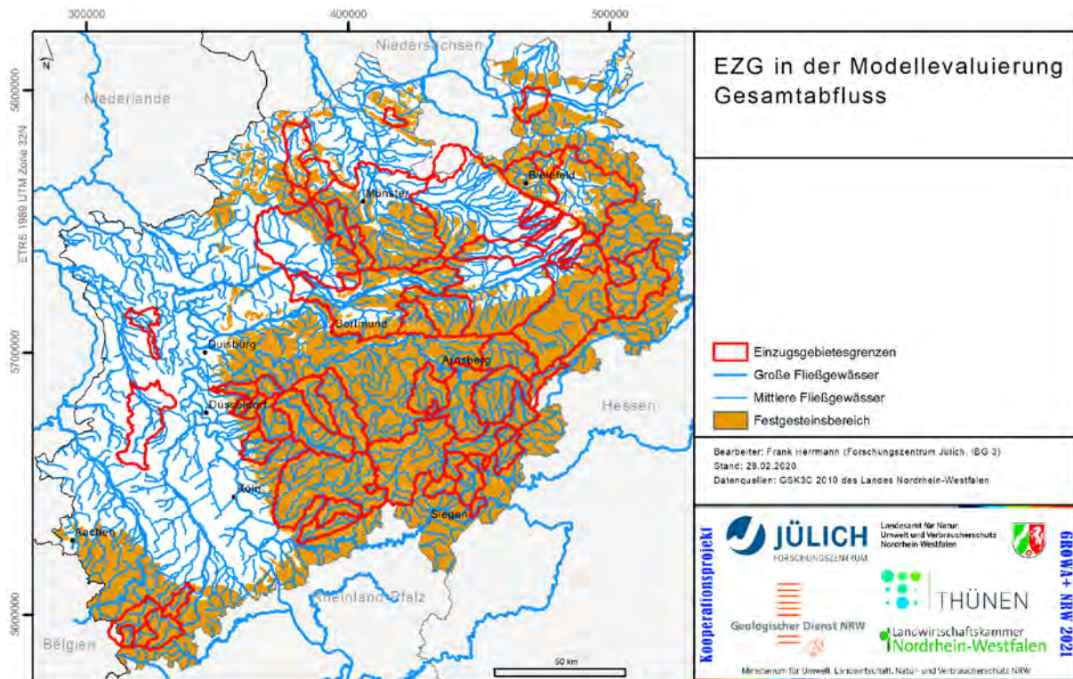
Abb. 47: Im Rahmen der Evaluierung des Gesamtabflusses ausgewählte Einzugsgebiete
