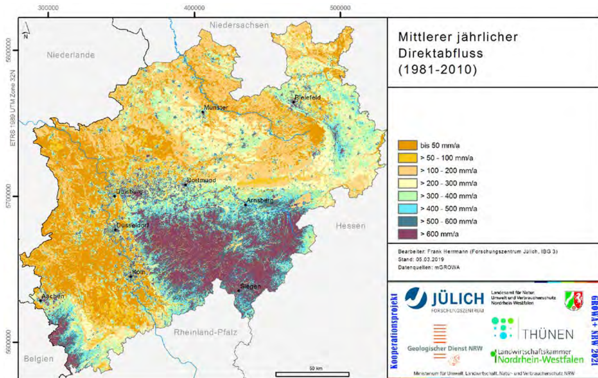
Abb. 42: Mittlerer jährlicher Direktabfluss (1981-2010)
