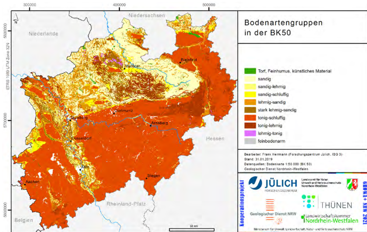
Abb. 17: Bodenartengruppen in der BK50. Weiße Flächen stellen einerseits Wasserflächen dar, aber auch Flächen, für die Ersatzprofile verwendet wurden
