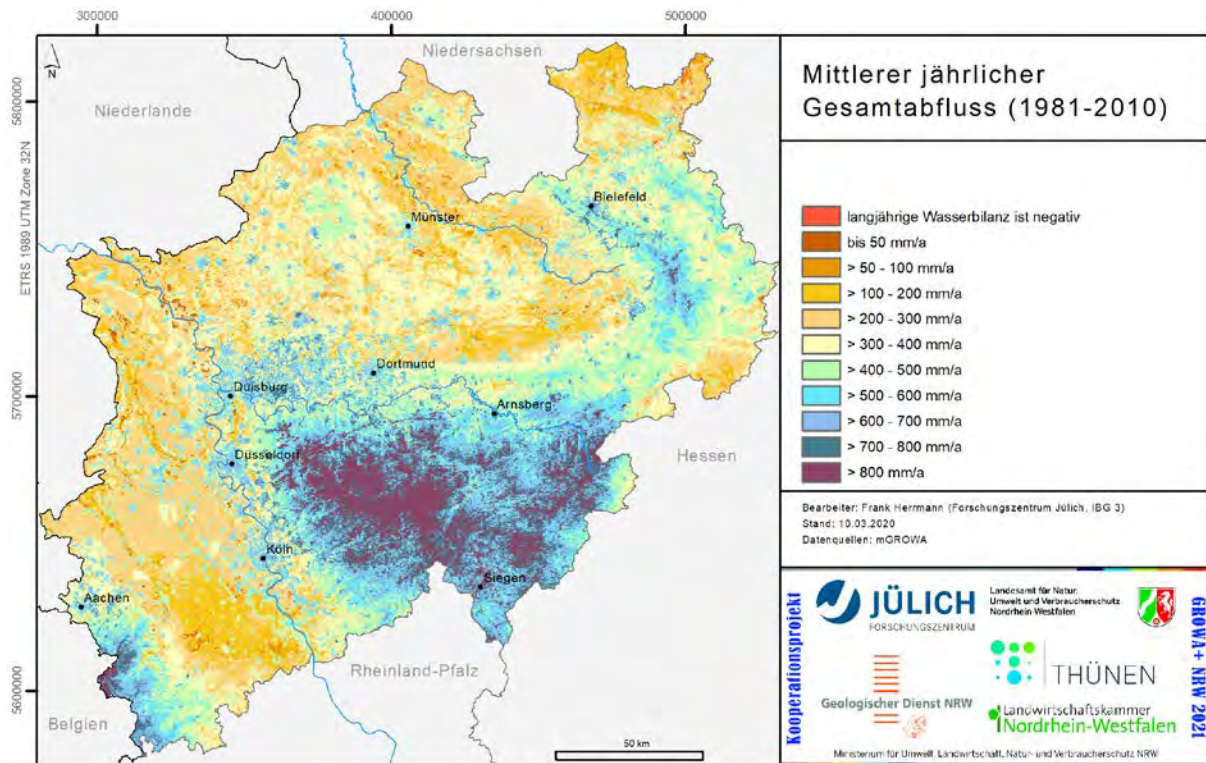
Abb. 39: Mittlerer jährlicher Gesamtabfluss (1981-2010)
