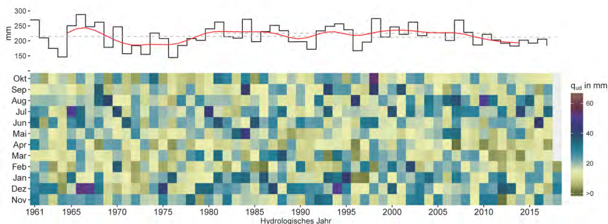
Abb. 31: Zeitreihendarstellung des urbanen Direktabflusses in NRW. Erläuterung der Darstellungsweise im Text am Kapitelanfang
