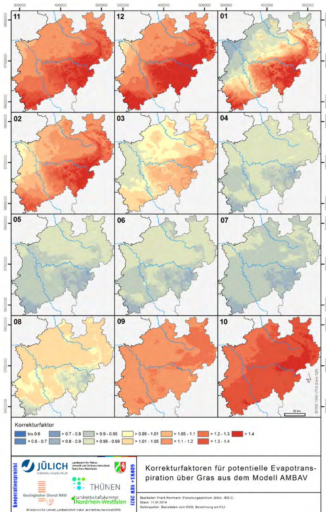
Abb. 6: Monatliche Korrekturfaktoren für potentielle Evapotranspiration über Gras aus dem Modell AMBAV
