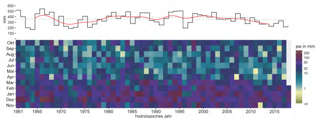
Abb. 32: Zeitreihendarstellung der Sickerwasserbildung aus der durchwurzelten Bodenzone in NRW. Erläuterung der Darstellungsweise im Text am Kapitelanfang
