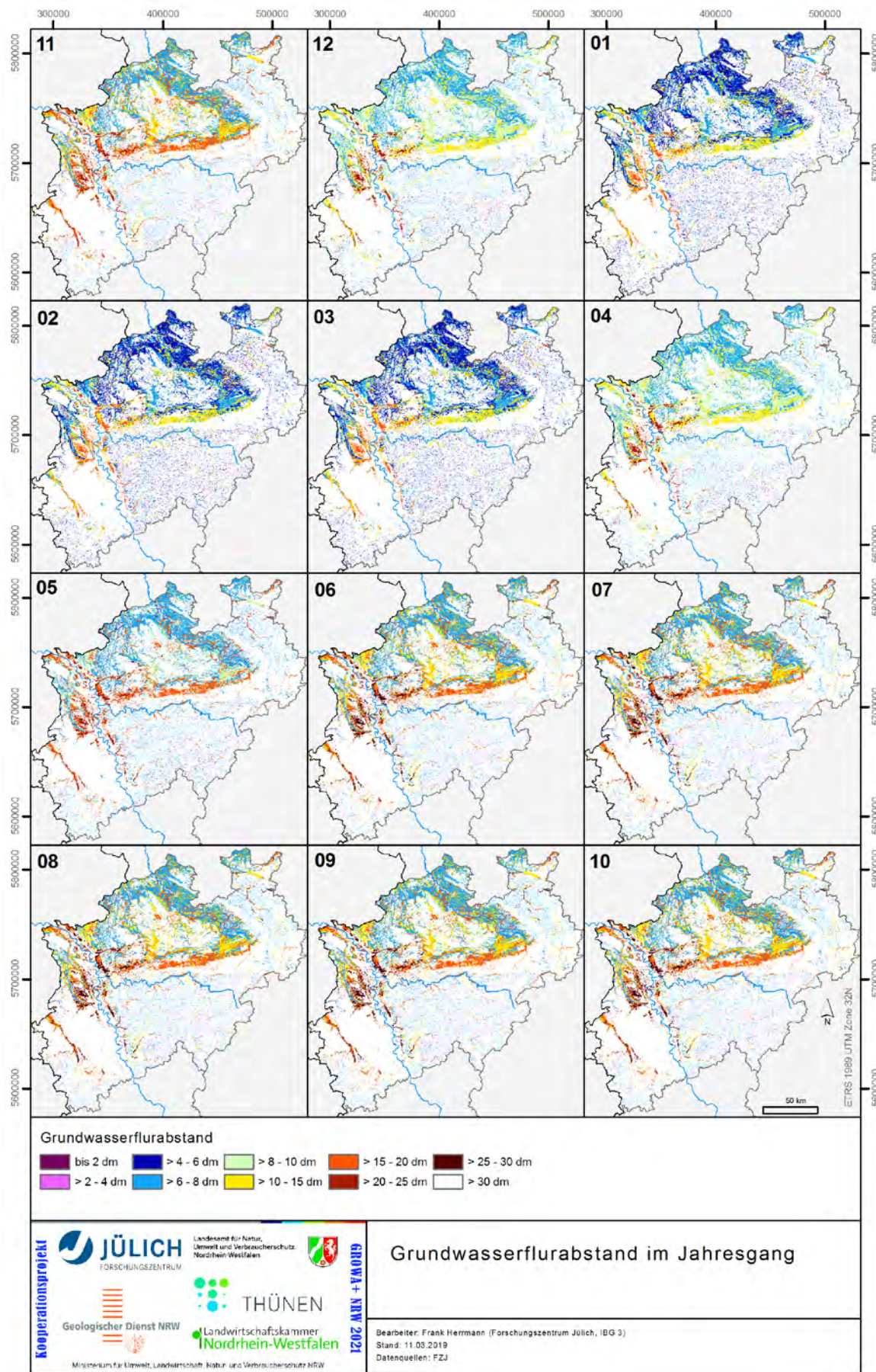
Abb. 27: Grundwasserflurabstand im Jahresgang (Monate nummeriert)
