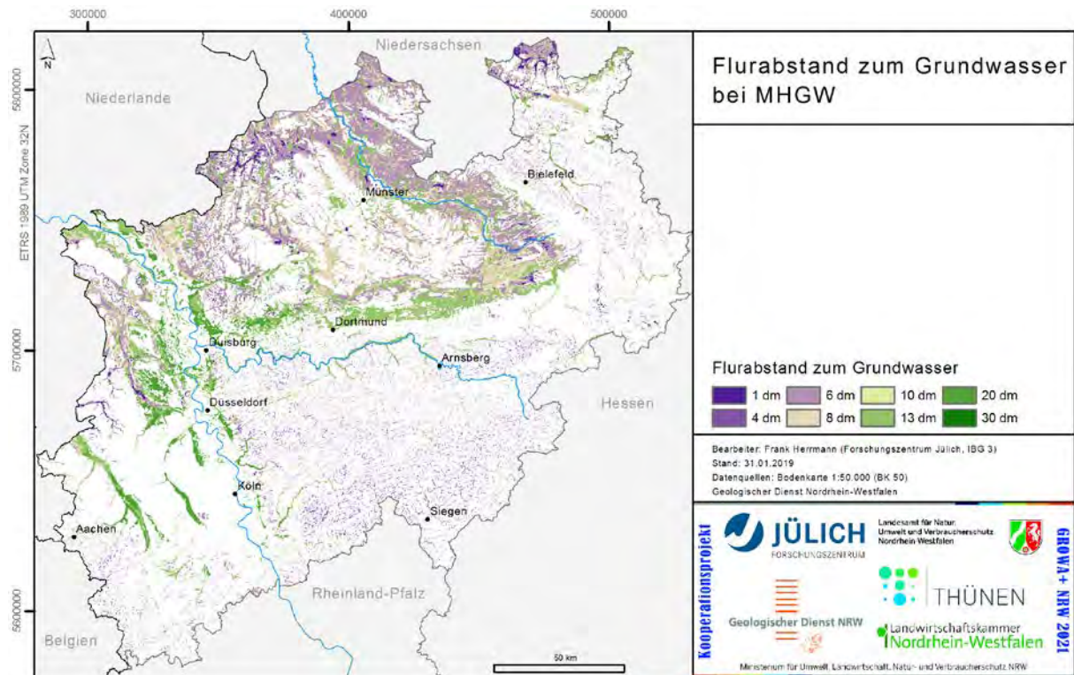
Abb. 22: Flurabstand des Grundwassers bei MHGW aus BK 50 (der Flurabstand der Grundwasserstufe ‚mittel‘ wurde bei MHGW auf 60 cm gesetzt)
