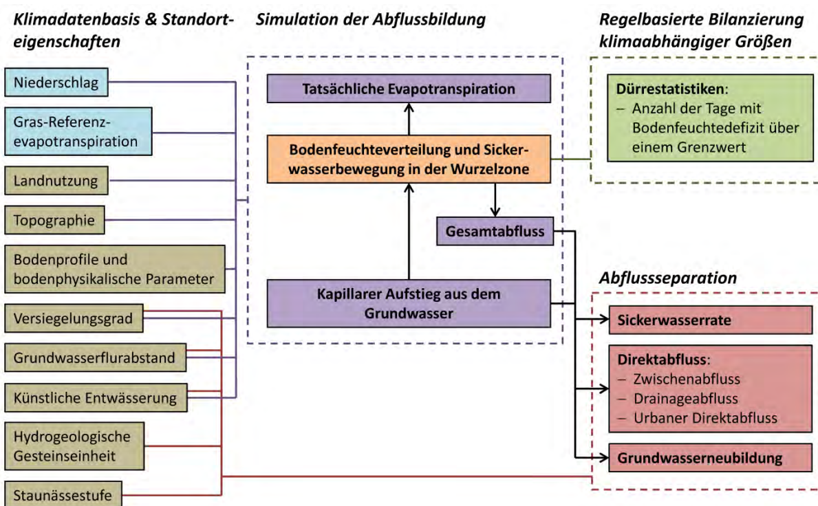
Abb. 1: Modellkonzept des Wasserhaushaltsmodells mGROWA in der Implementierung für Nordrhein-Westfalen.
