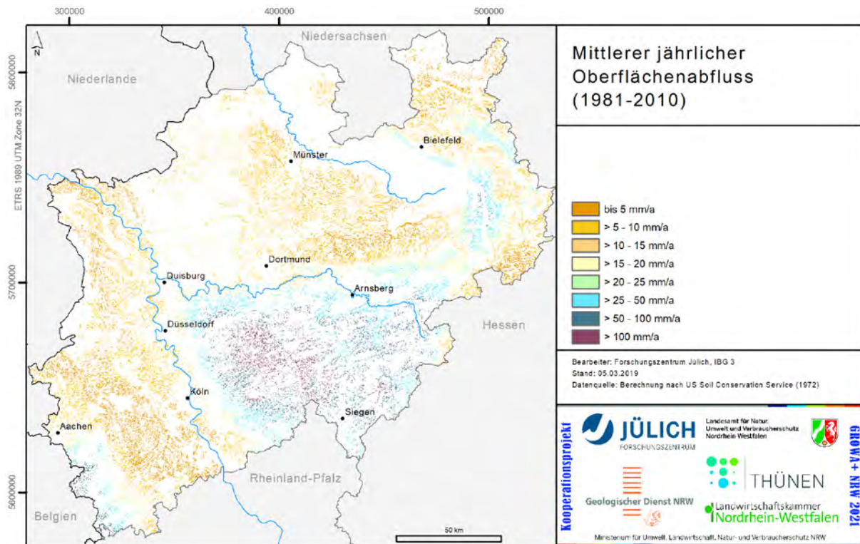
Abb. 45: Mittlerer jährlicher Oberflächenabfluss (1981-2010) auf den für die Nährstoffmodellierung relevanten Flächen mit Gewässeranbindung; berechnet nach US Soil Conservation Service (1972)
