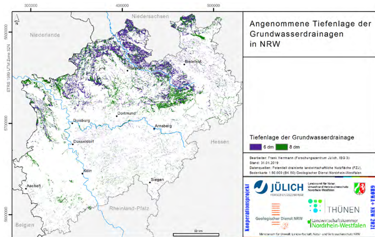
Abb. 24: Angenommene Tiefenlage der Grundwasserdrainagen in NRW
