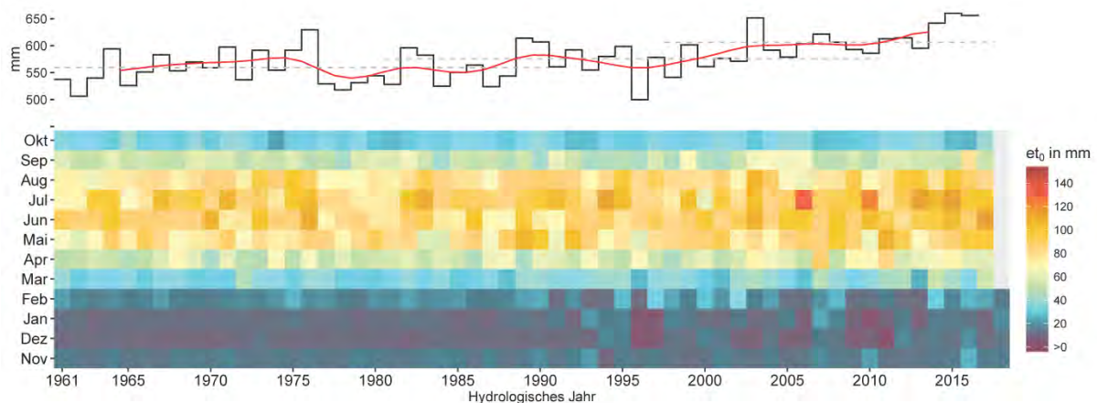
Abb. 28: Zeitreihendarstellung der potentiellen Evapotranspiration über Gras in NRW. Erläuterung der Darstellungsweise im Text am Kapitelanfang
