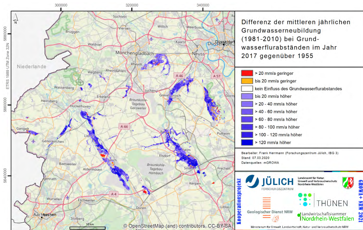
Abb. 46: Differenz der mittleren jährlichen Grundwasserneubildung (1981-2010) bei Grundwasserflurabständen im Jahr 2017 gegenüber 1955
