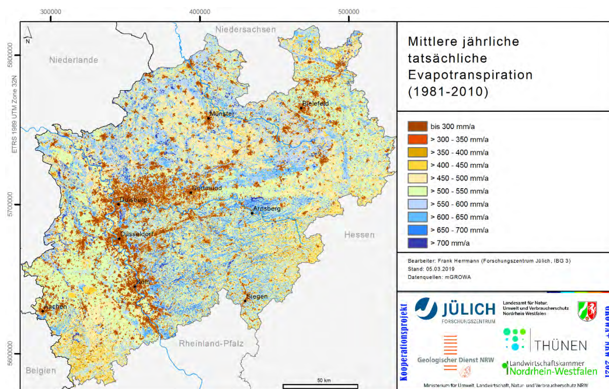
Abb. 36: Mittlere jährliche tatsächliche Evapotranspiration (1981-2010)
