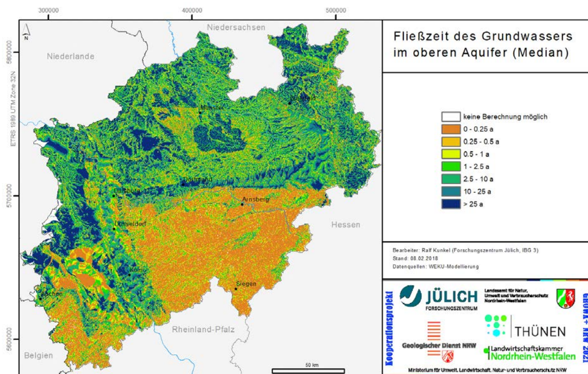
Abb. 7-2: Fließzeit des Grundwassers im oberen Aquifer
