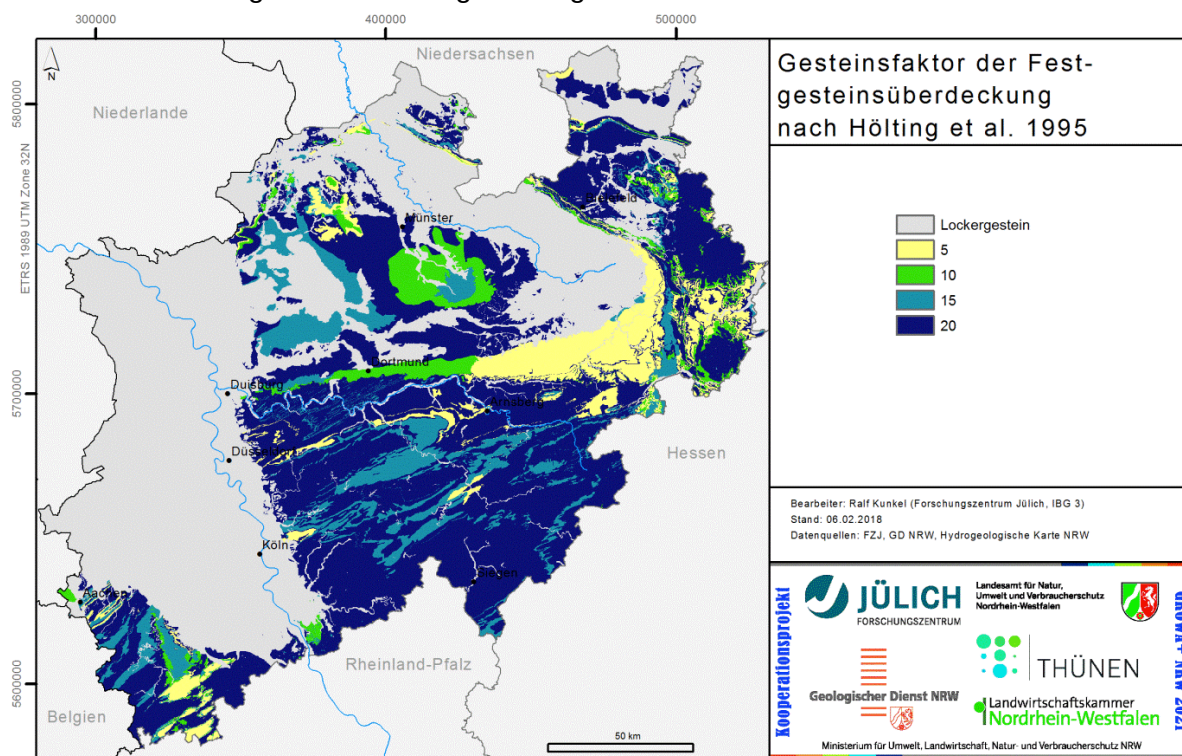
Abb. 5-13: Hölting - Punktwert für die Gesteinsart
