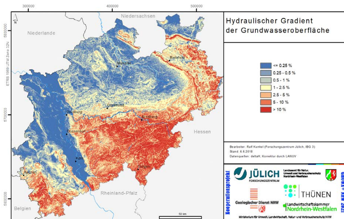
Abb. 5-7: Hydraulischer Gradient der Grundwasseroberfläche
