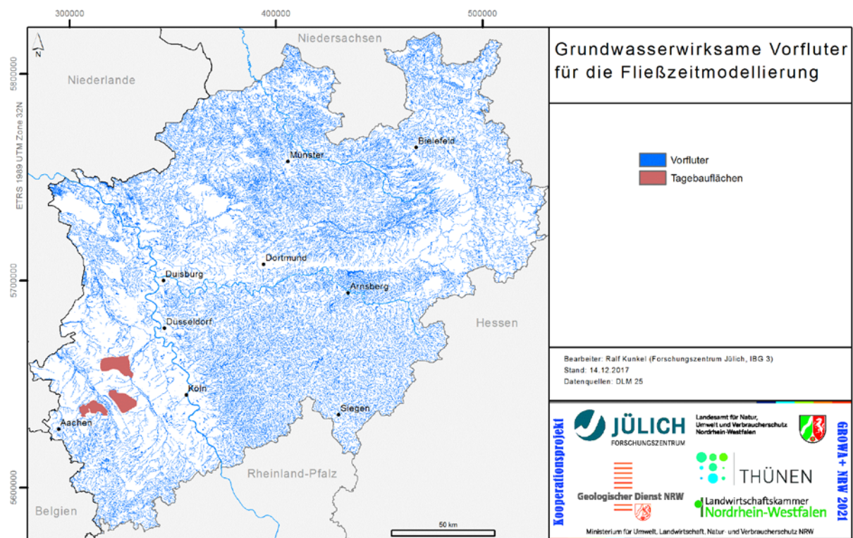
Abb. 5-9: Grundwasserwirksame Vorfluter
