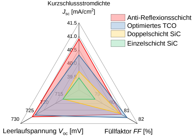
Abbildung 0.2.: Entwicklung der Solarzellenparameter J_{sc} , V_{oc} und FF bei Einsatz einer Einzelschicht \mu\text{c-SiC:H}(n) ( \eta = 22.3\% ), einer Doppelschicht \mu\text{c-SiC:H}(n) ( \eta = 22.9\% ), einer optimierten TCO Deposition ( \eta = 23.8\% ) und einer Anti-Reflexionsbeschichtung ( \eta = 24\% ).
