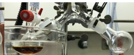
07:22 on 28.02.2019: 3 days checkpoint.
