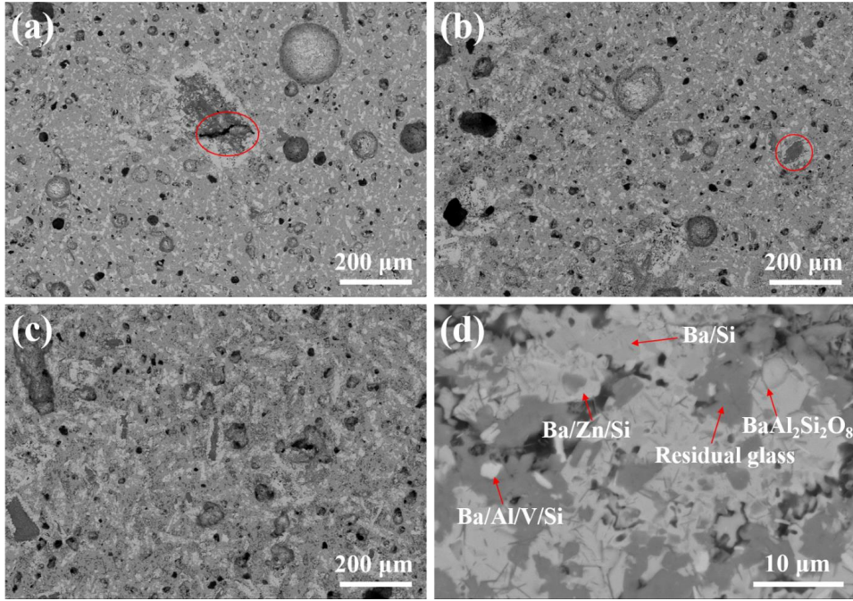
Fig. 4-35. SEM-EDS analyses for annealing composites (a) HBS10A, (b) HBS20A, (c) HBS30A, (d) magnification microstructure of HBS30A
