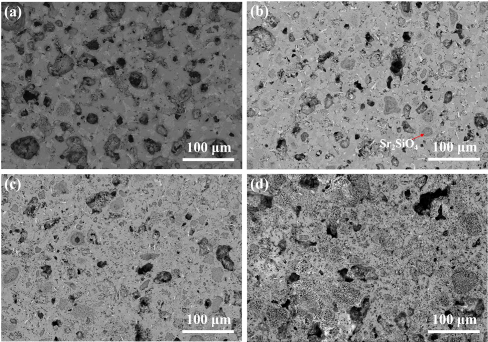
Fig. 4-47. SEM-EDS analyses of annealed composites (a) HS2S10A, (b) HS2S20A, (c) HS2S30A, (d) HS2S40A
